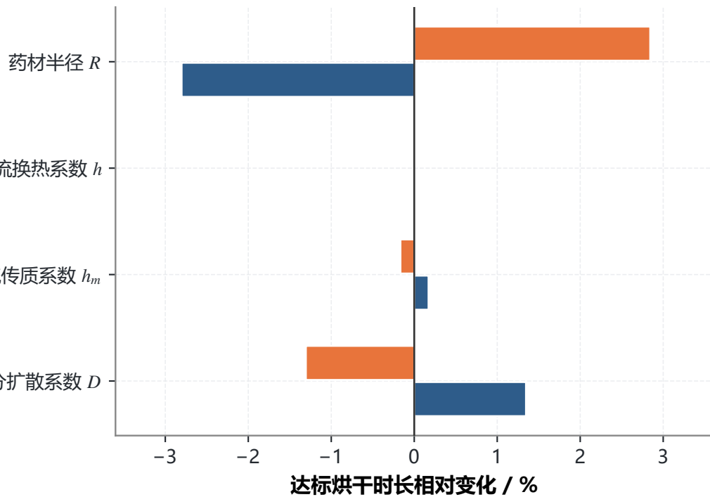
(a) 问题3 敏感性响应
