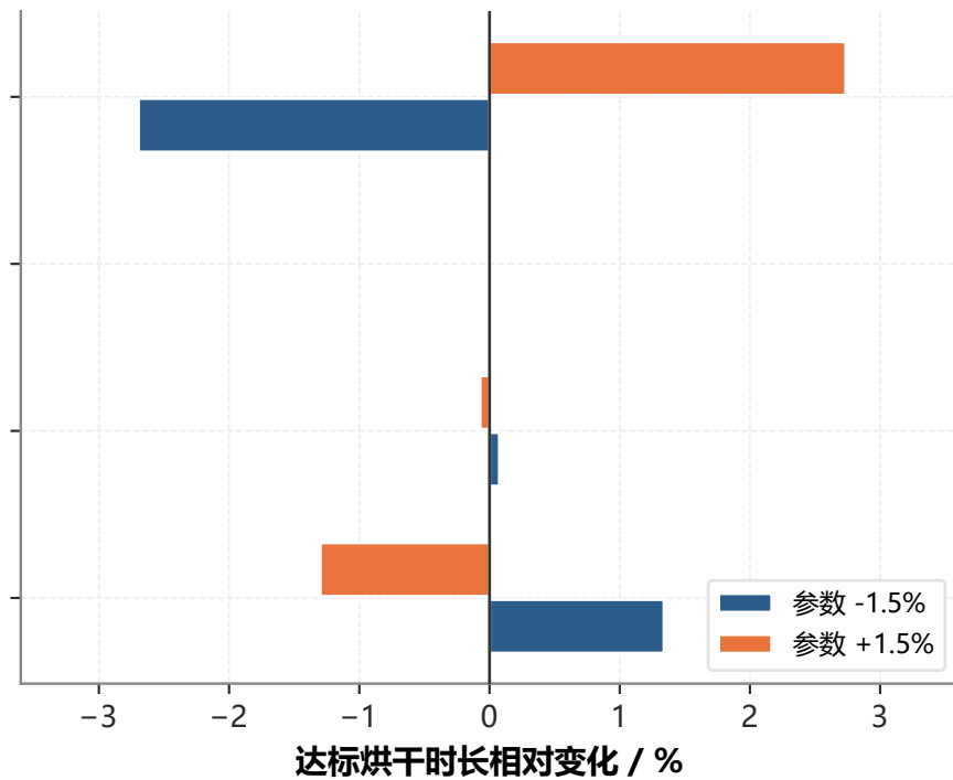
(b) 问题4 敏感性响应
