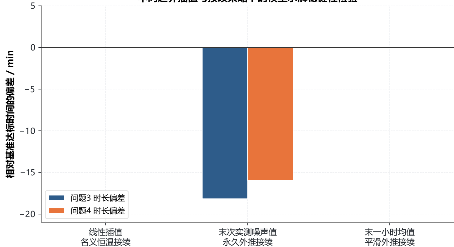
不同边界插值与接续策略下的模型求解稳健性检验
