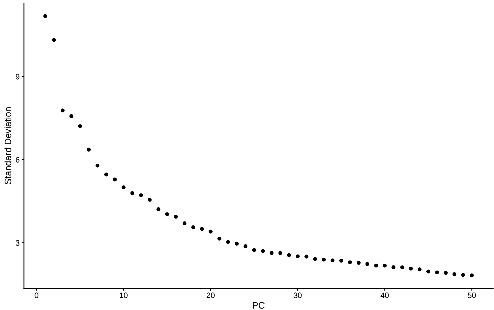
PCA elbow plot
