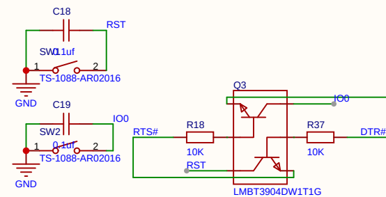
主控芯片-esp32s3-wroom-u2-n16r8以及复位电路
