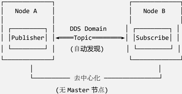
图 1-1 : DDS 去中心化架构
