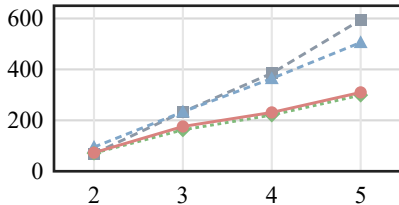
(b) MMLU
