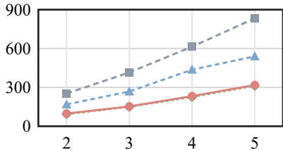
(a) GSM8K
