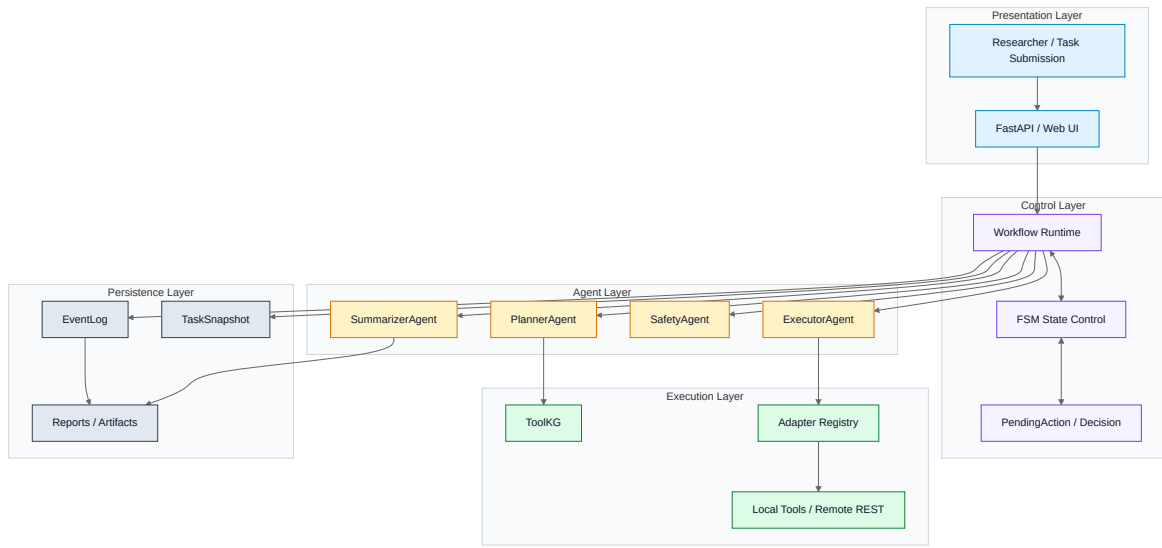
图 3: 系统分层架构概览
