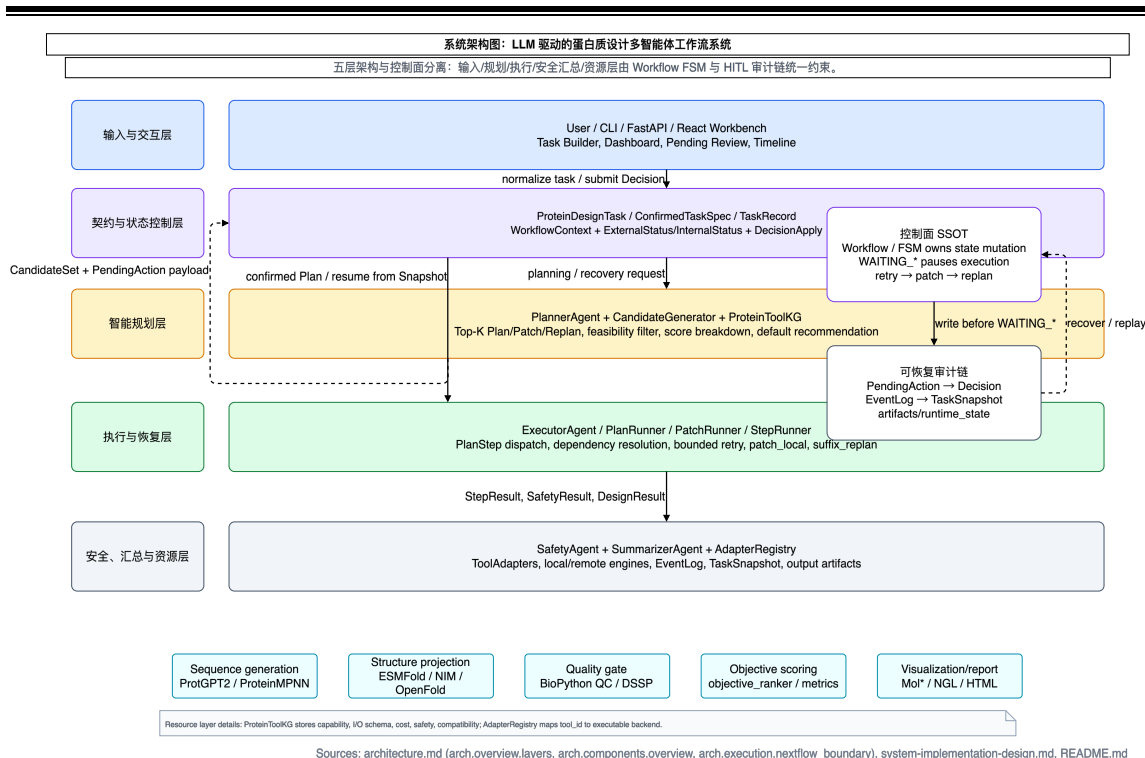
图 4-1 系统五层分层架构
