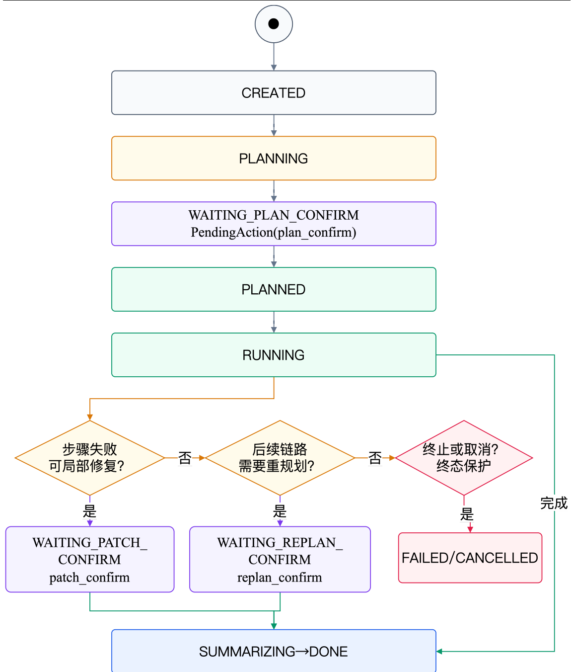
图 4-3 FSM 状态转移图
