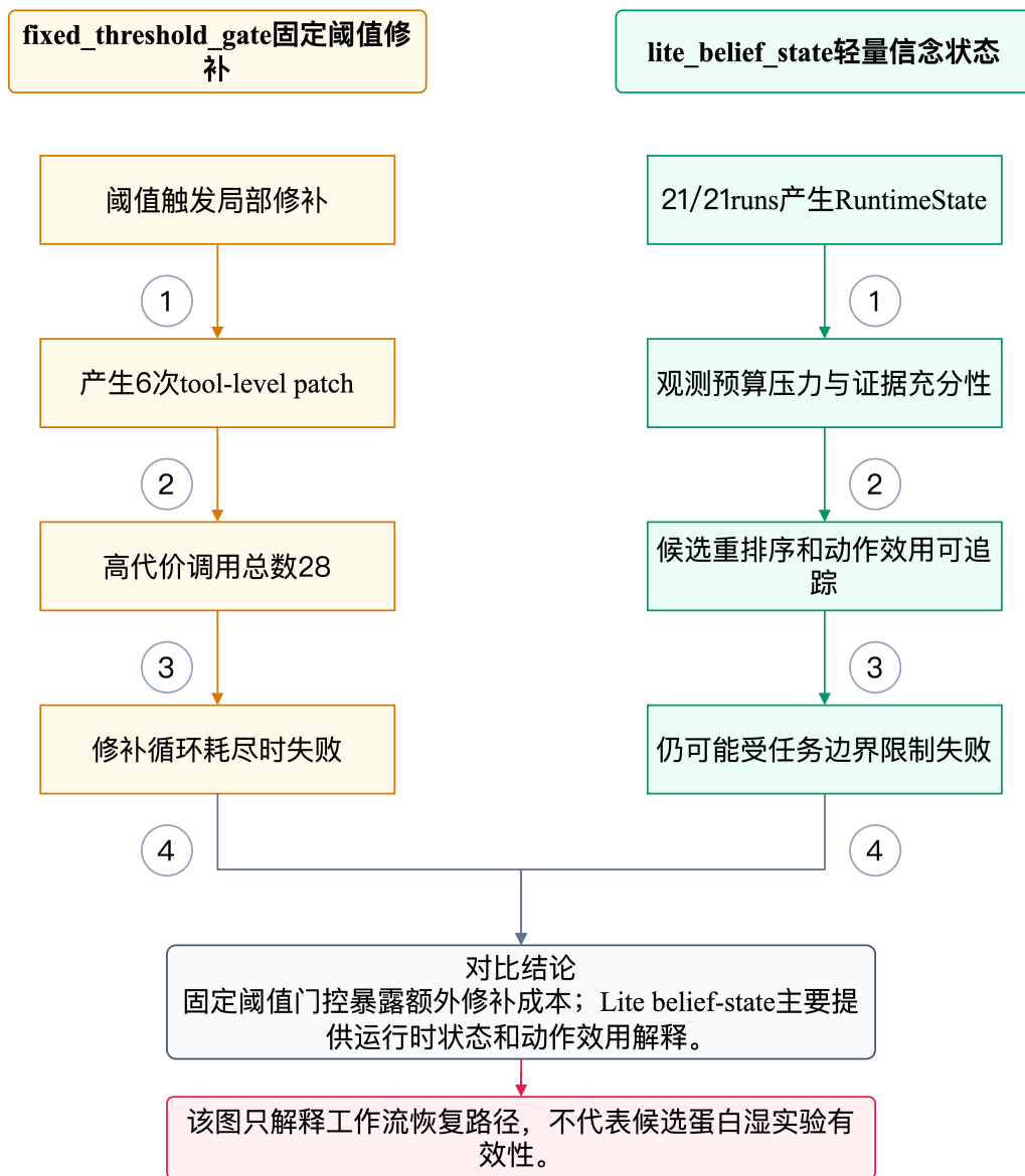
图 6-2 固定修补与 Lite belief-state 重排序的恢复路径对比
