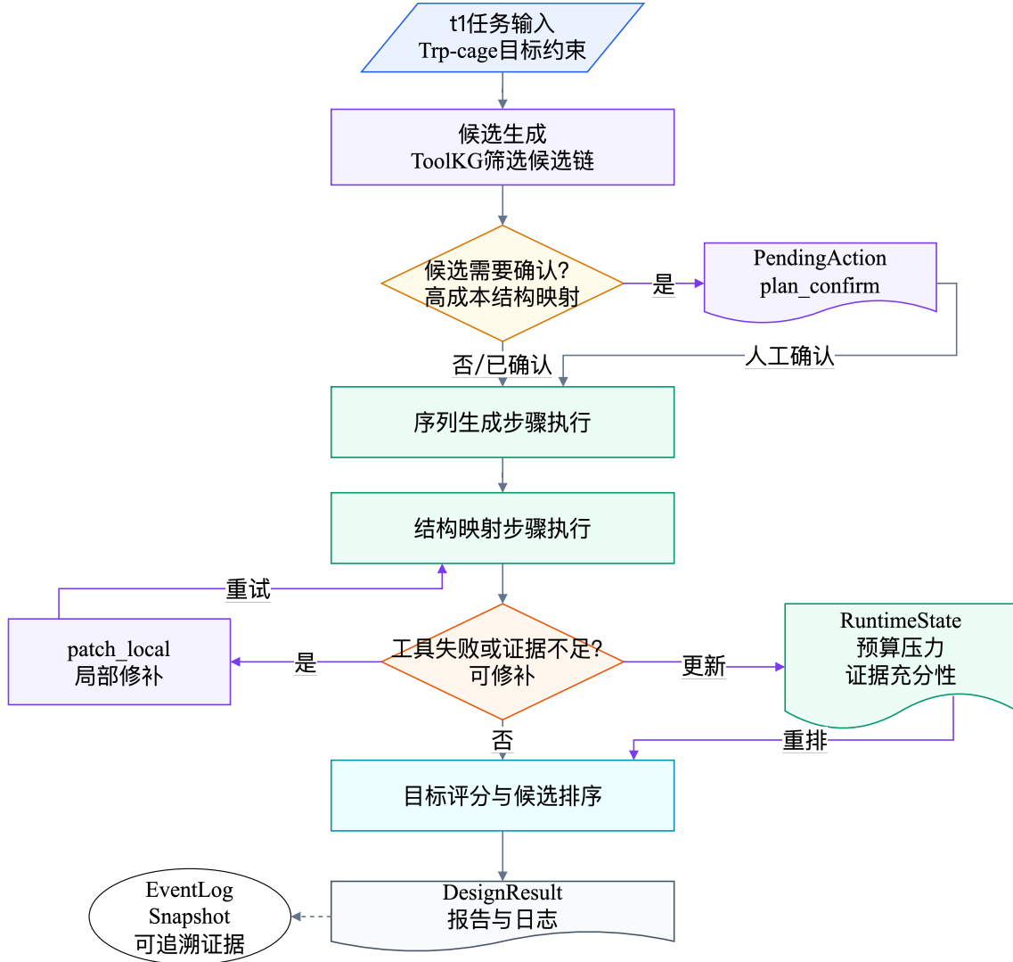
图 4-8 t1 任务实例走查
