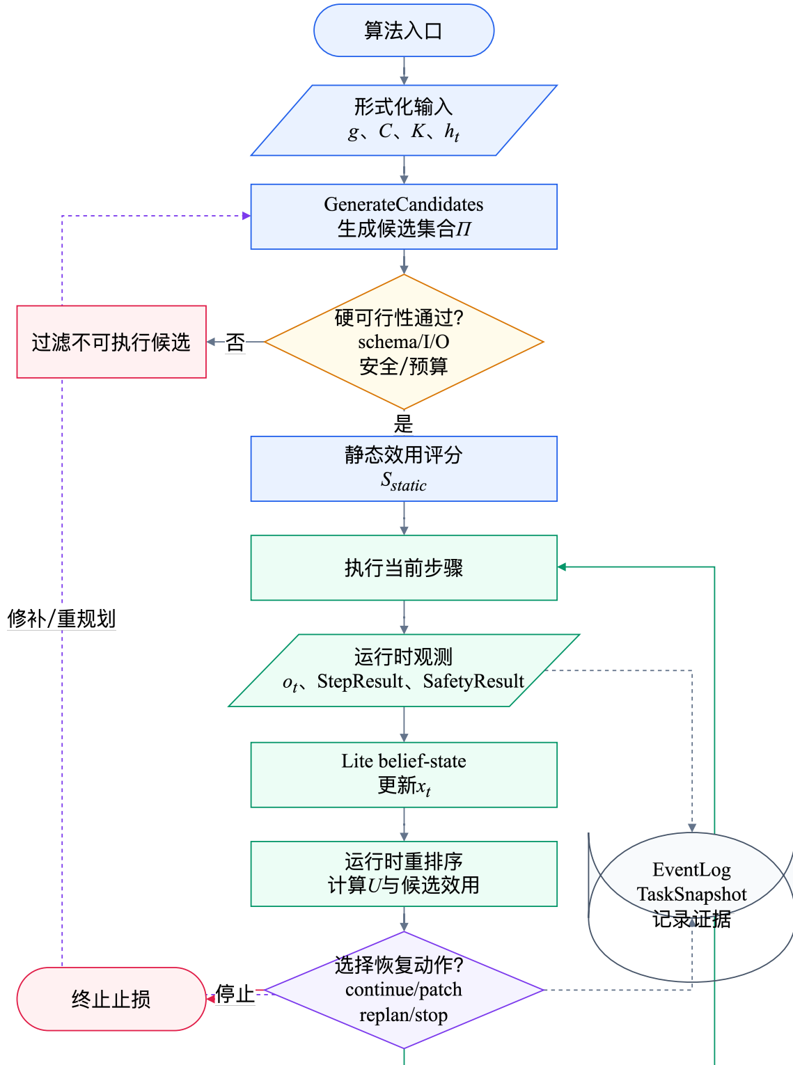
图 4-6 CEBRA-WP 算法闭环
