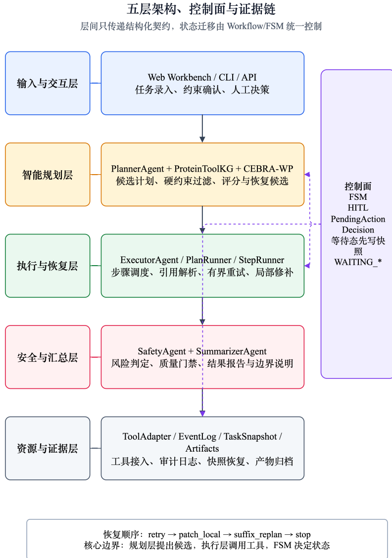
图 4-1 系统五层分层架构
