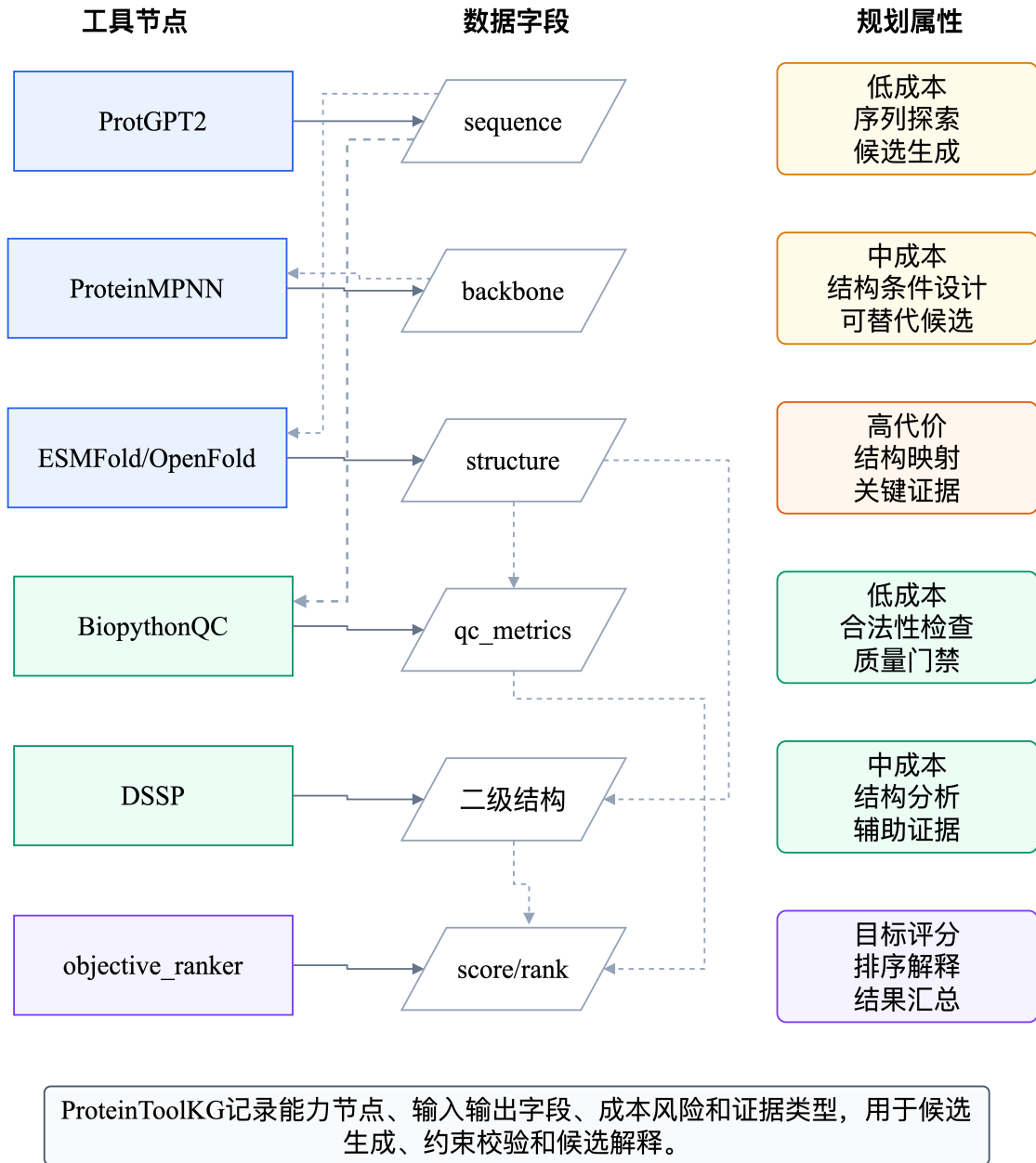
图 4-2 ProteinToolKG 局部可视化
