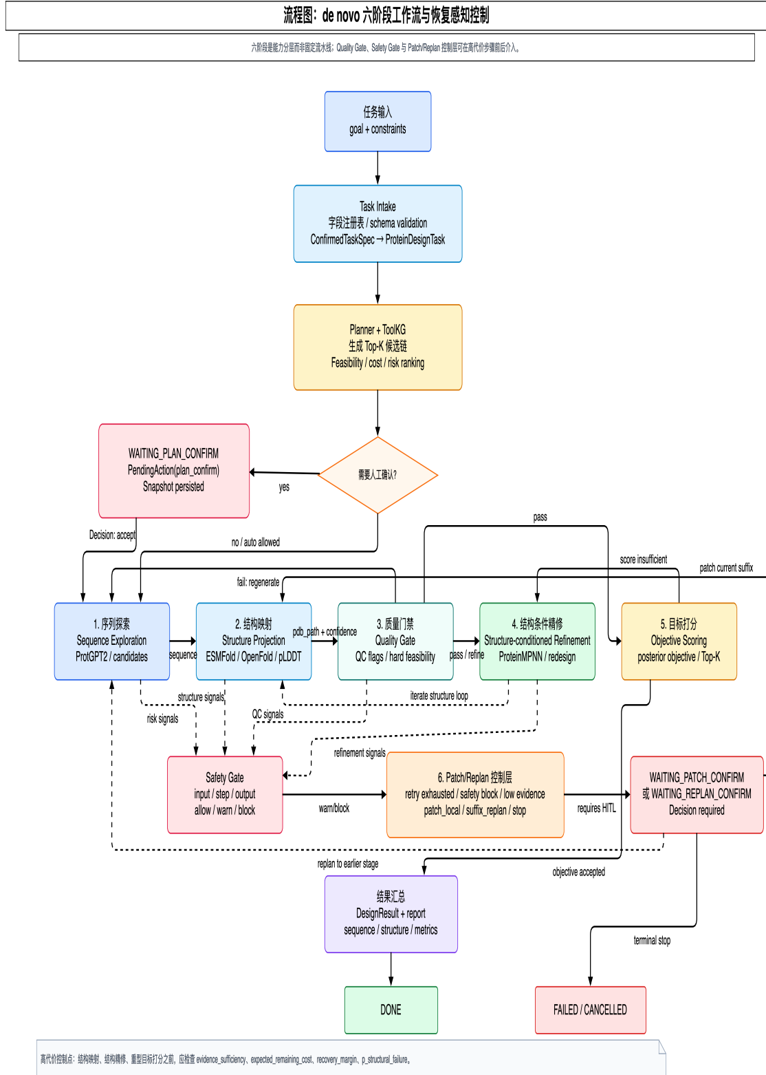
图 4-5 六阶段 de novo 蛋白质设计 workflow
