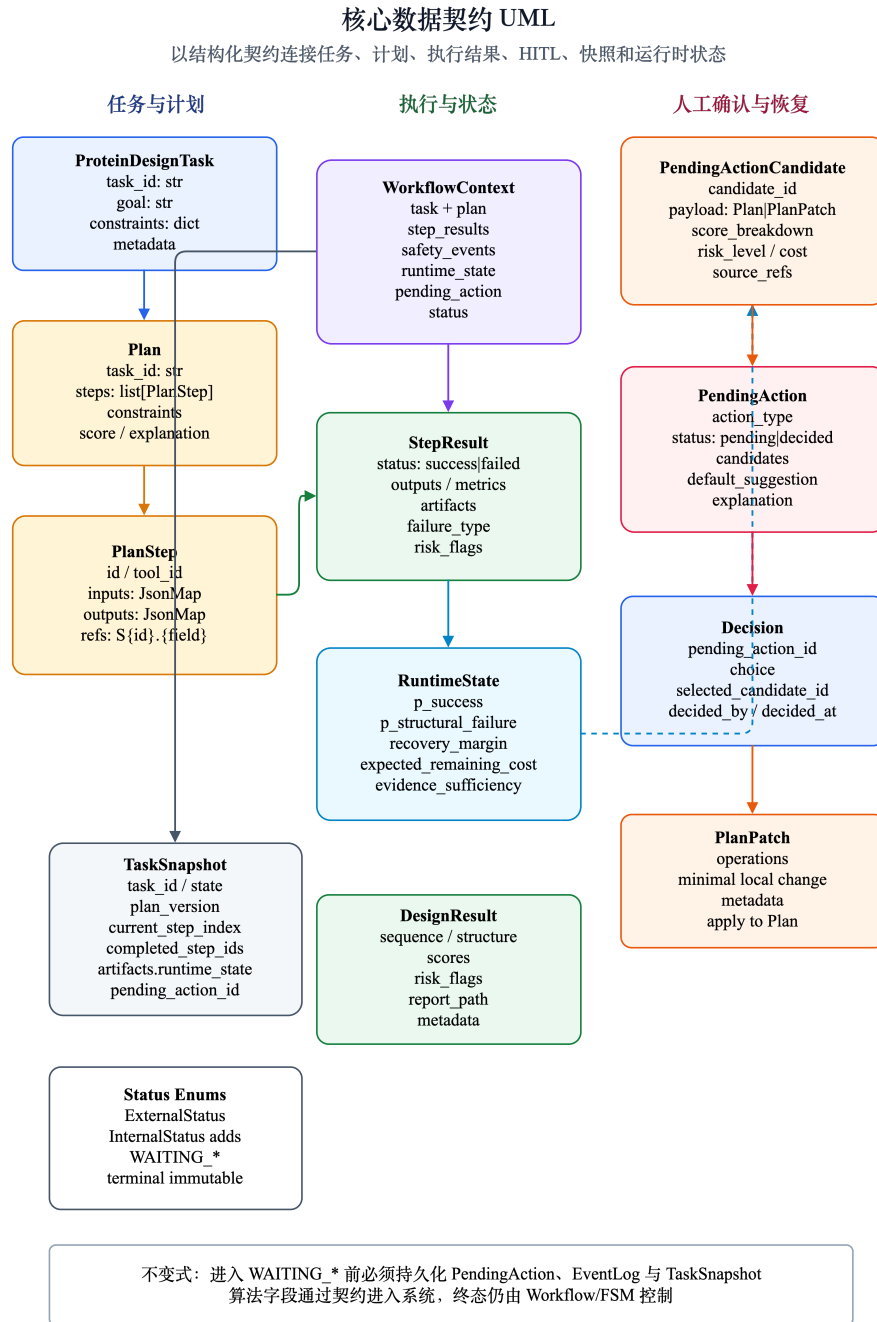
图 4-7 核心数据契约 UML
