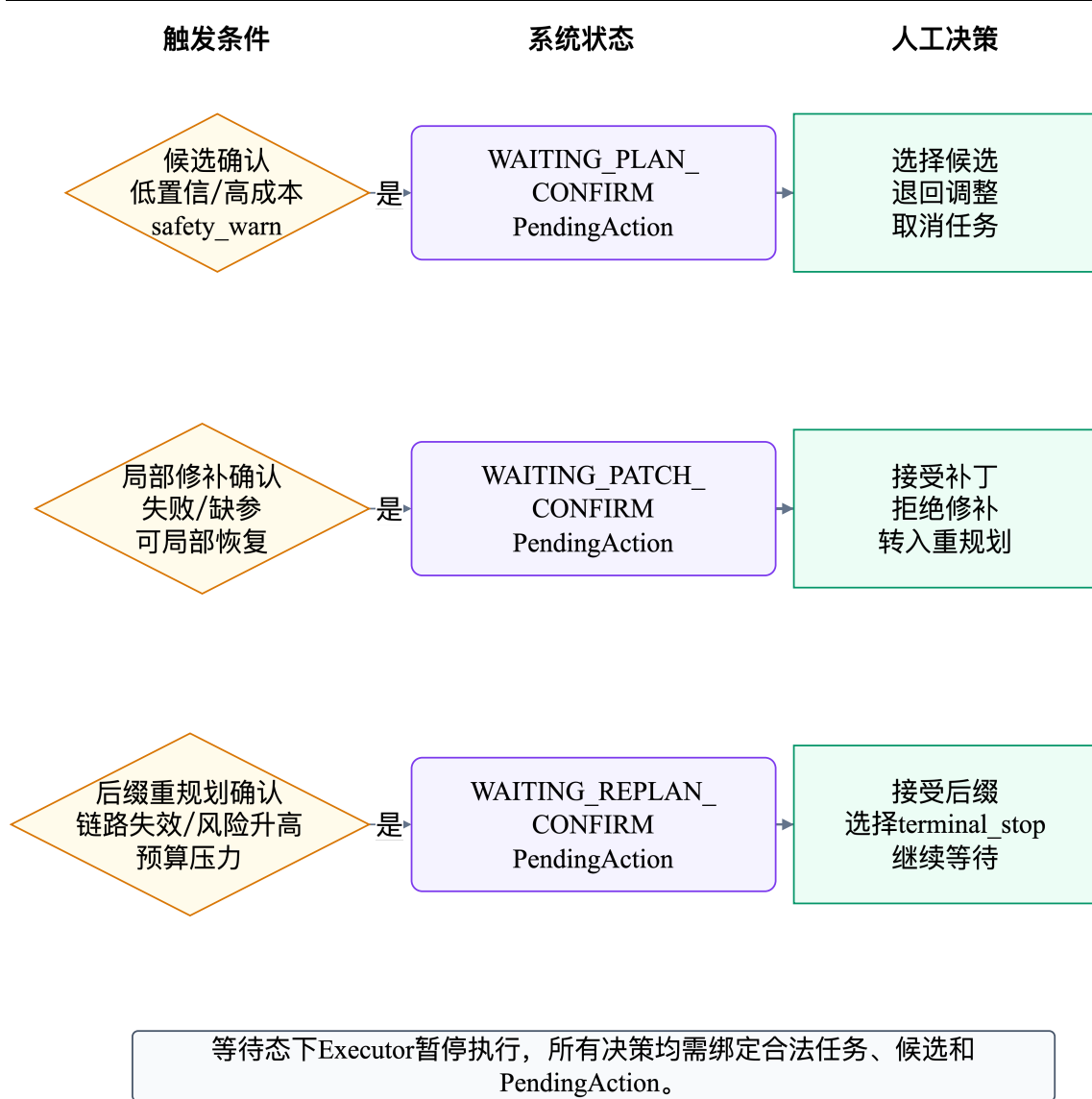
图 4-4 HITL 决策条件
