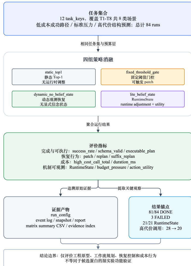
图 6-1 实验设计框架
