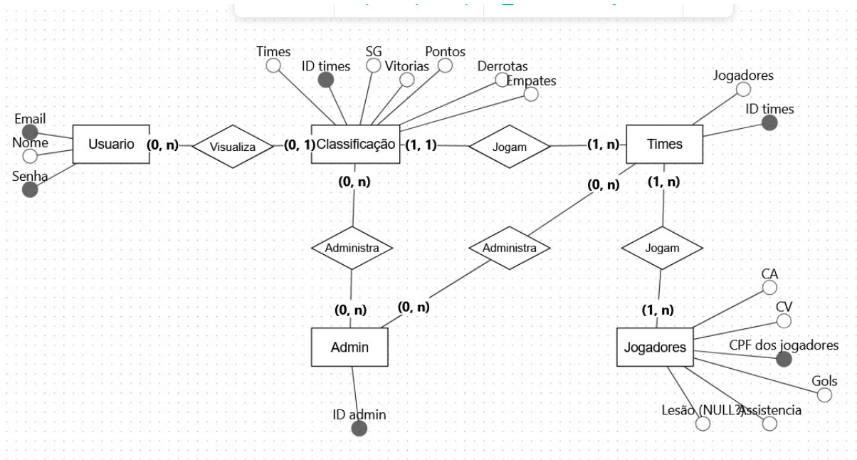
Figura 1: Modelo Conceitual
