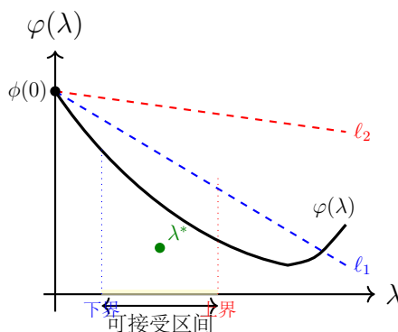
图 4.1: Goldstein 条件的几何解释：可接受步长位于两条直线之间的区域
