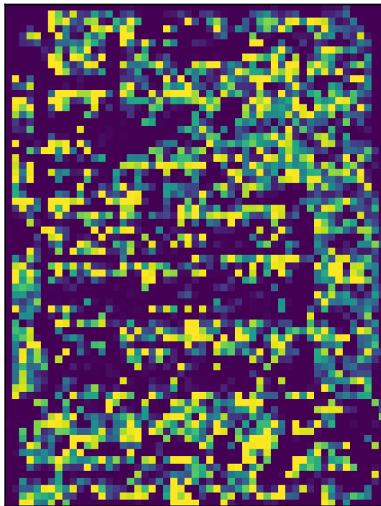
docvqa: 70×53
