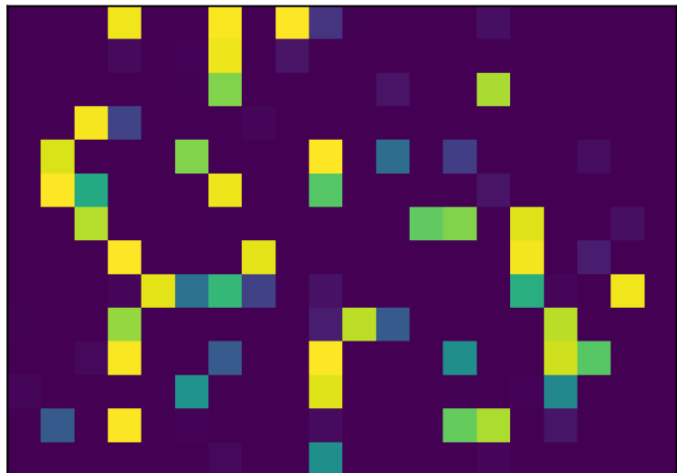
cow: 14×20
