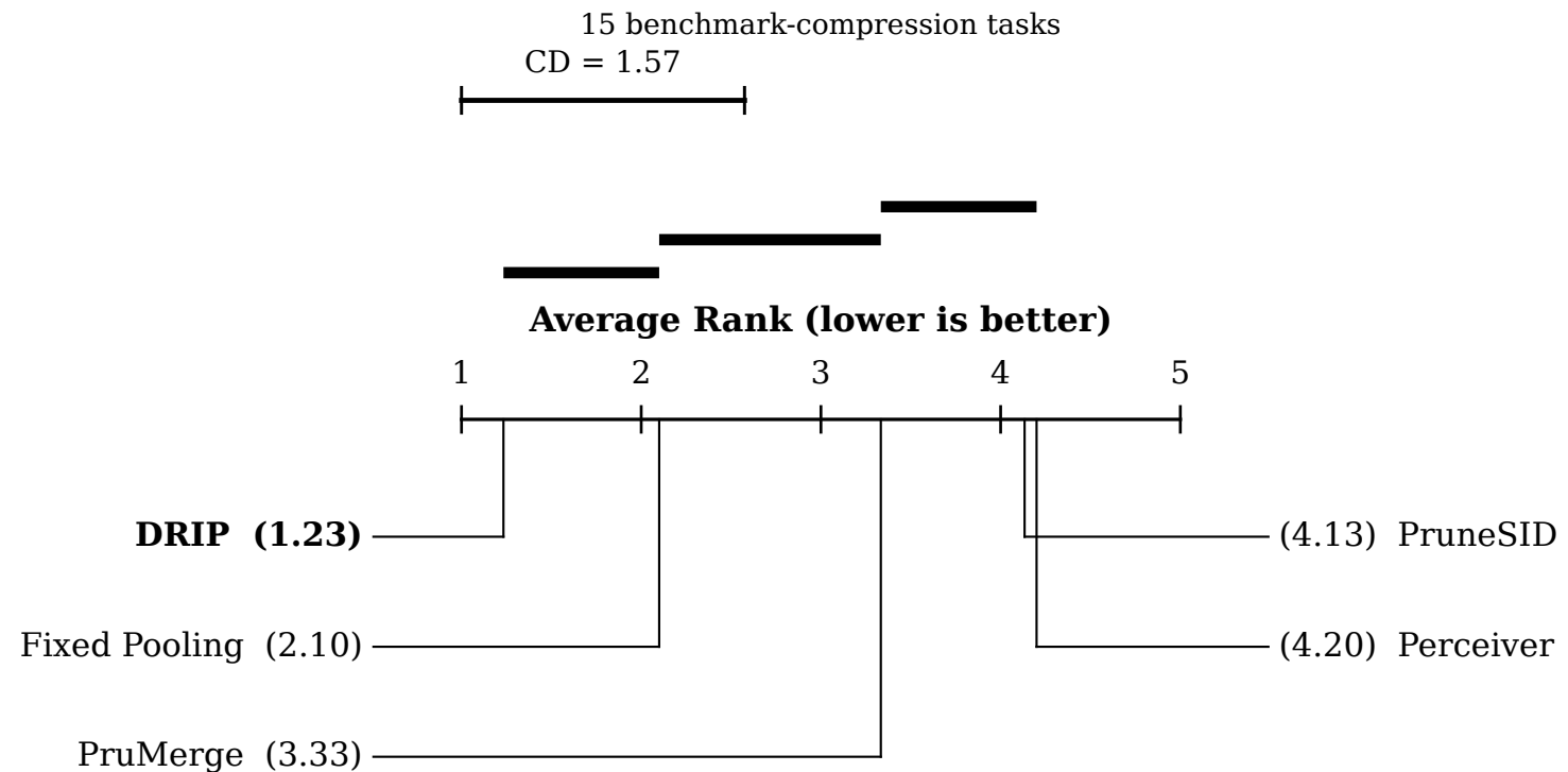
(b) OCR
