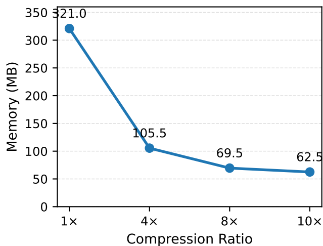
KV Cache
