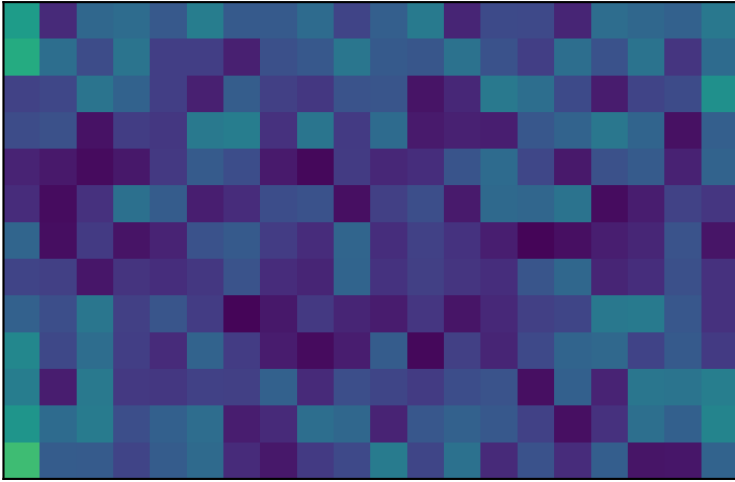
dog: 13×20
