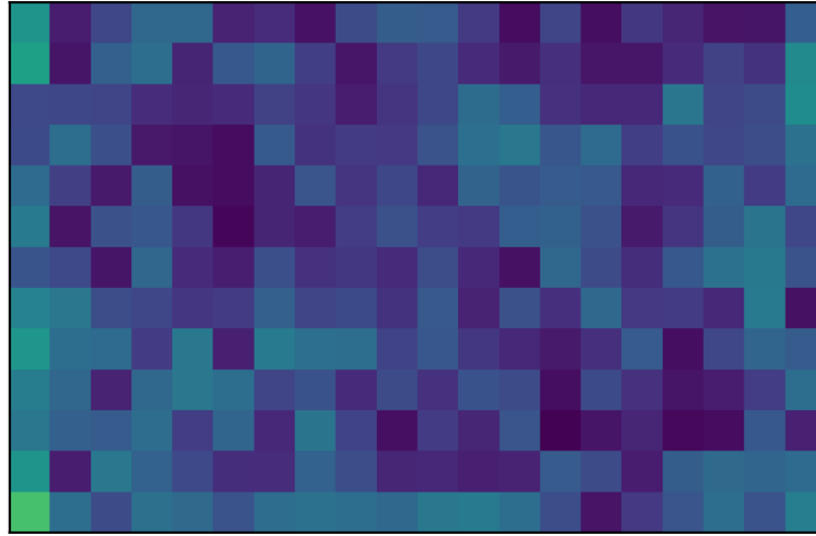
elephant: 13×20
