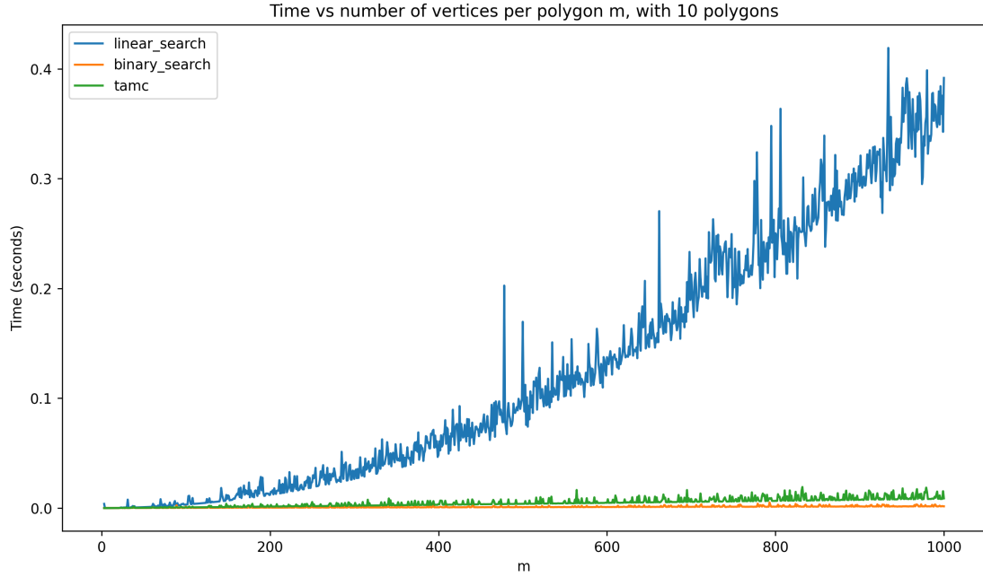
Figura 14: Comparação dos 3 algoritmos conforme m , o número de vértices por polígono, cresce, com k = 10 polígonos.
