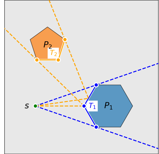
Figura 2: Região de primeiro contato T_1 de P_1 e T_2 de P_2 .
