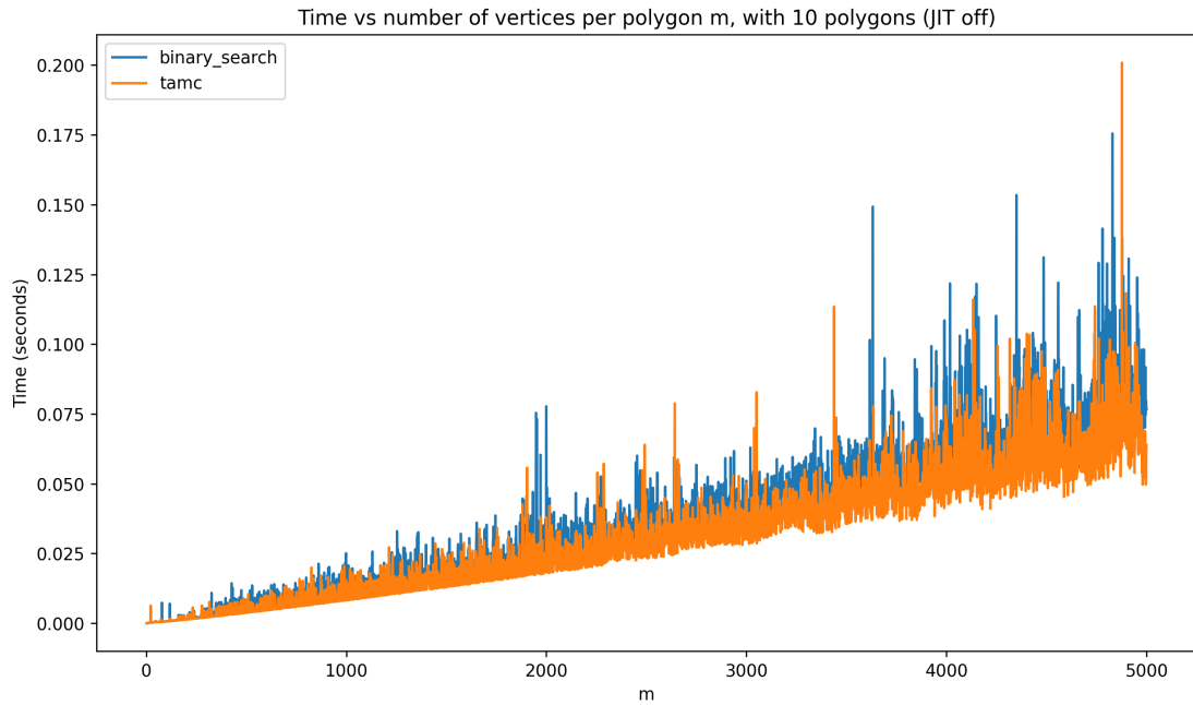
Figura 15: Comparação da busca binária (programação dinâmica) com algoritmo de Tan e Jiang
