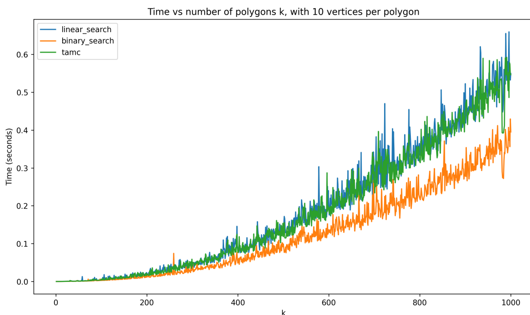
Figura 13: Comparação dos 3 algoritmos conforme k cresce, com 10 vértices por polígono.
