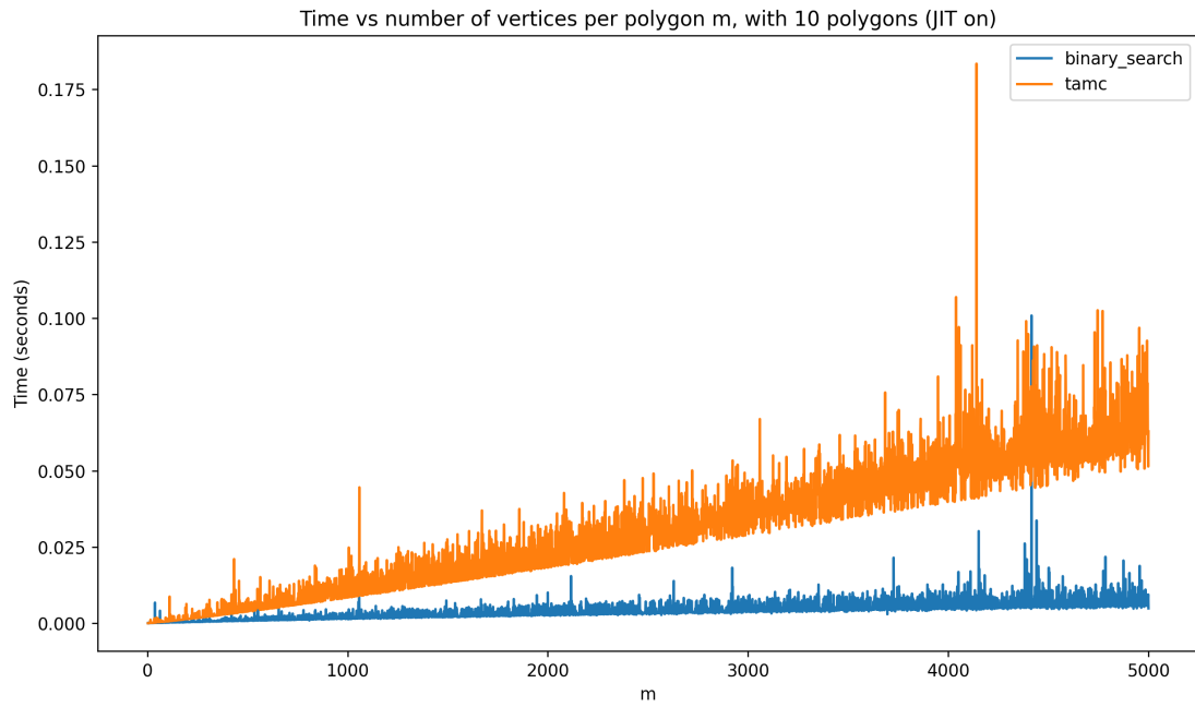
Figura 16: Comparação da busca binária (JIT) com algoritmo de Tan e Jiang, com JIT
