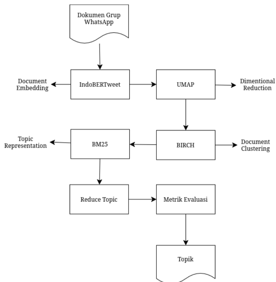
Gambar 3.2: Rancangan framework BERTopic yang dimodifikasi pada tahap pembuatan model
