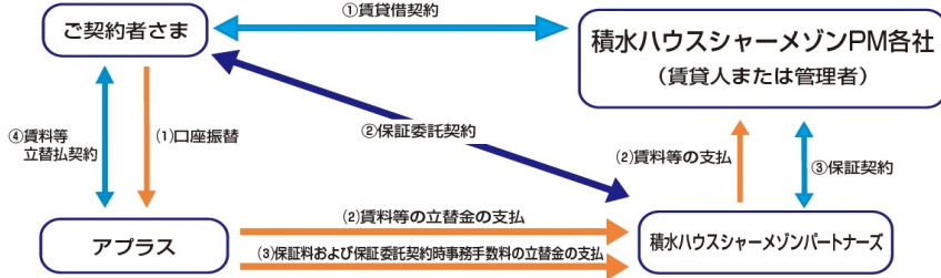
取引形態図
