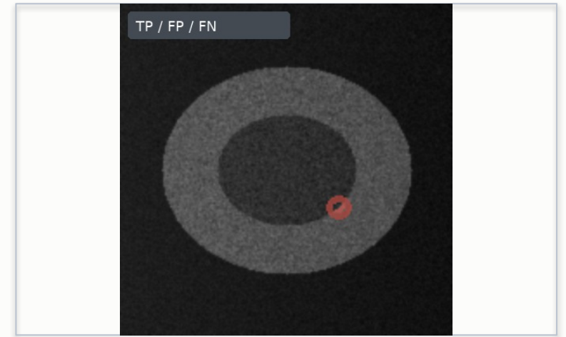
Error map
