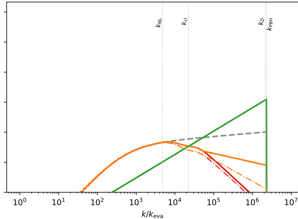
Choptuik: 10^4 g , \beta_f = 10^{-6}
