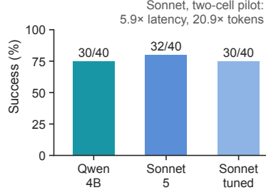
b LIBERO-Plus
