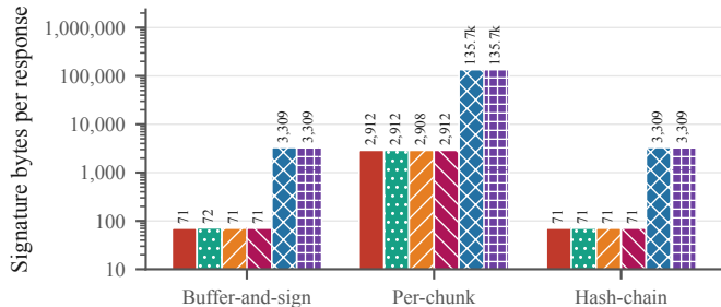
(d) Signature bytes: 200-token response
