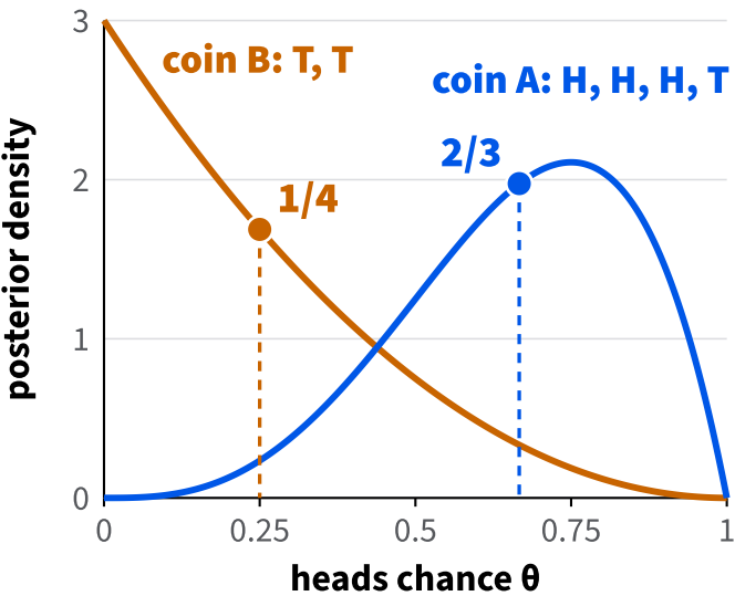
posterior densities, uniform prior: B: 3 \cdot (1 - \theta)^2 , A: 20 \cdot \theta^3 \cdot (1 - \theta)
