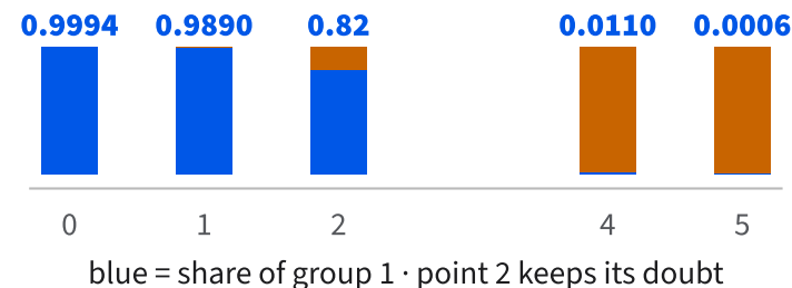
EM ( \sigma = 1 ): soft labels
