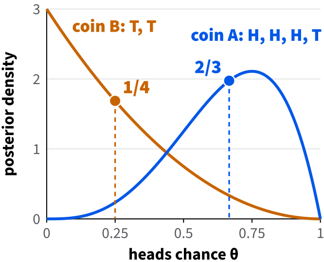
posterior densities, uniform prior: B: 3(1 - \theta)^2 , A: 20\theta^3(1 - \theta)
