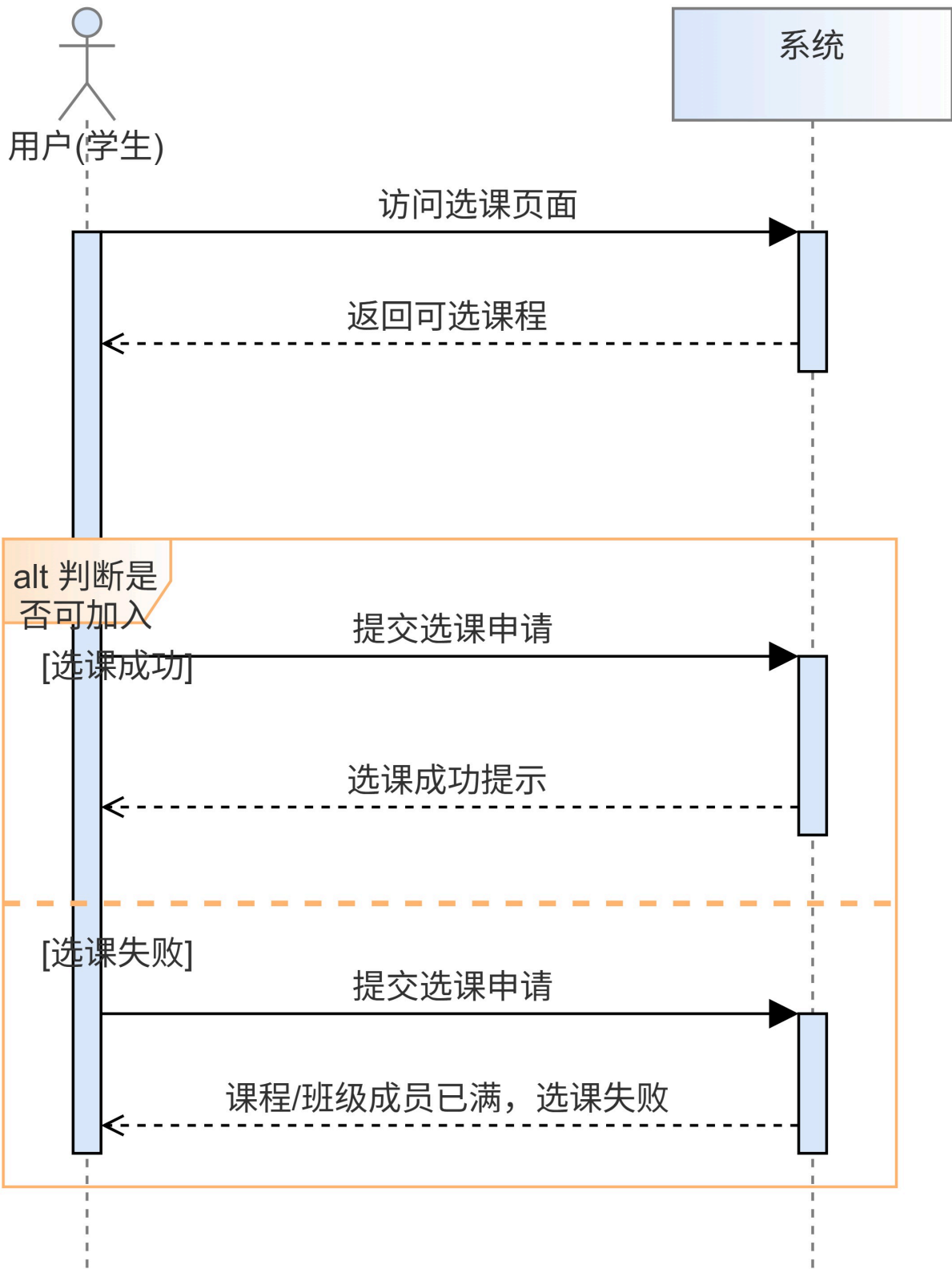
组件级顺序图（概要设计）：
