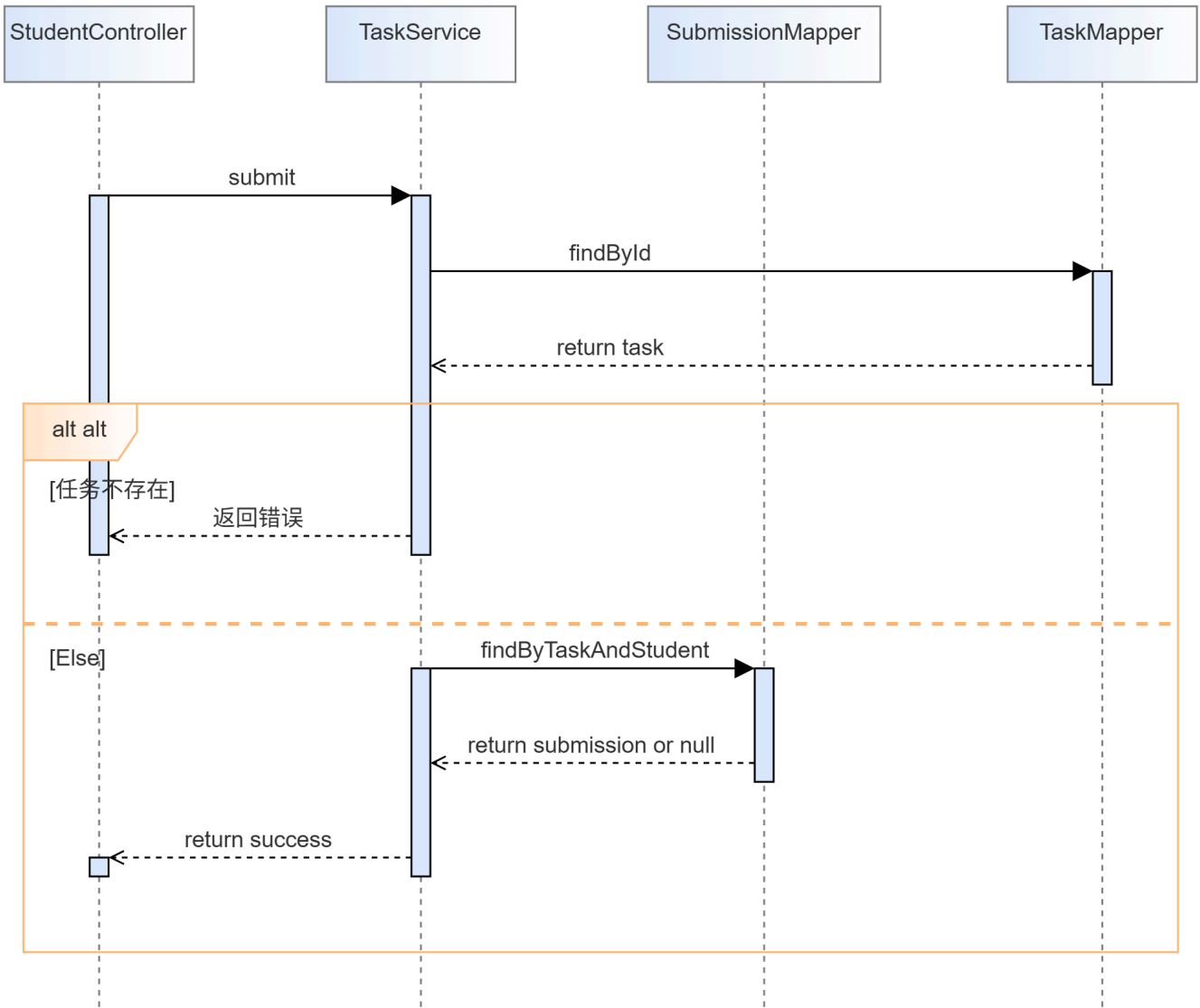
类级顺序图（详细设计）：
