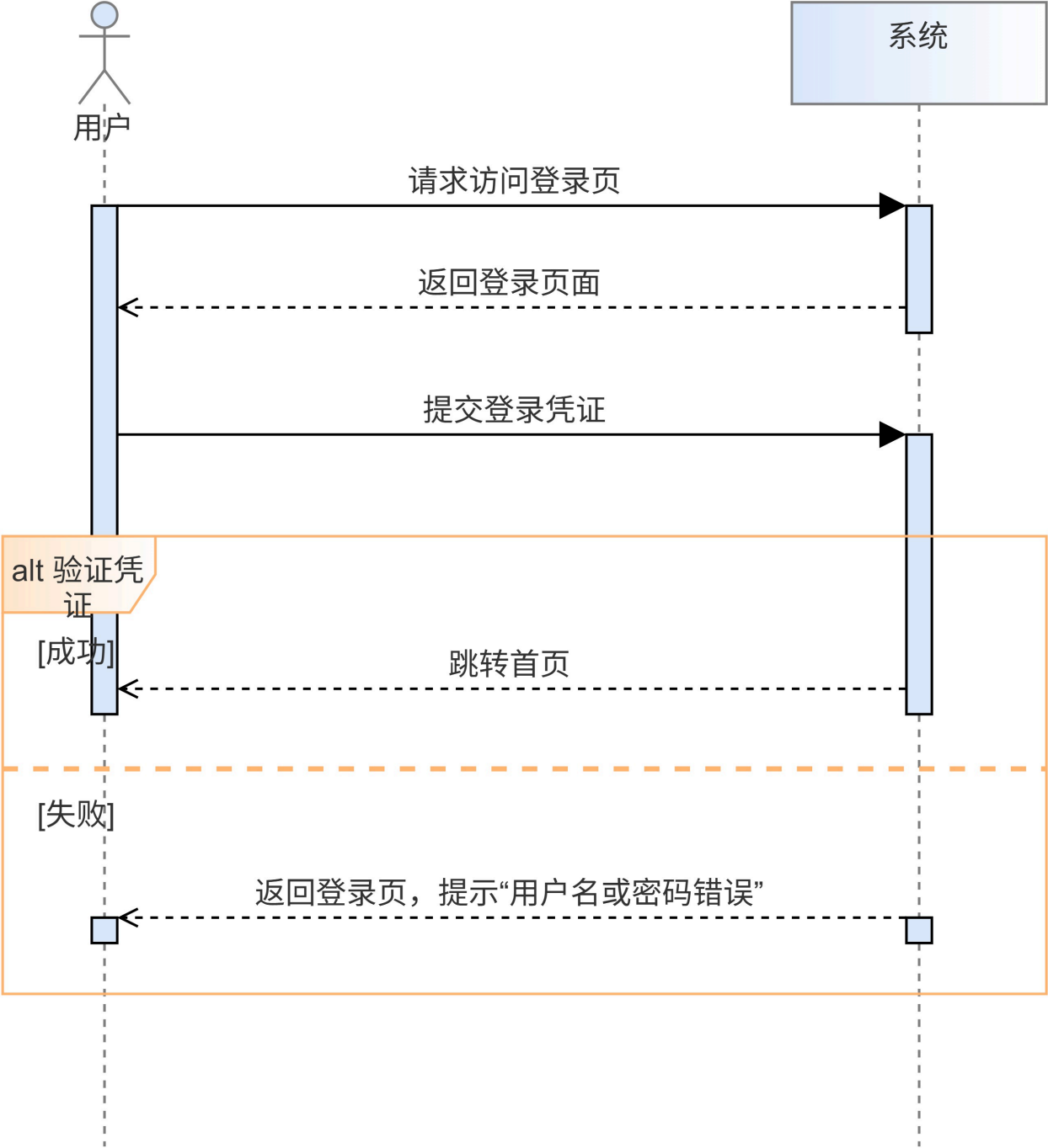
组件级顺序图（概要设计）：
