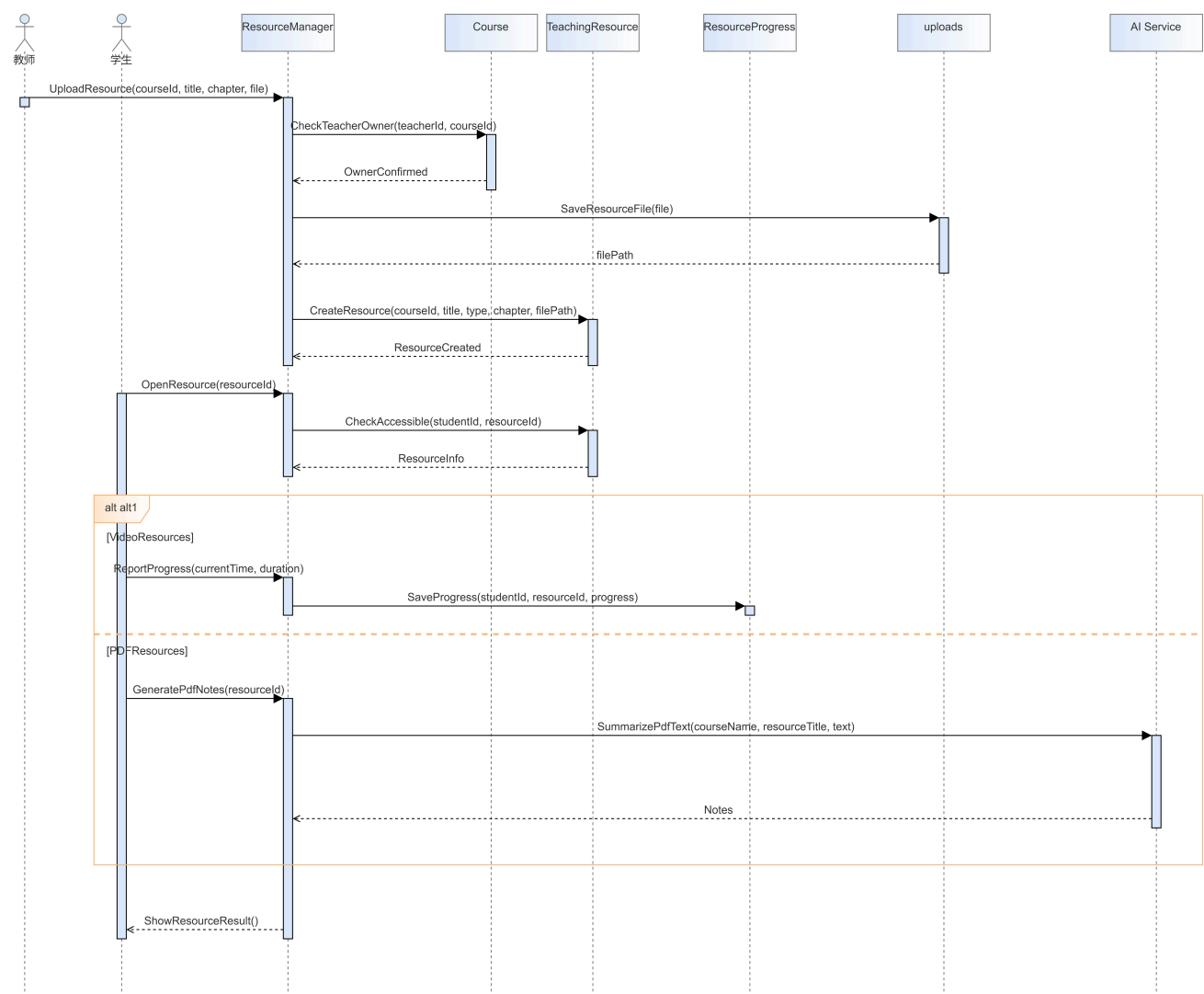
类级顺序图（详细设计）：
