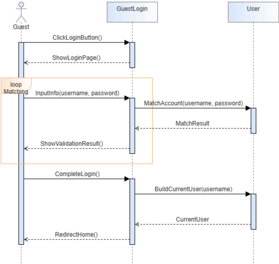
类级顺序图（详细设计）：
