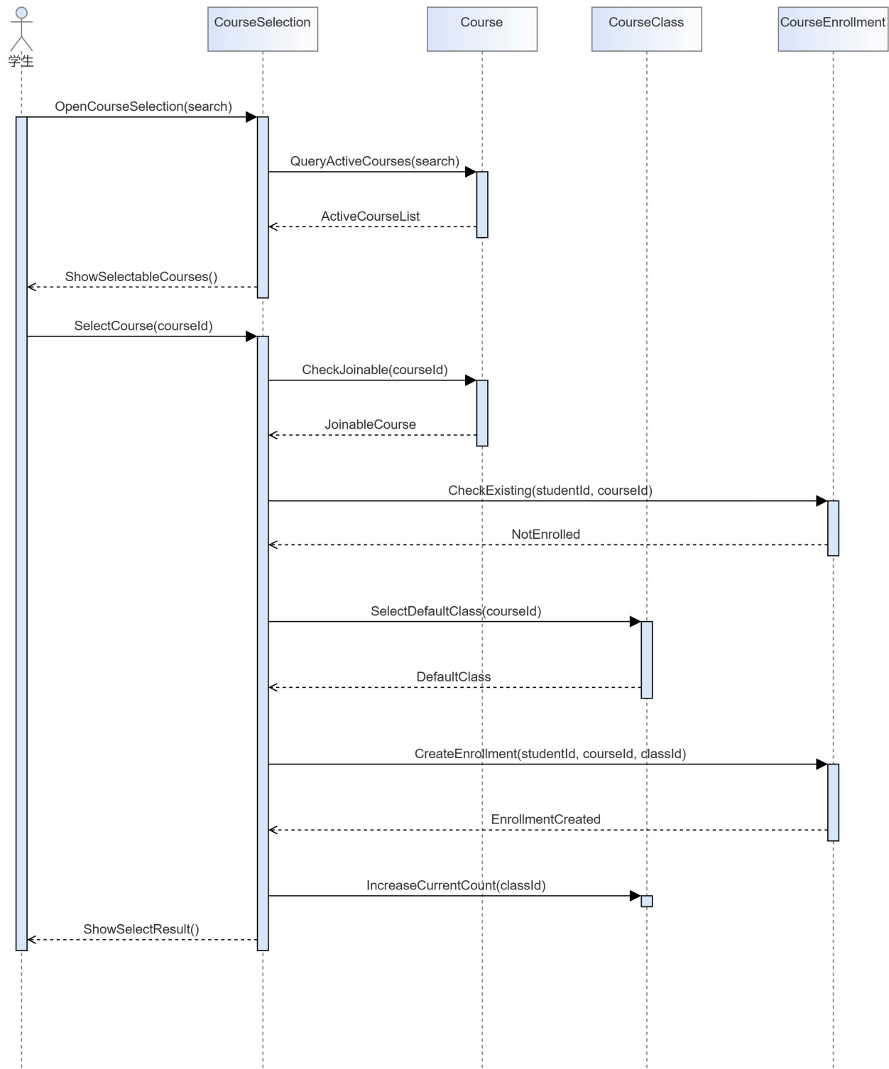
类级顺序图（详细设计）：
