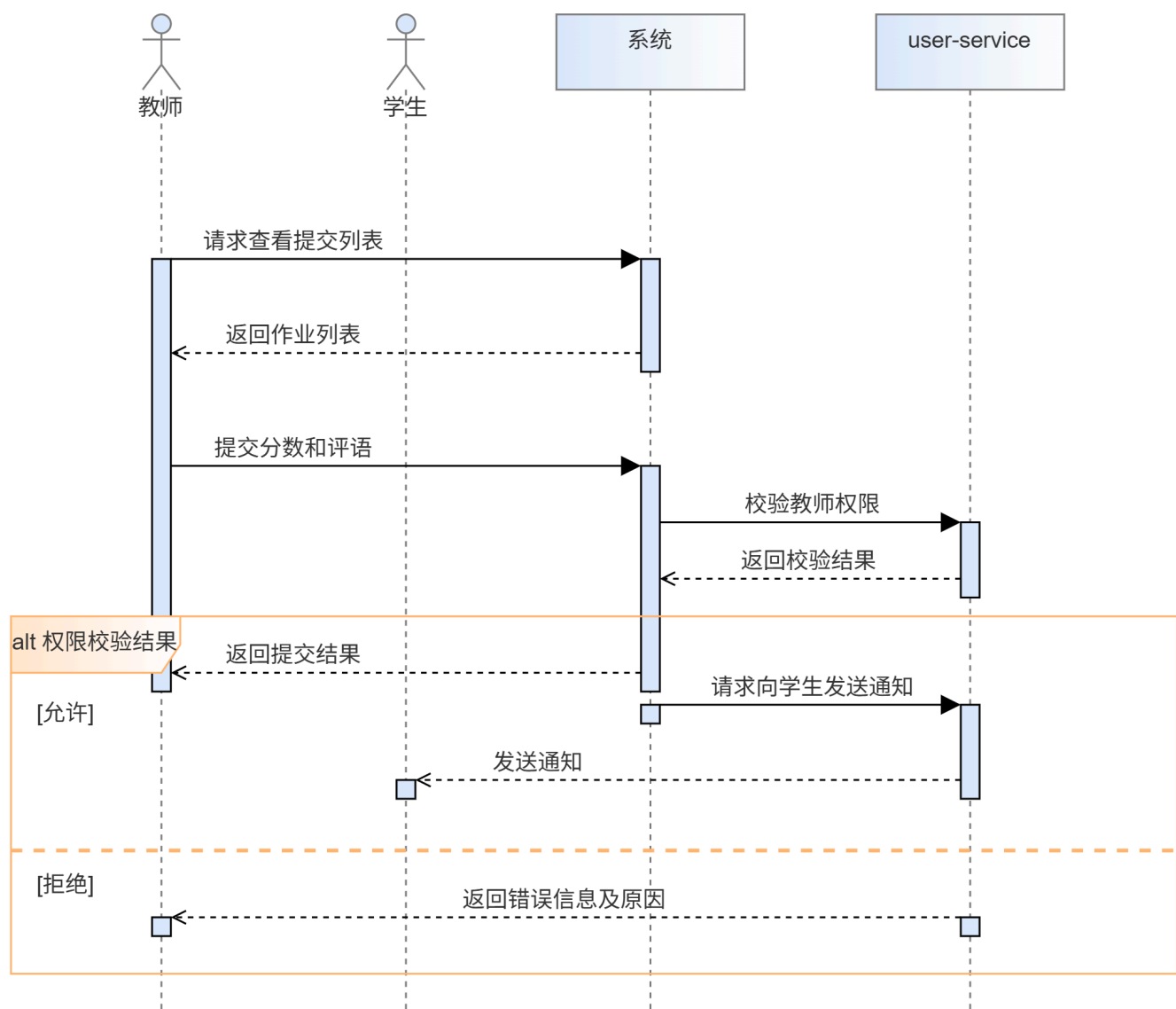
系统级顺序图（需求文档）：
