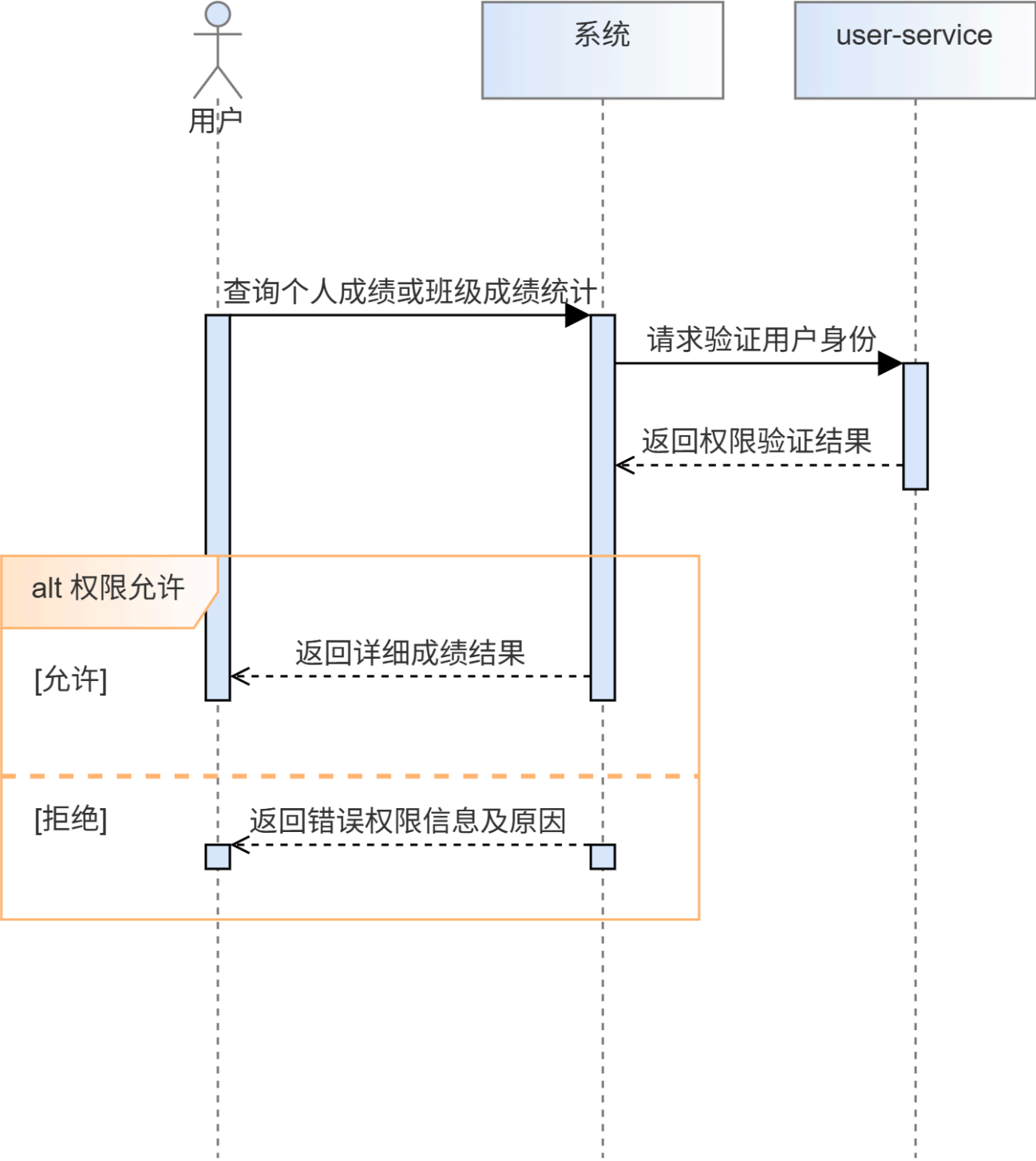
组件级顺序图（概要设计）：
