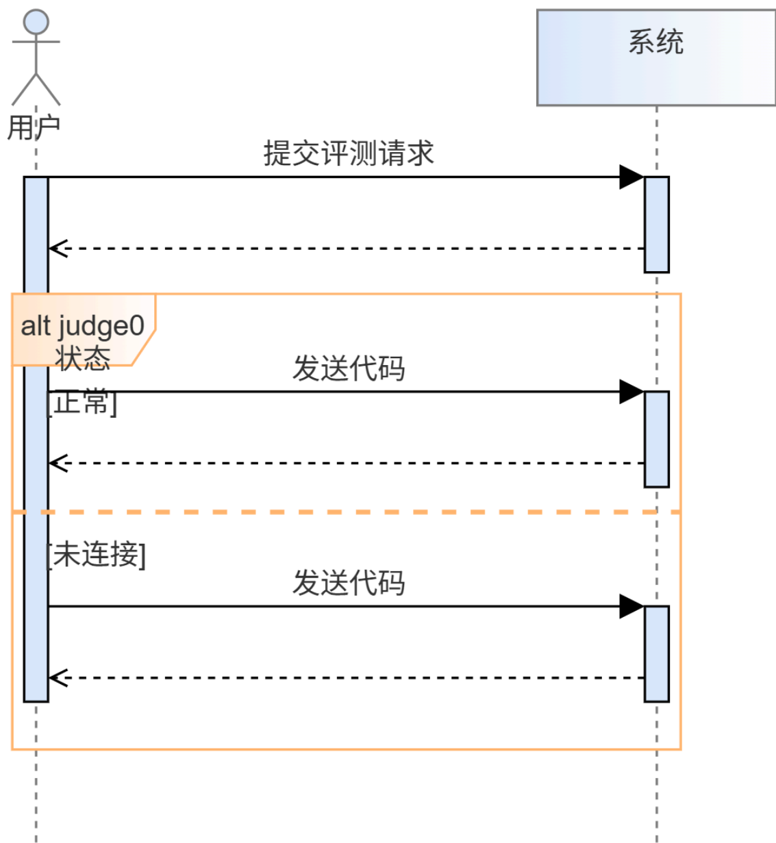
组件级顺序图（概要设计）：
