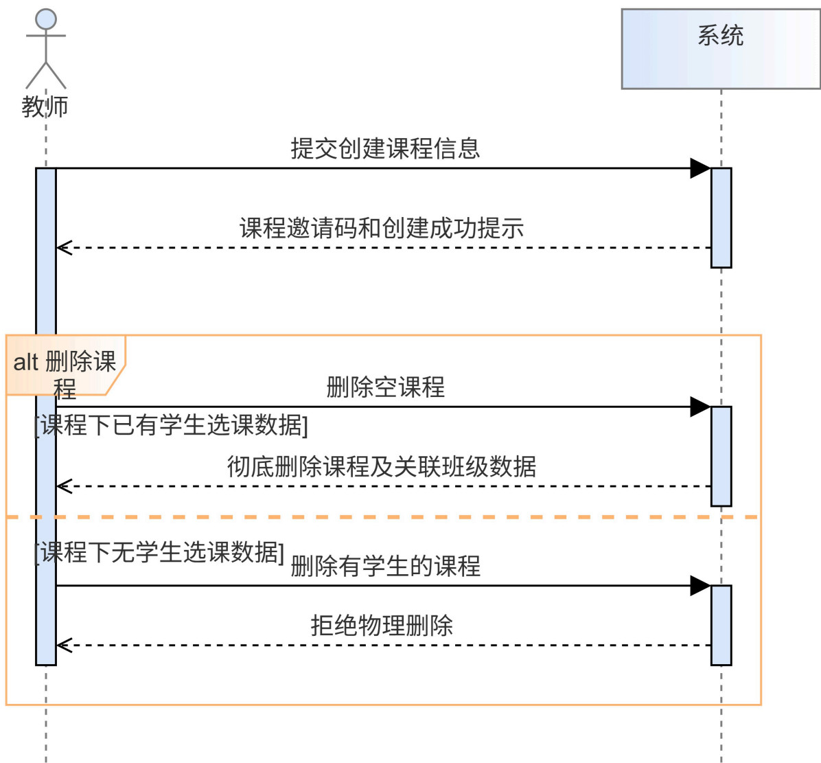
组件级顺序图（概要设计）：
