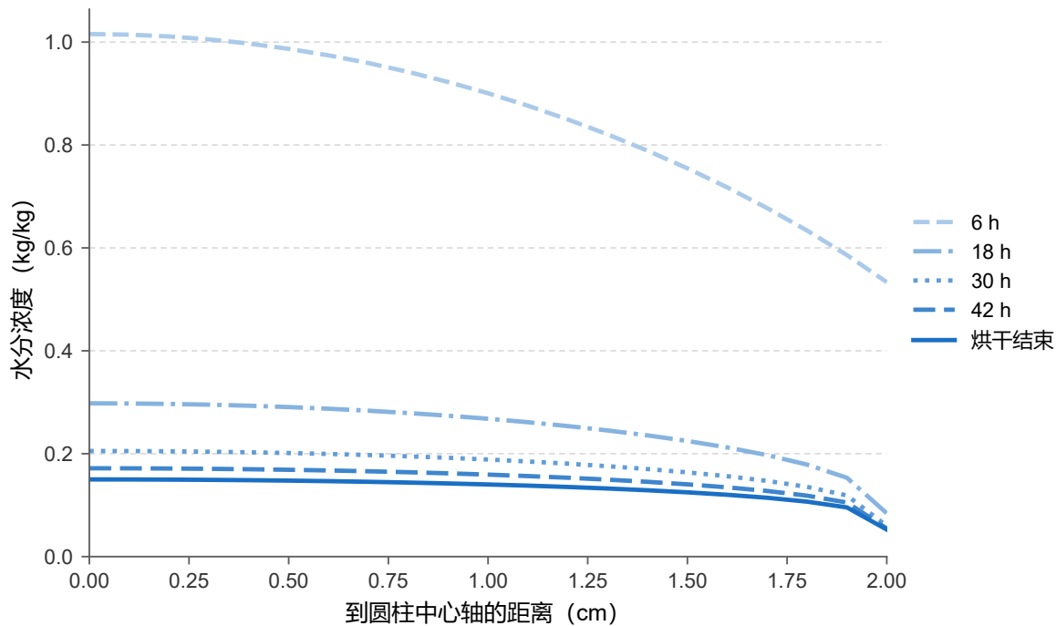
典型时刻径向水分浓度分布
