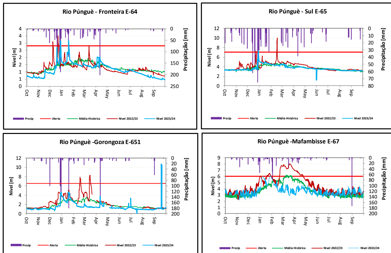
Figura 7 – Níveis hidrométricos registados na bacia do Púnguè no ano 2023/24.
