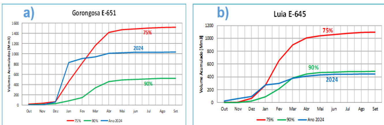
Figura 13 –Volumes mensais cumulativos. (a) no rio Púnguè em Gorongosa e (b) no rio Luia na bacia do Zambeze.
