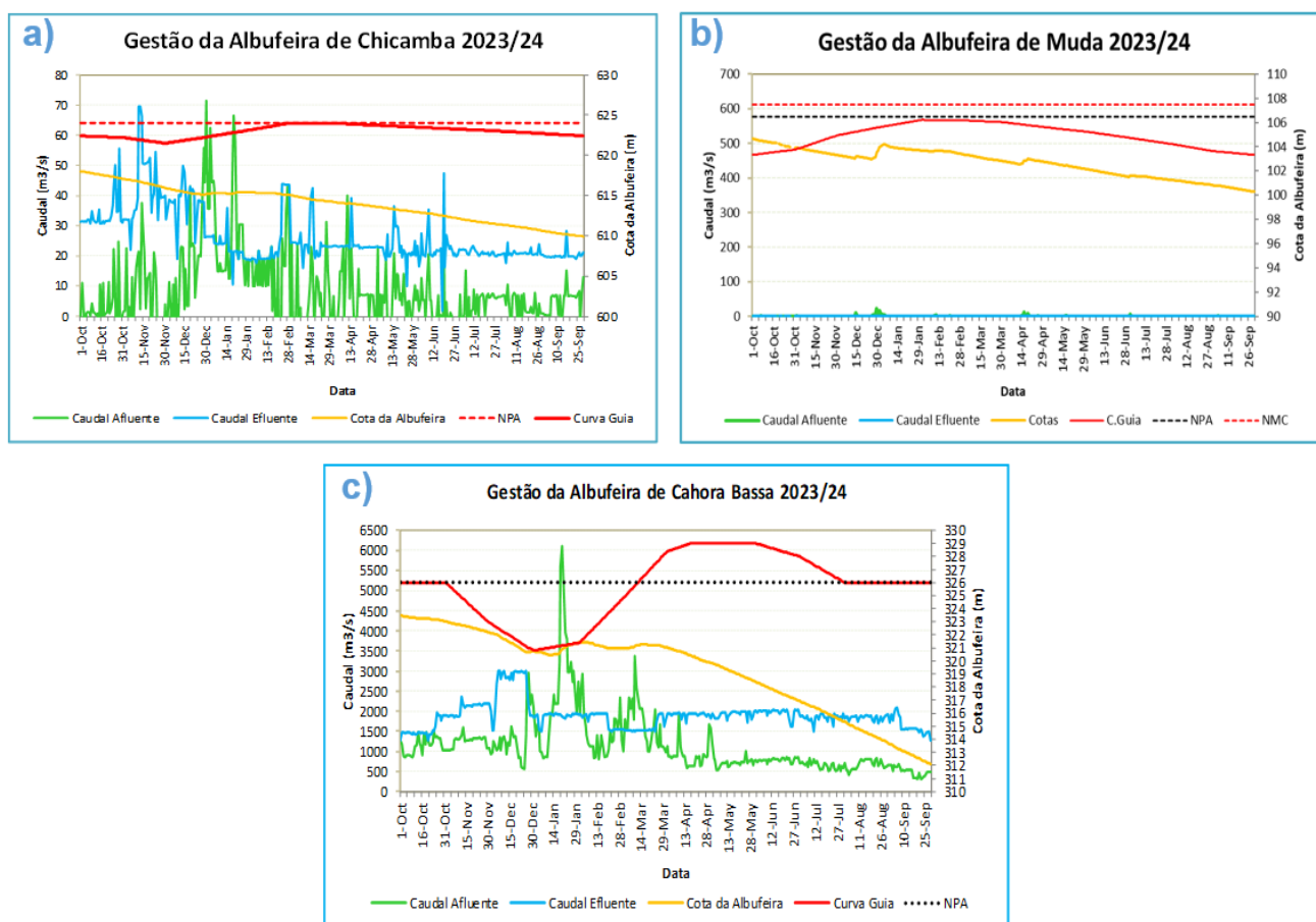
Figura 14– Gestão hidrológica das albufeiras no ano 2023/24: (a) Chicamba Real; (b) Muda Nhaurire e (c) Cahora Bassa.
