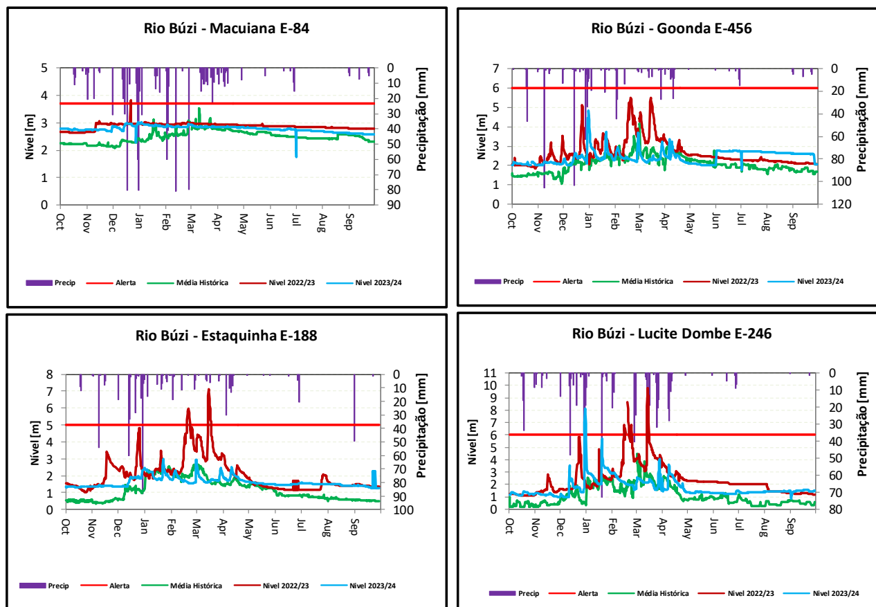
Figura 5 – Níveis hidrométricos registado na bacia do Búzi no ano 2023/24.
