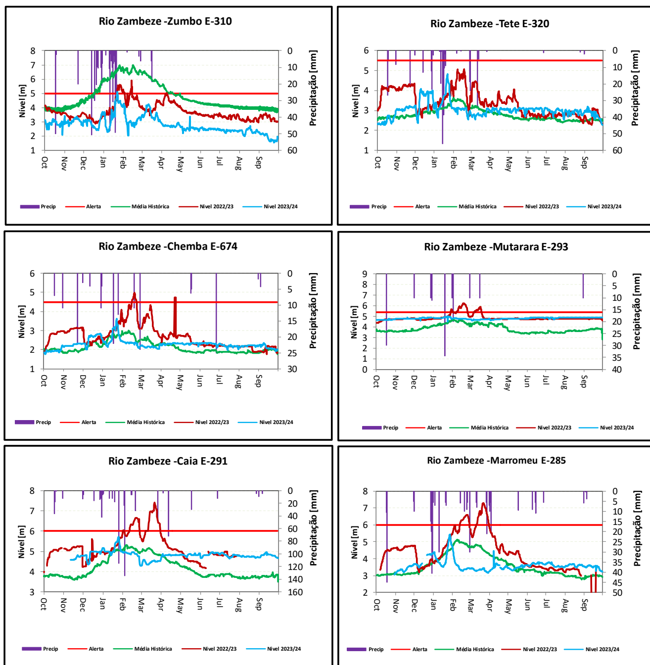
Figura 9 – Níveis hidrométricos registado na bacia do Zambeze no ano 2023/24.
