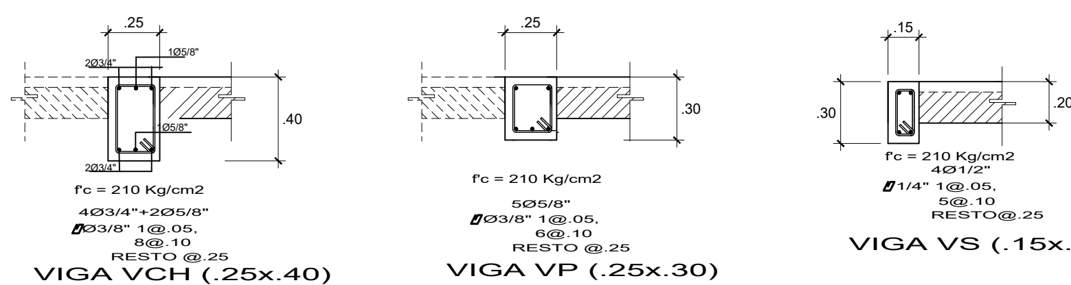
PRIMER PISO (S/C = 200 Kg/m²)
