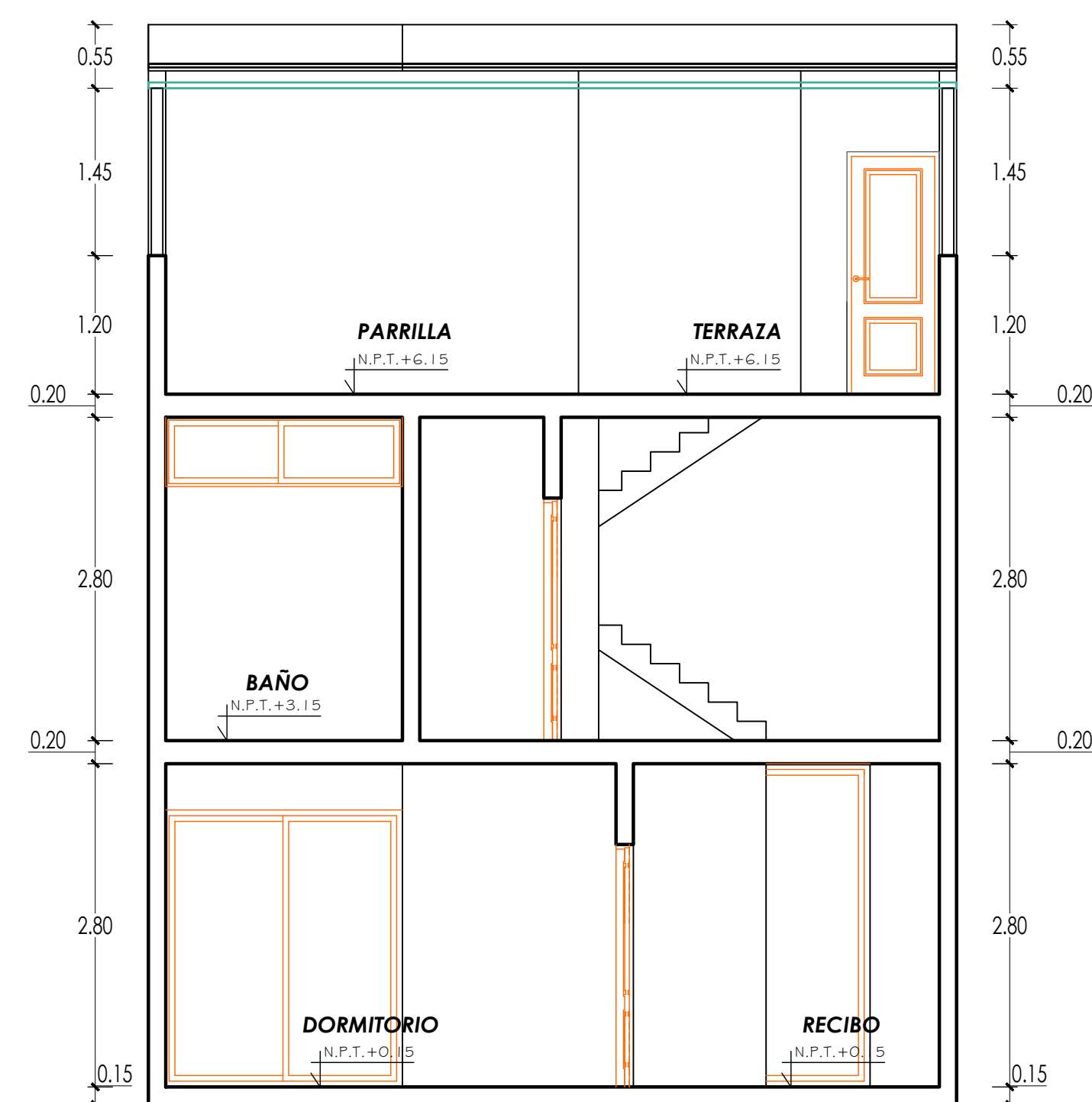
SECCIÓN C - C Esc: 1/50
