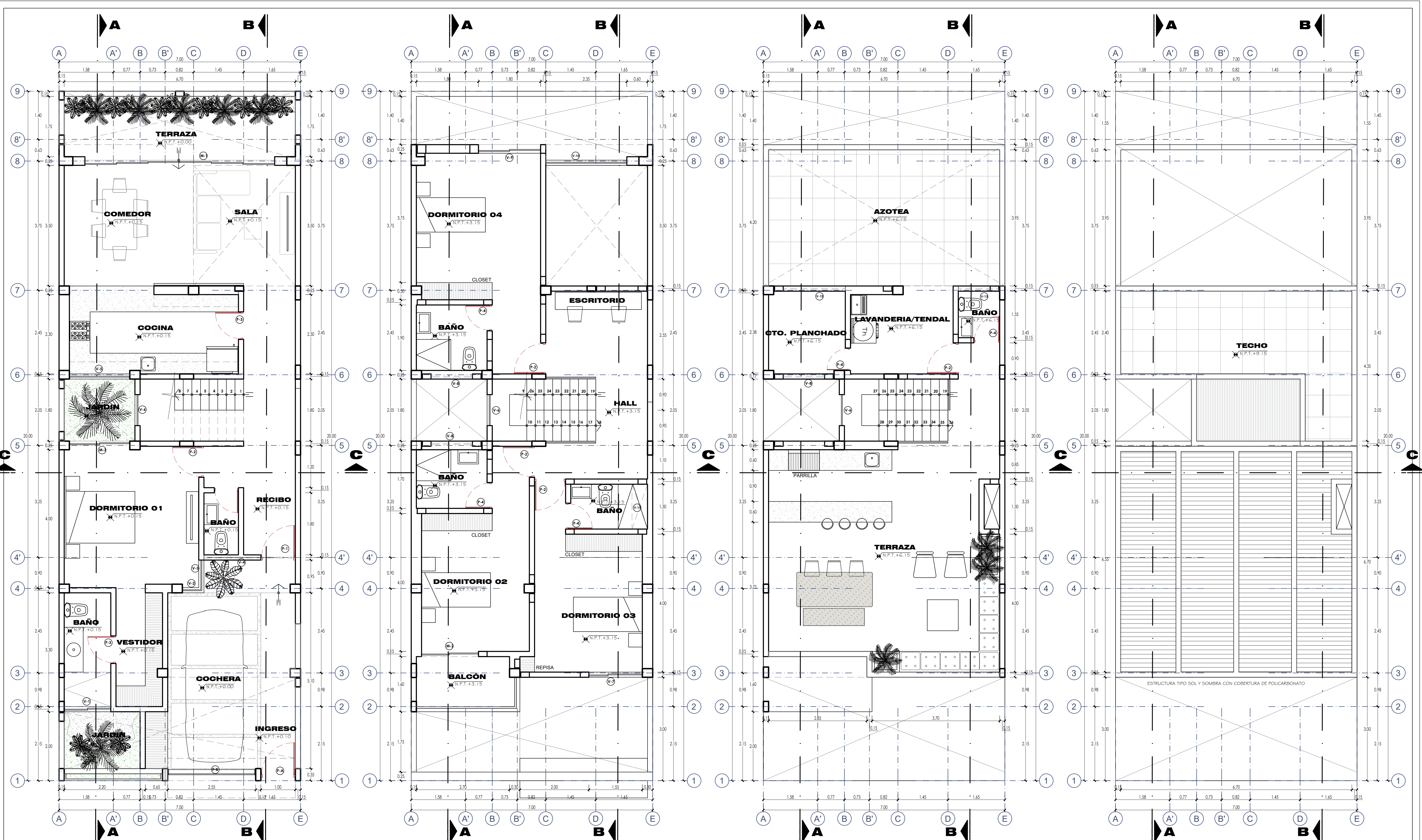
PLANTA PRIMER PISO Esc: 1/50
