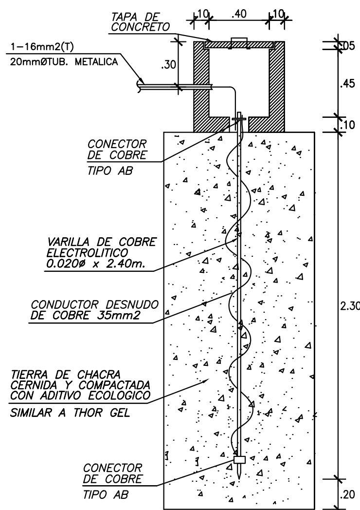
POZO DE TIERRA RESISTENCIA <20 ohmios Esc. = 1/25
