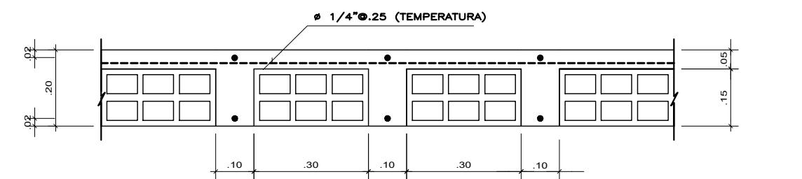
DETALLE TIPICO DE ALIGERADO h=0.20
