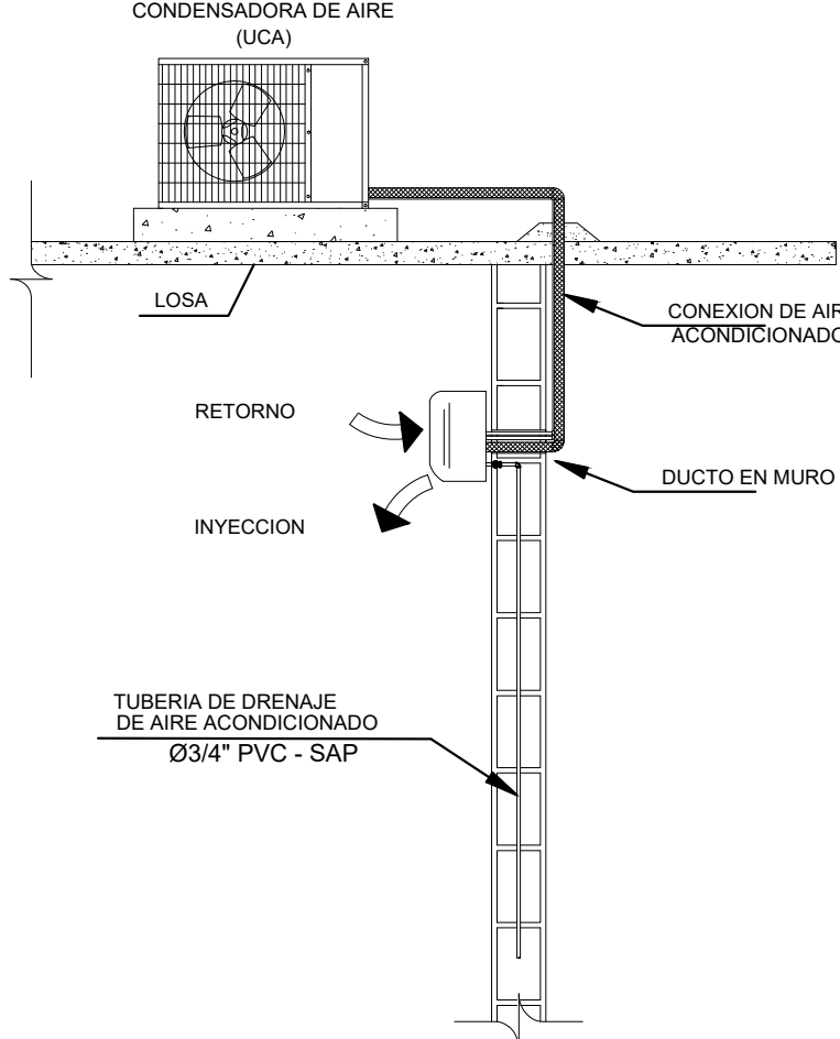
DETALLE - 01 INSTALACION TIPO DE UNIDAD EN MURO
