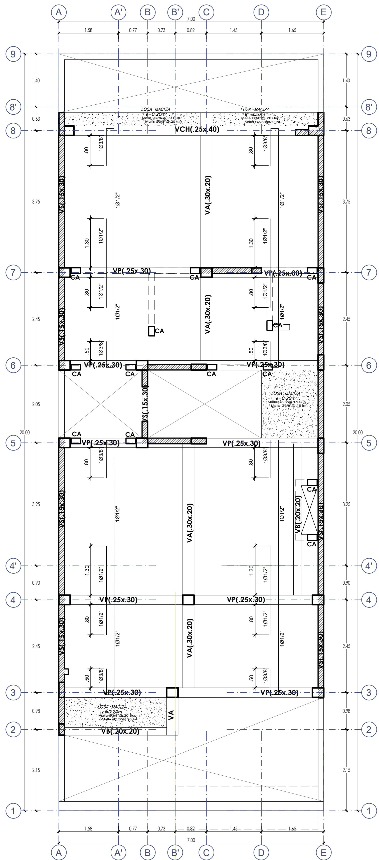
SEGUNDO PISO (S/C = 200 Kg/m²)
