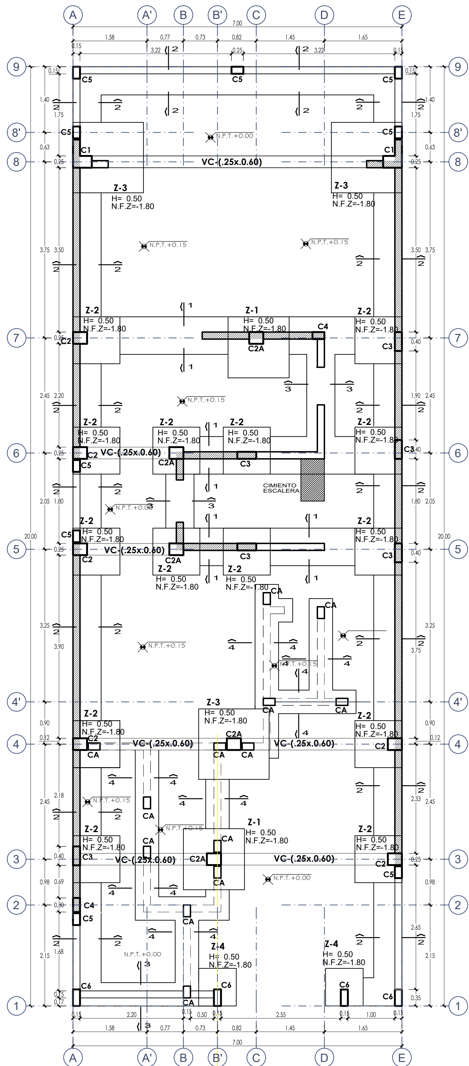
CIMENTACION Escala 1/50
