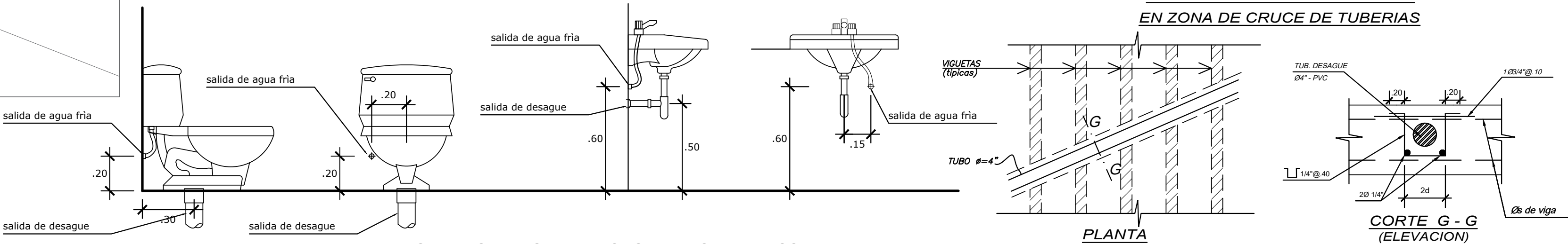
DETALLE DE SALIDAS DE AGUA Y DESAGUE EN SANITARIOS ESC 1/20
