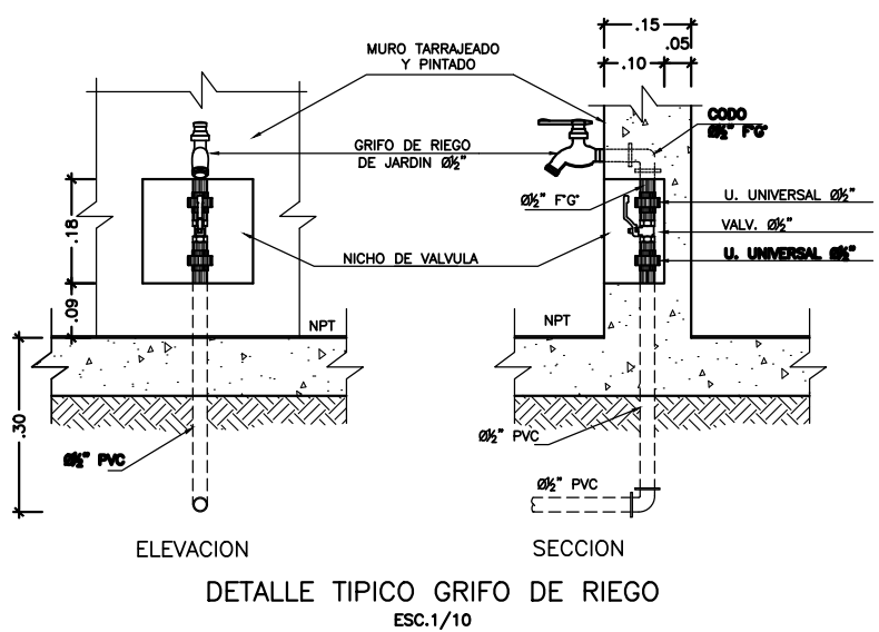
DETALLE TÍPICO GRIFO DE RIEGO ESC:1/10
