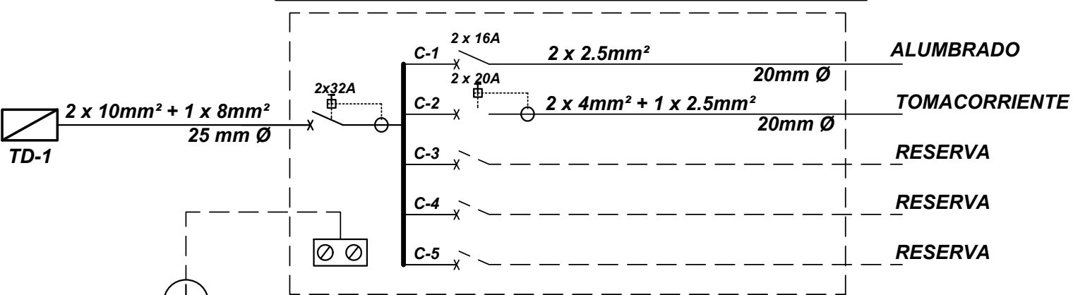
DIAGRAMA UNIFILAR TABLERO AZOTEA (TD3)
