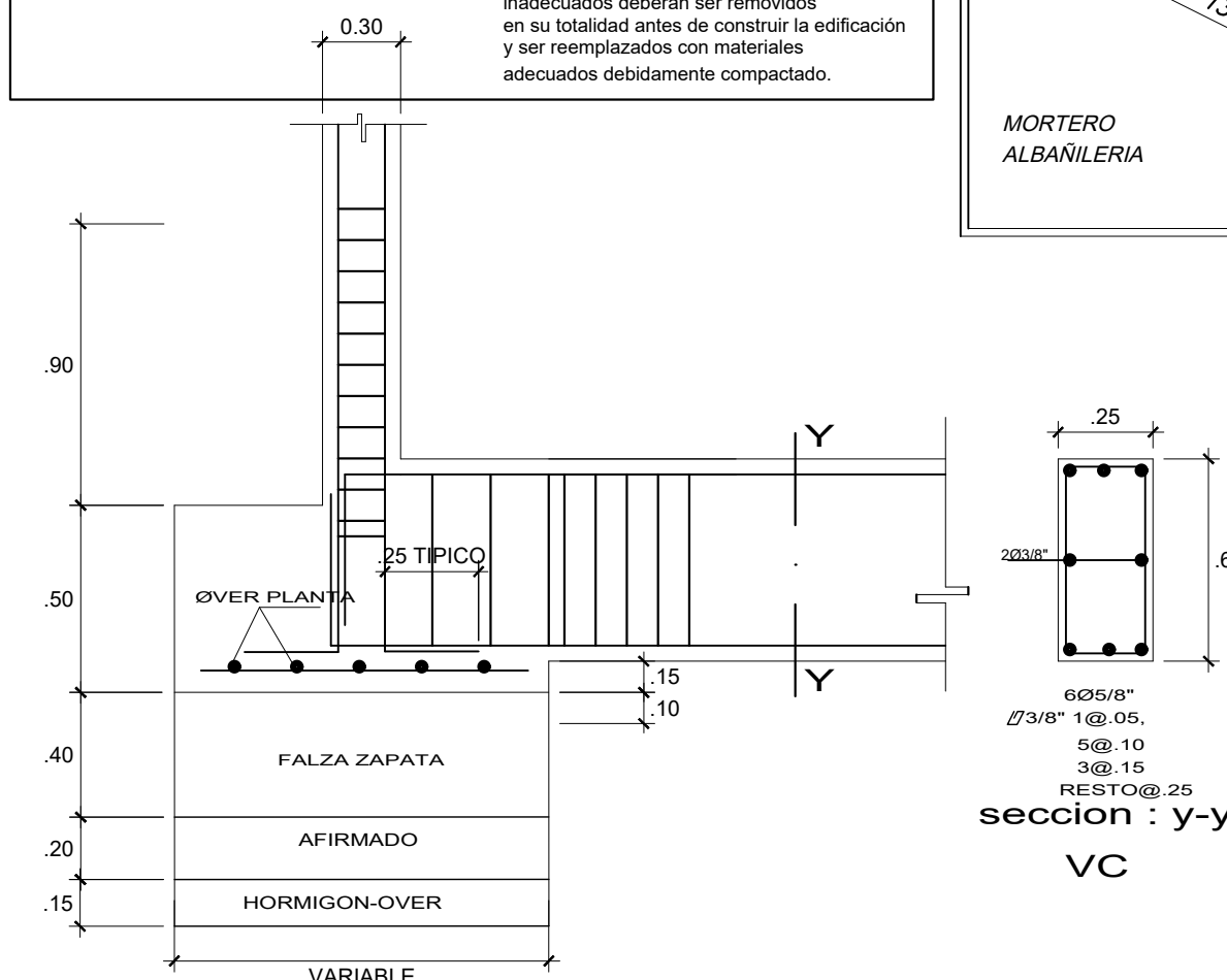
DETALLE TIPICO DE VIGA DE CIMENTACION e = 1/25
