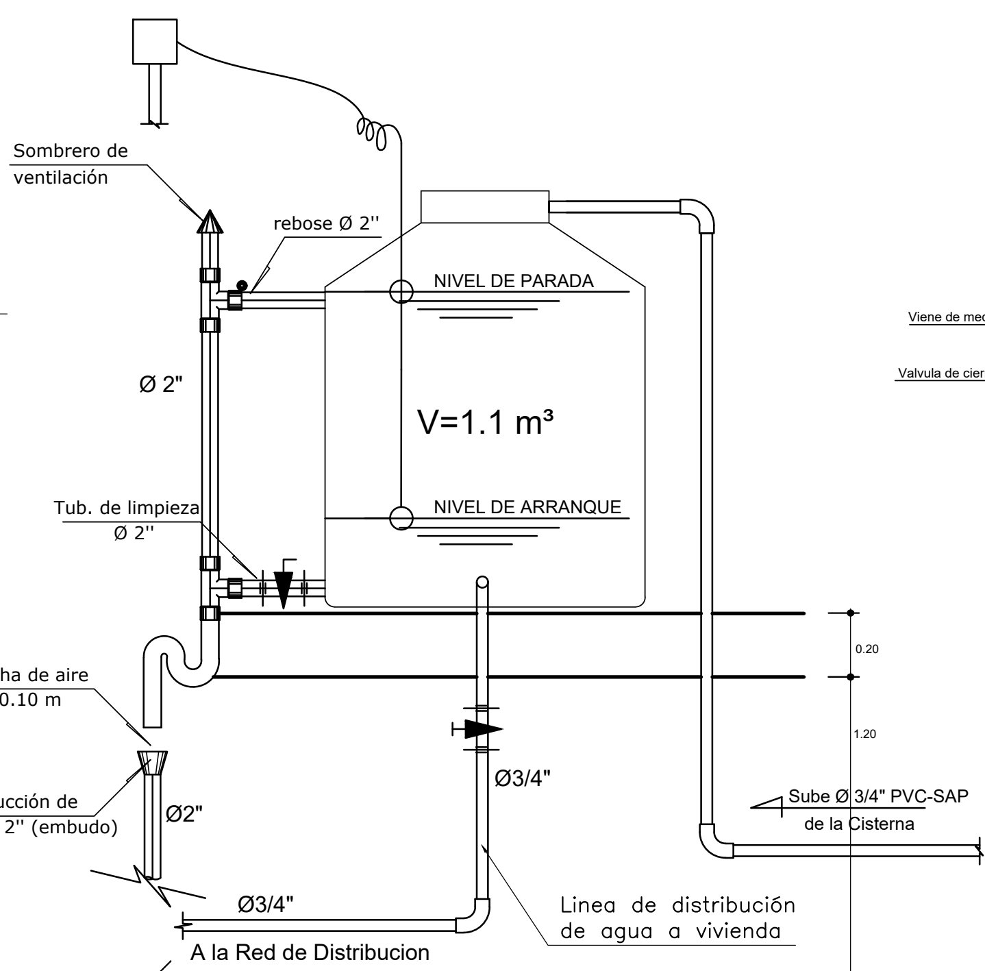
TANQUE ELEVADO ESC 1/25
