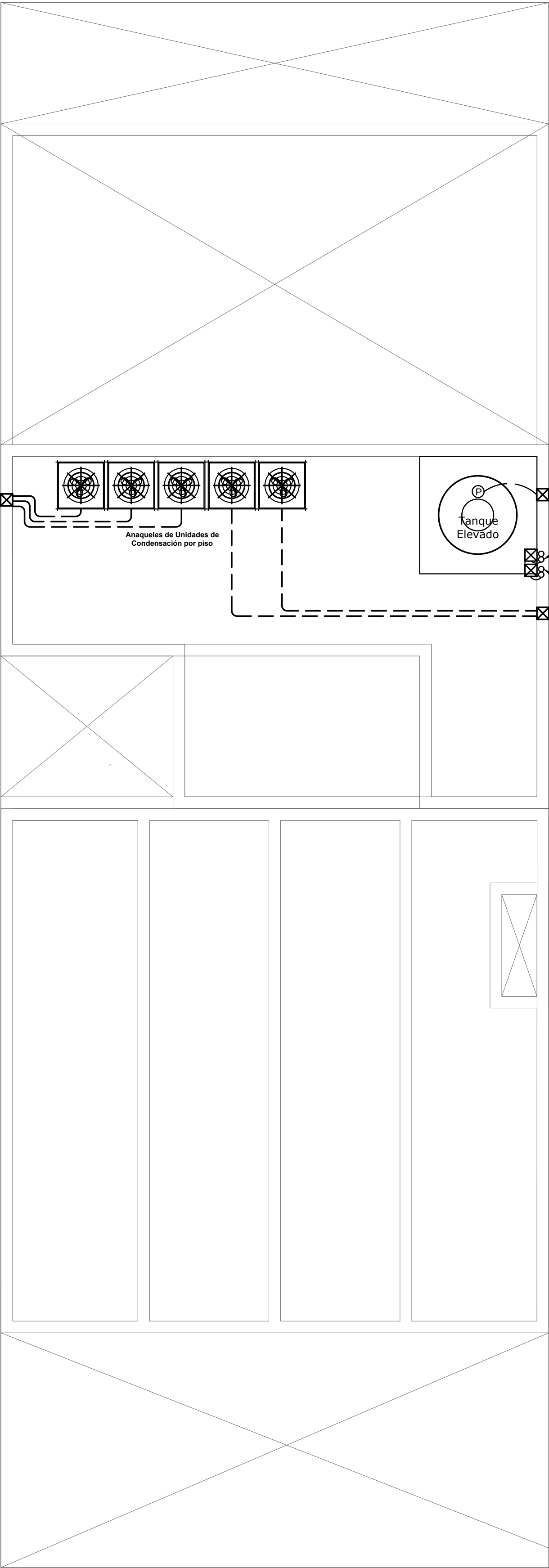
PLANTA TECHO ESC:1/50
