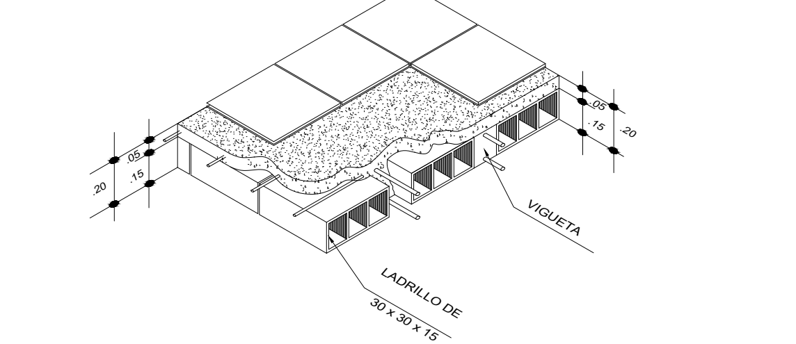
DETALLE TIPICO DE ALIGERADO h=0.20
