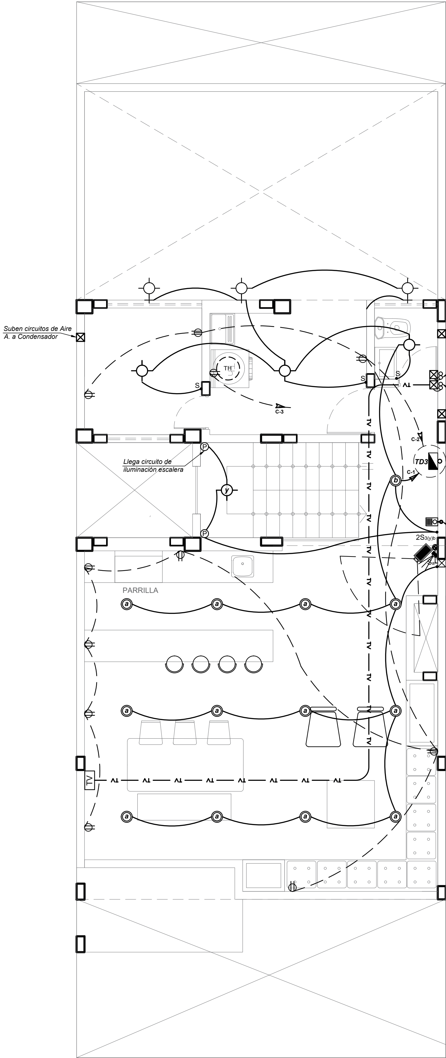
PLANTA AZOTEA ESC:1/50
