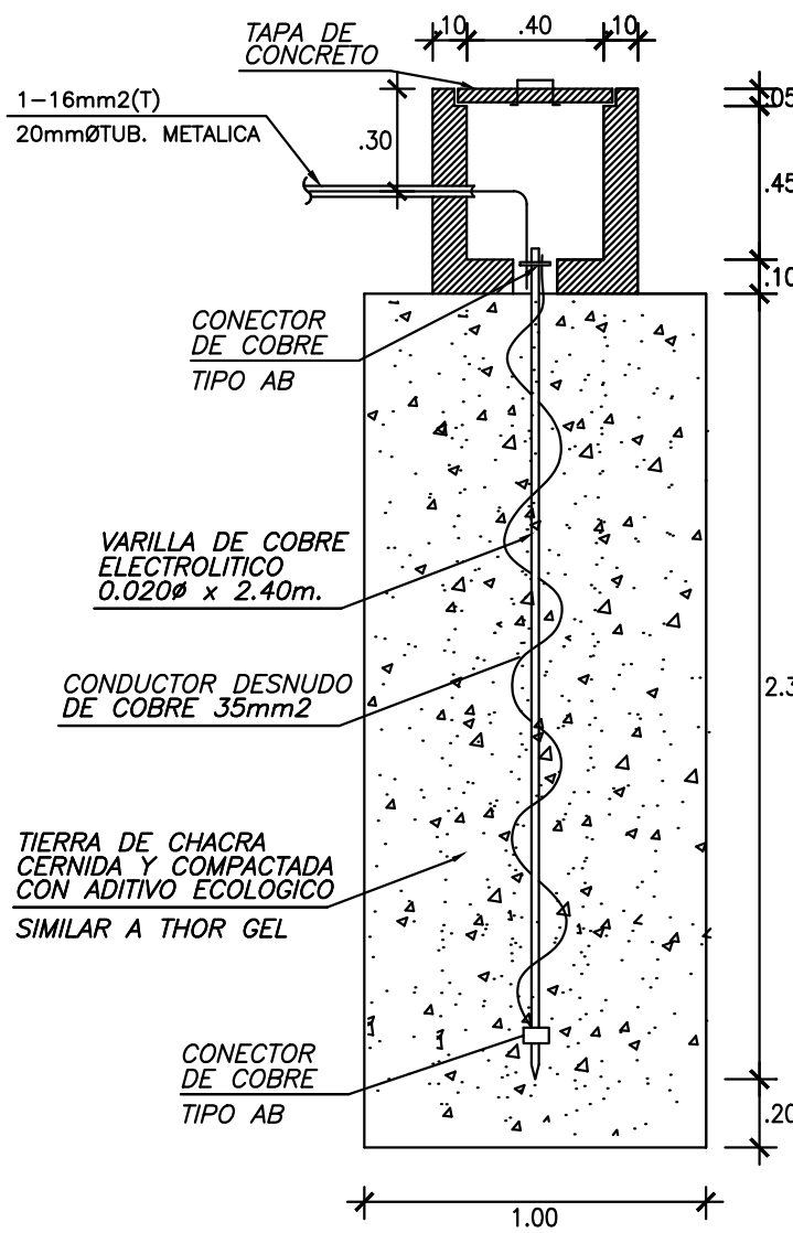
POZO DE TIERRA RESISTENCIA <20 ohmios Esc. = 1/25
