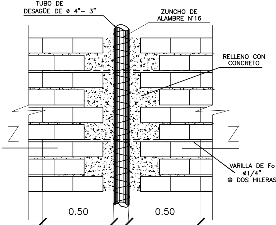
DETALLE DE REFUERZO PARA TUBERIA DE \phi 4" ESC. 1/20
