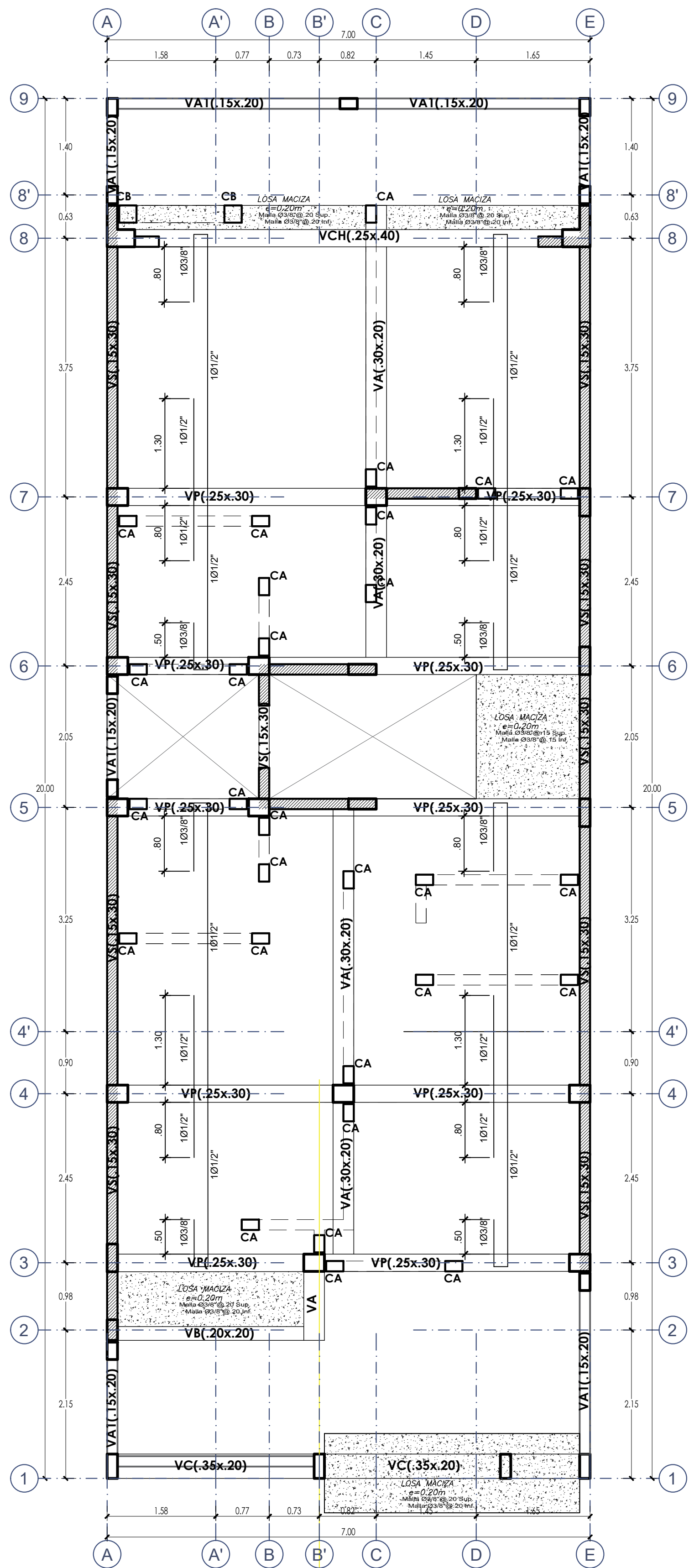
PRIMER PISO (S/C = 200 Kg/m²)
