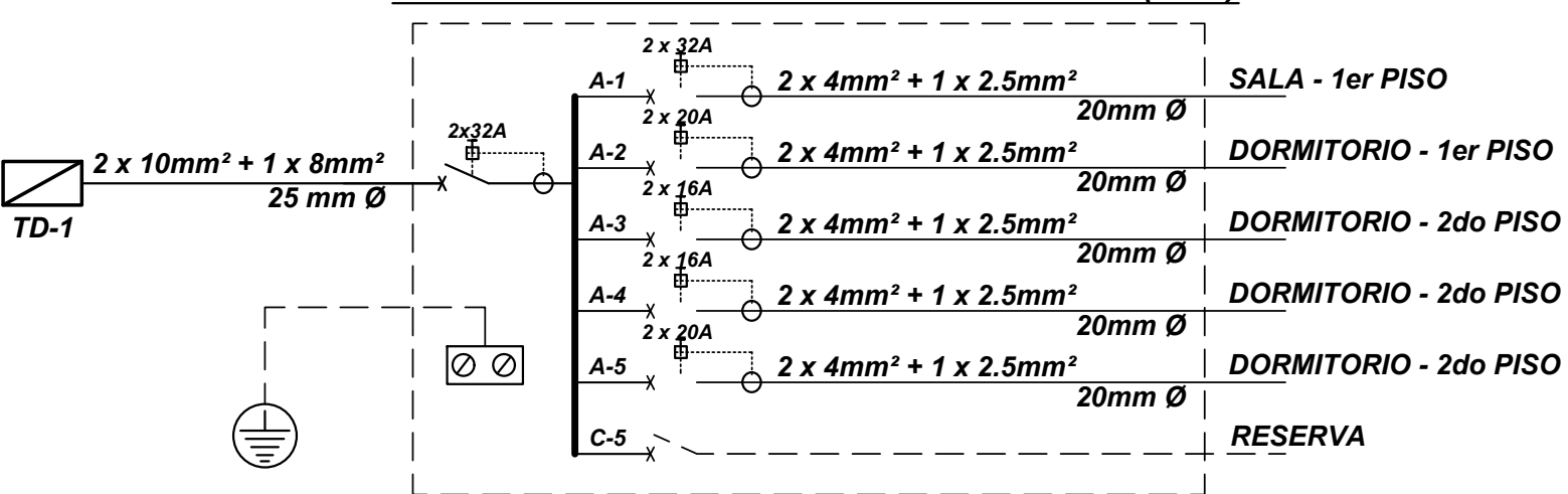
DIAGRAMA UNIFILAR TAB. AIRE ACOND. (TAA)
