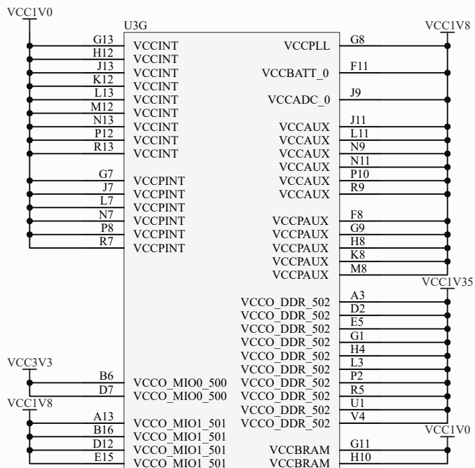
XC7Z010-2CLG400I
