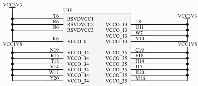
XC7Z010-2CLG400I
