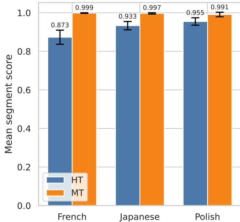
LitTransProQA
