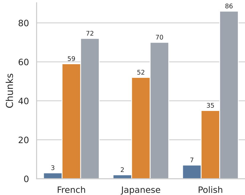
LitTransProQA
