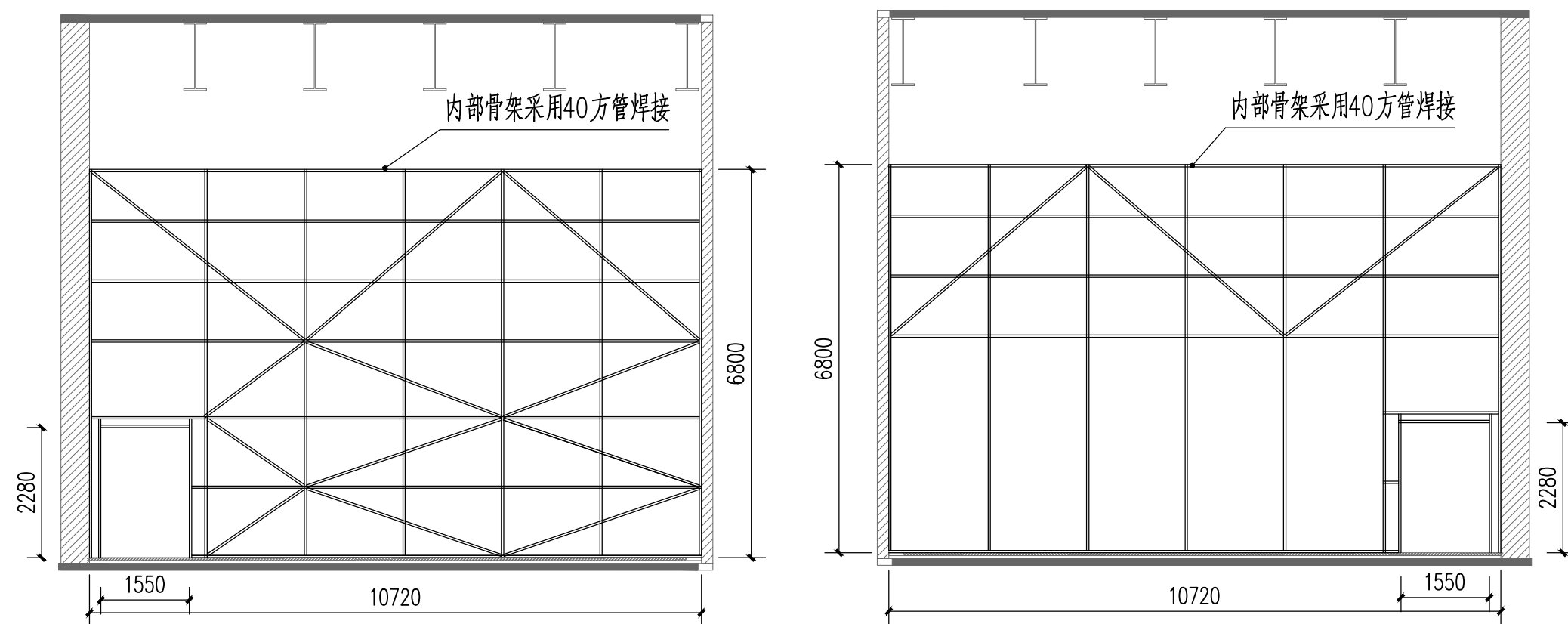
隔墙短边A立面钢骨架图 1:100
