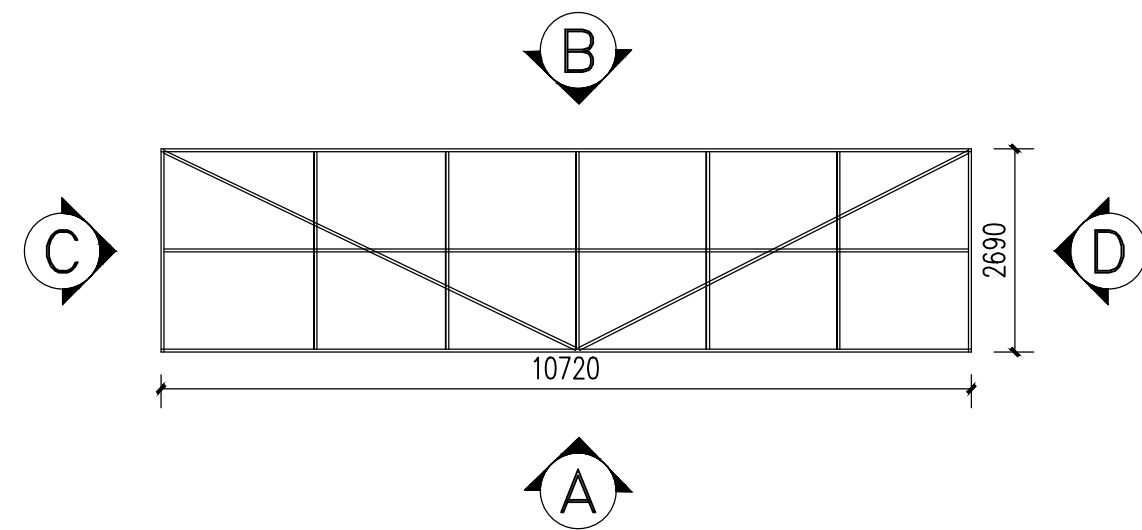
① 隔墙短边平面钢骨架图 1:100
