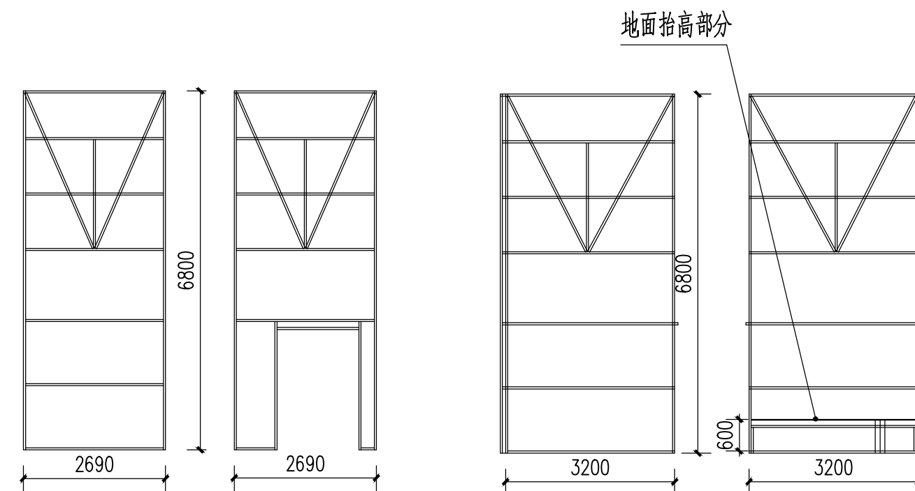
隔墙短边CD立面钢骨架图 1:100
