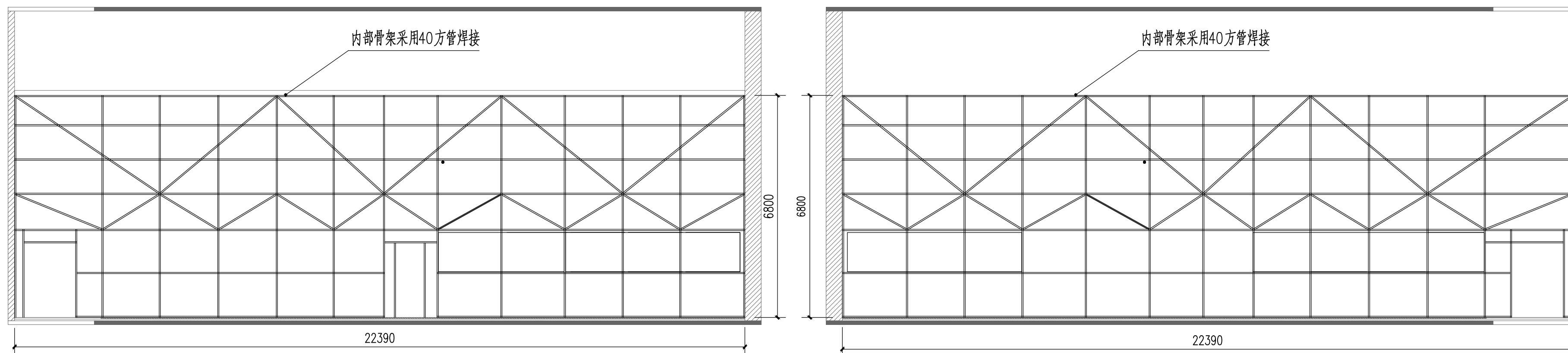
隔墙长边A立面钢骨架图 1:100
