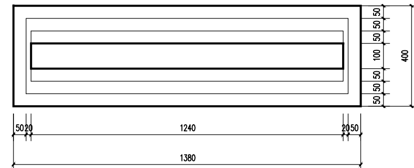
隔断 顶视图 1:15
