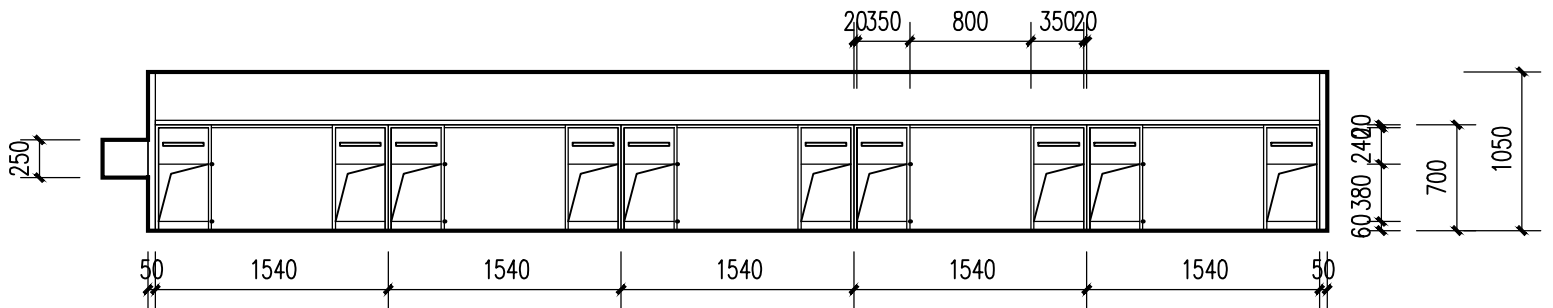
西服务台 后视图 1:50
