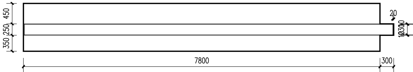
西服务台 前视图 1:50
