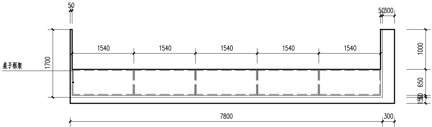
西服务台 顶视图 1:50
