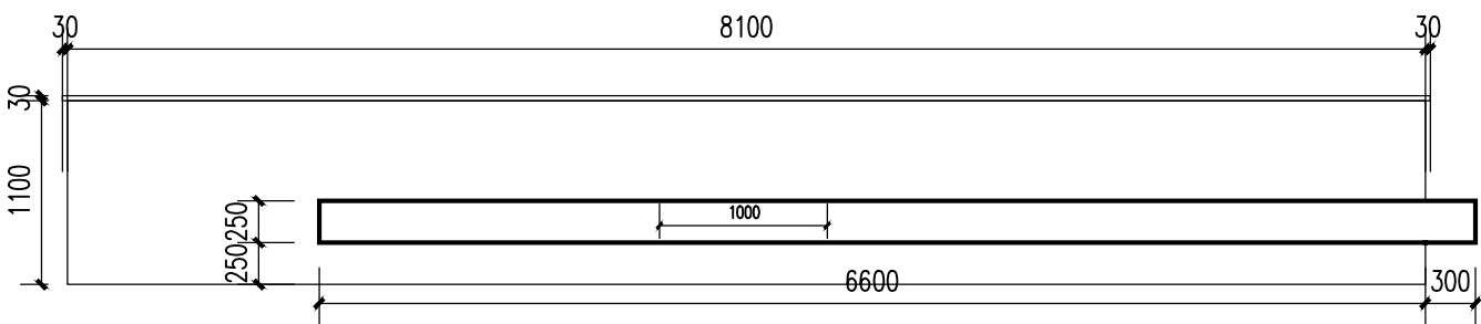
南欢迎台 前视图 1:50
