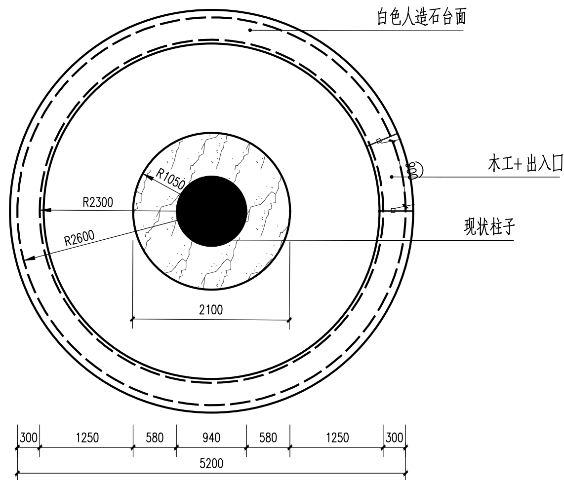
水吧 平面图 1:50
