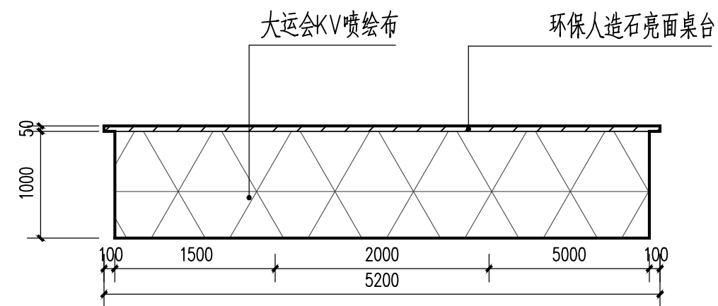
水吧外吧台 正视图 1:50
