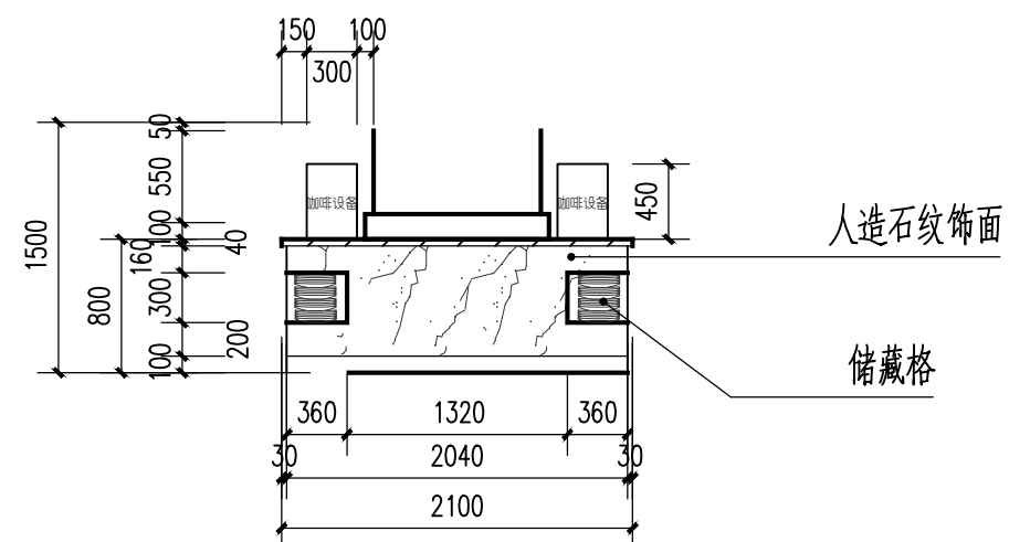
水吧内吧台 侧视图 1:50
