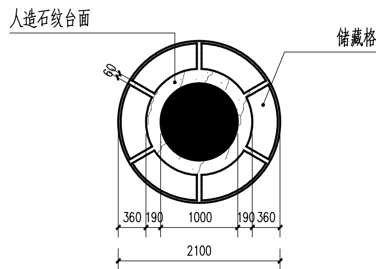
水吧内吧台 平面图 1:50
