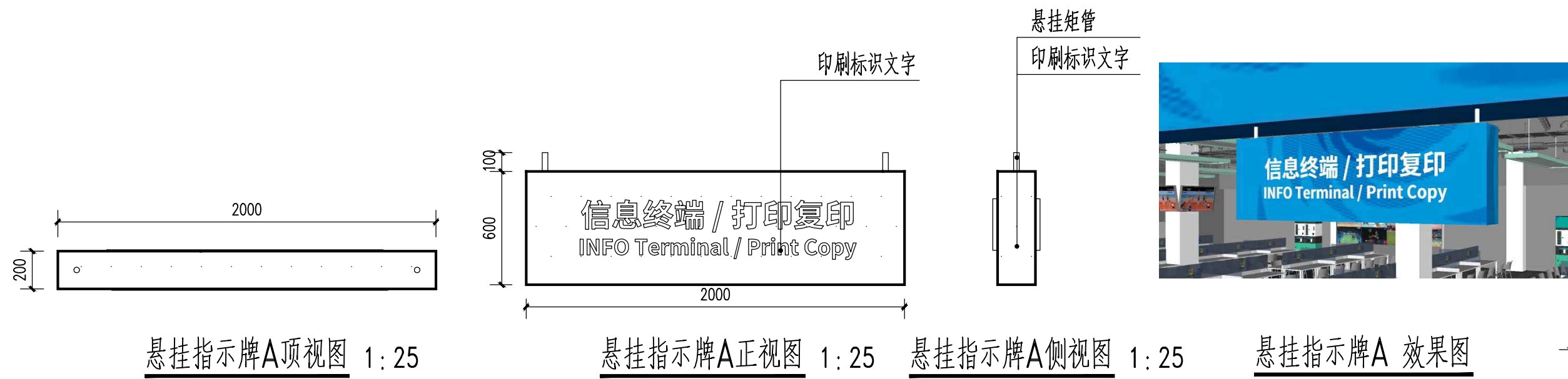
① 悬挂指示牌A大样图 1:25
