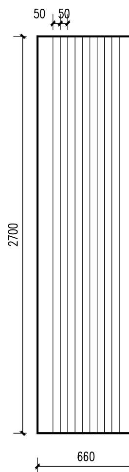
餐厅柱饰面 侧视图 1:25
