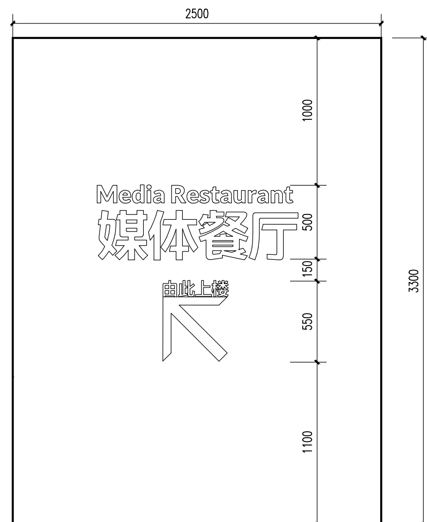
餐厅指示A 正视图 1:25
