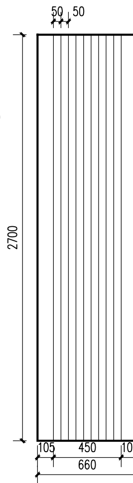
餐厅柱饰面 正视图 1:25
