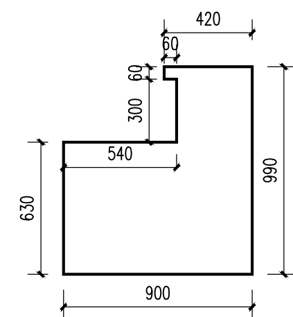
餐厅服务台 侧视图 1: 25
