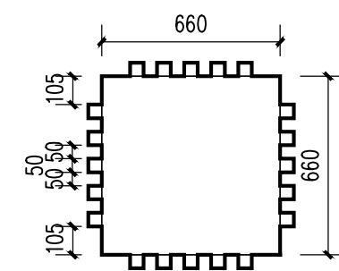
餐厅柱饰面 顶视图 1: 25
