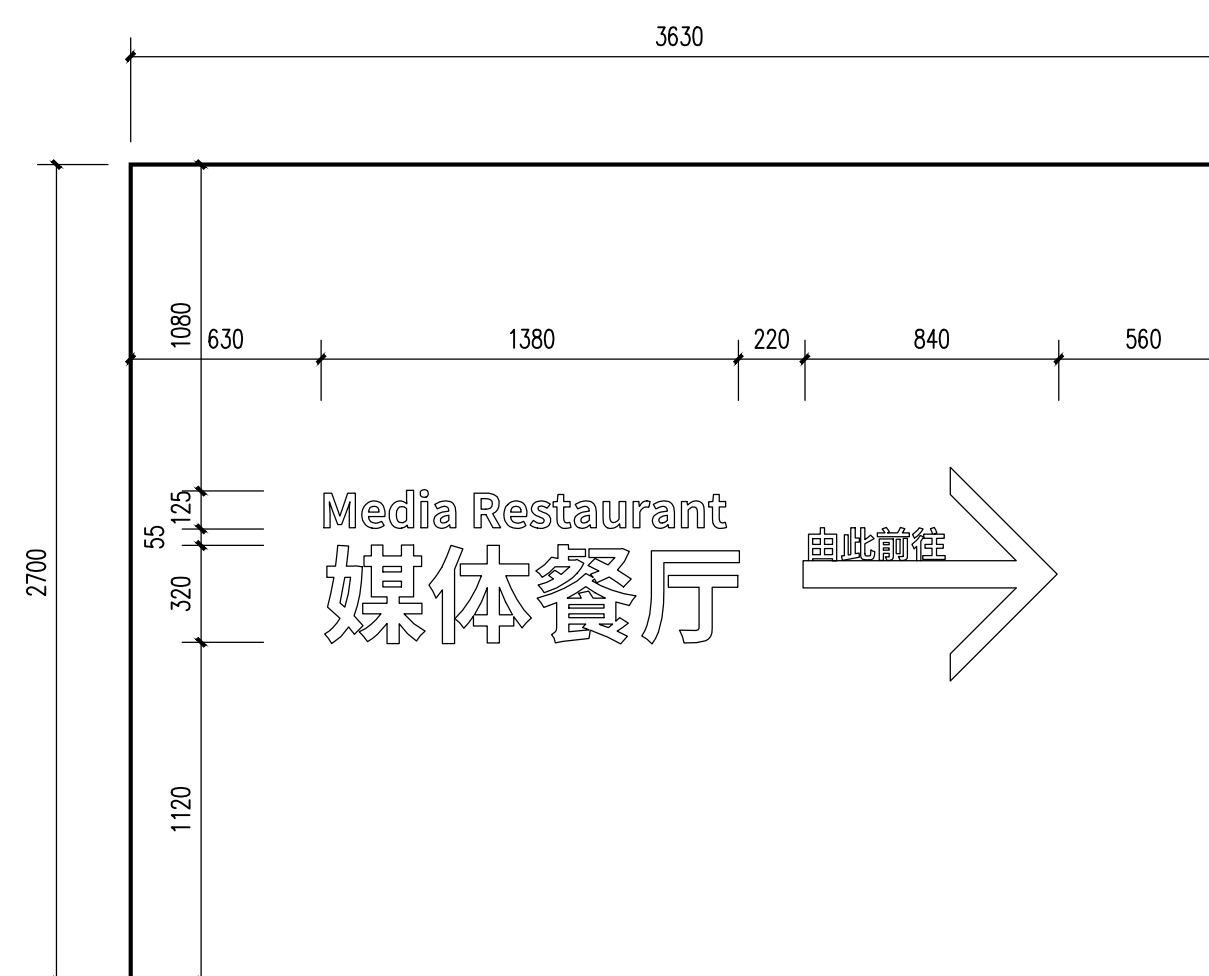
餐厅指示B 正视图 1:25
