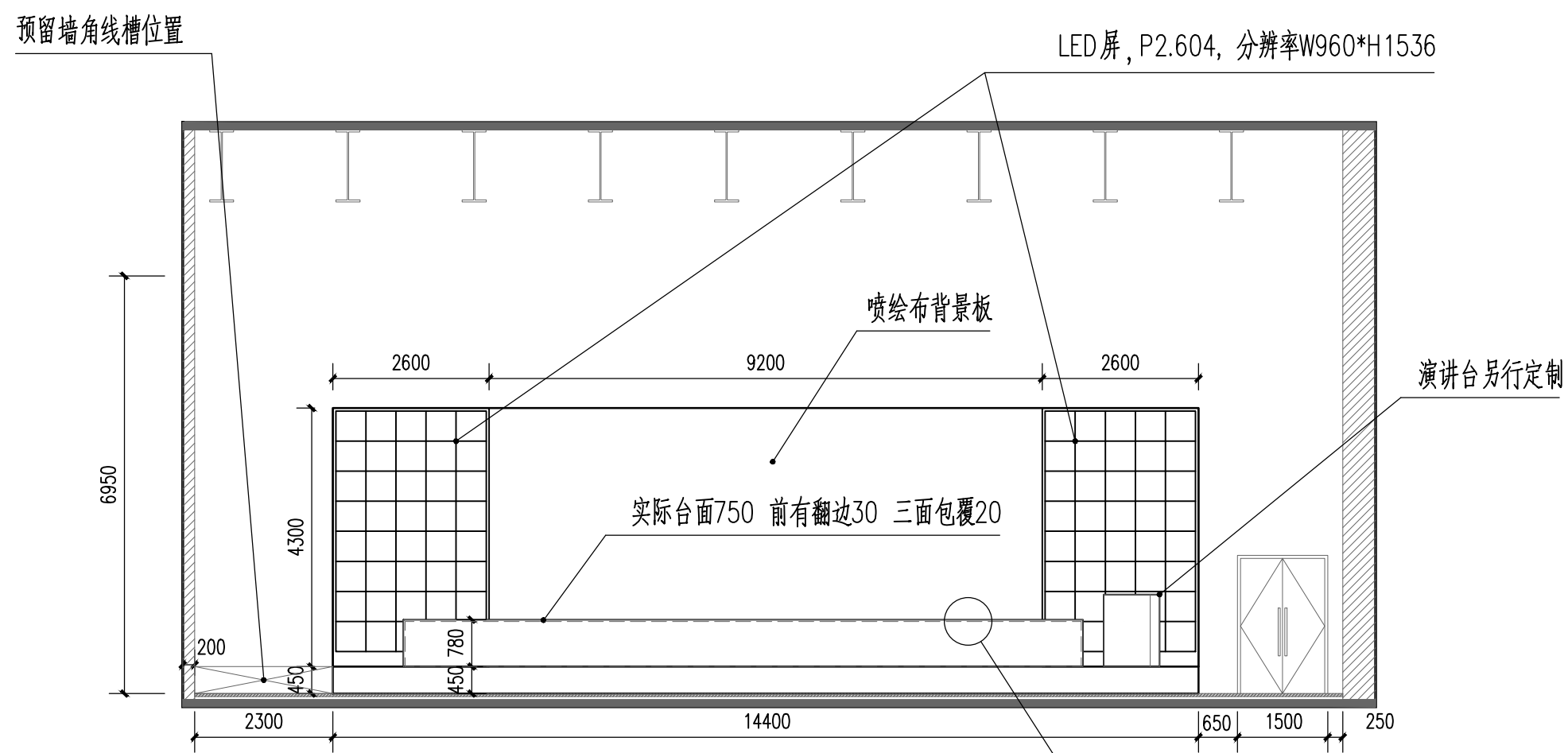
发布厅1 C立面图 1:100
