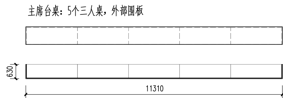
① 发布厅1主席台桌子详图 1:100
