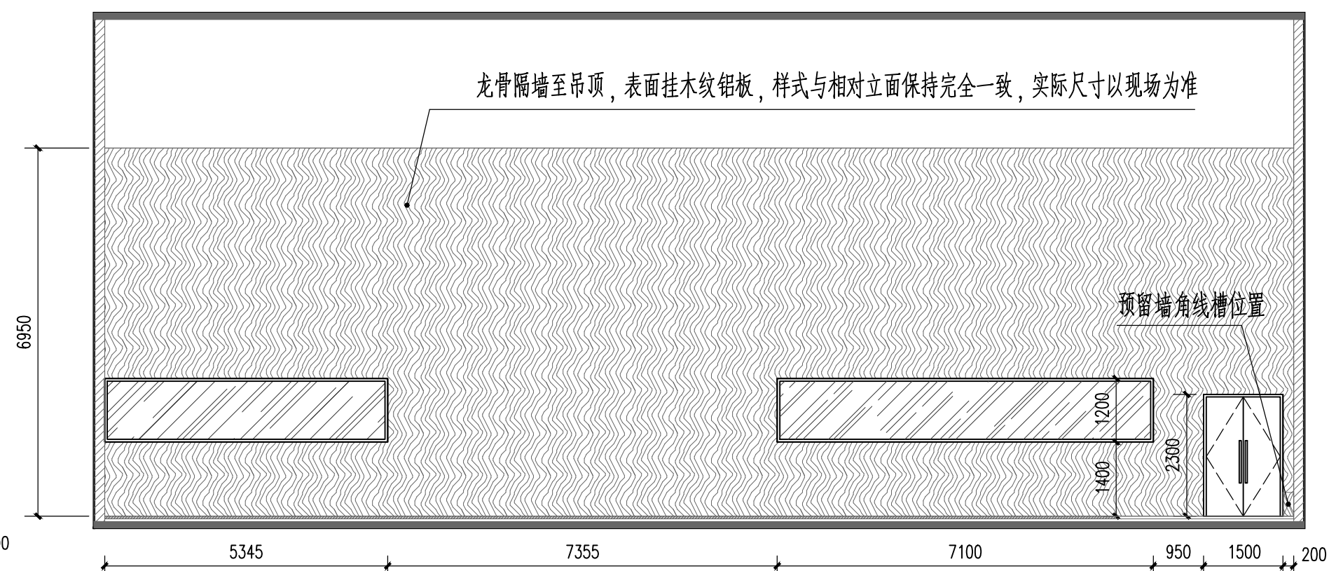
发布厅1 B立面图 1:100
