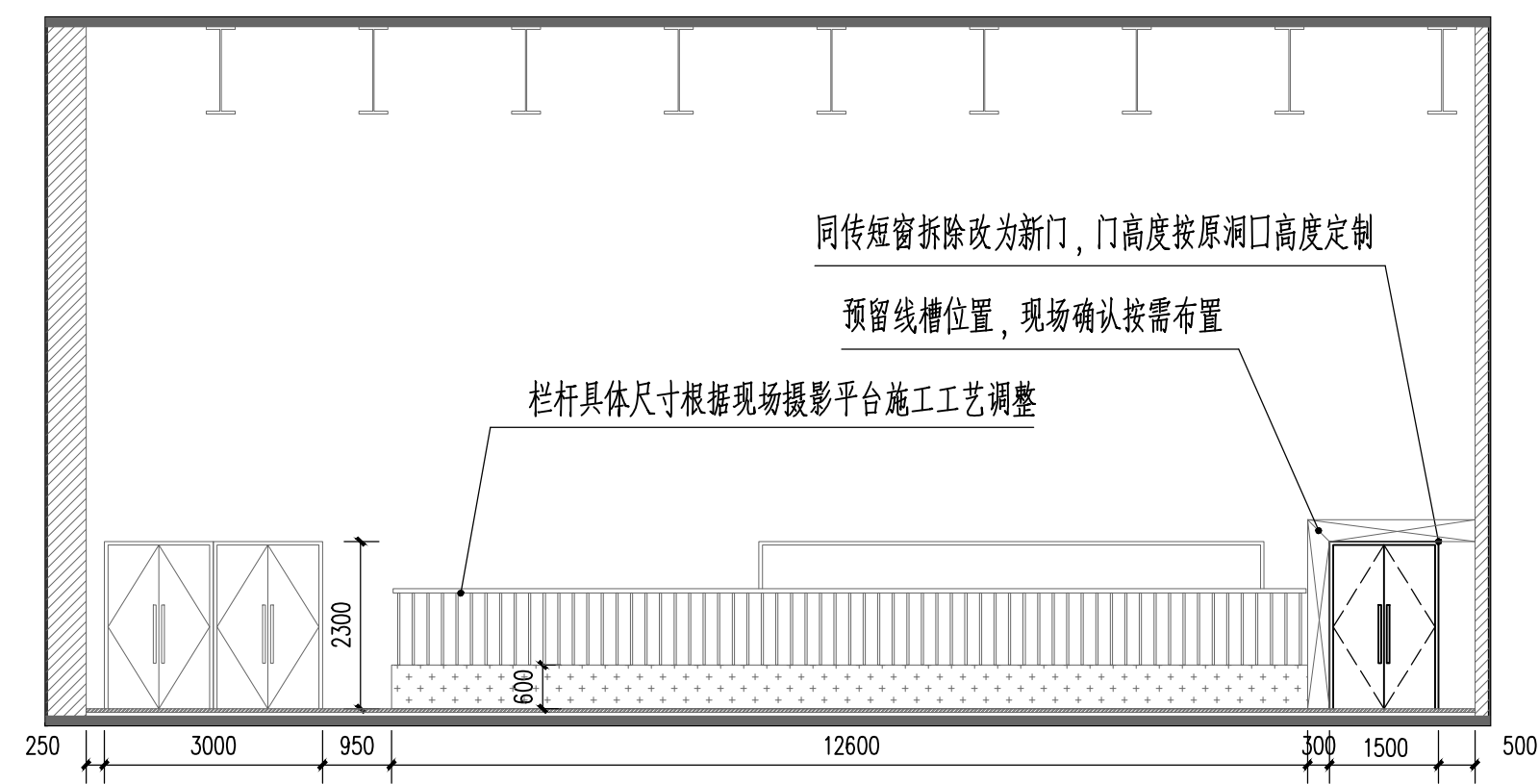
发布厅1 A立面图 1:100
