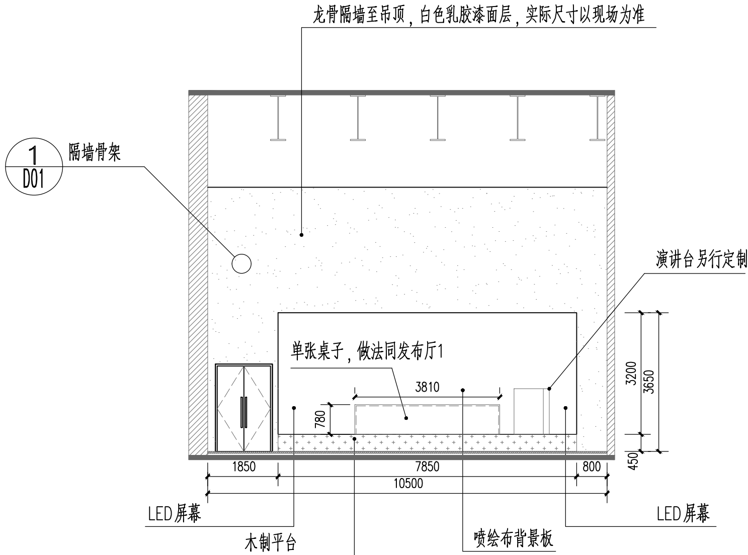
发布厅2 C立面图 1:100
