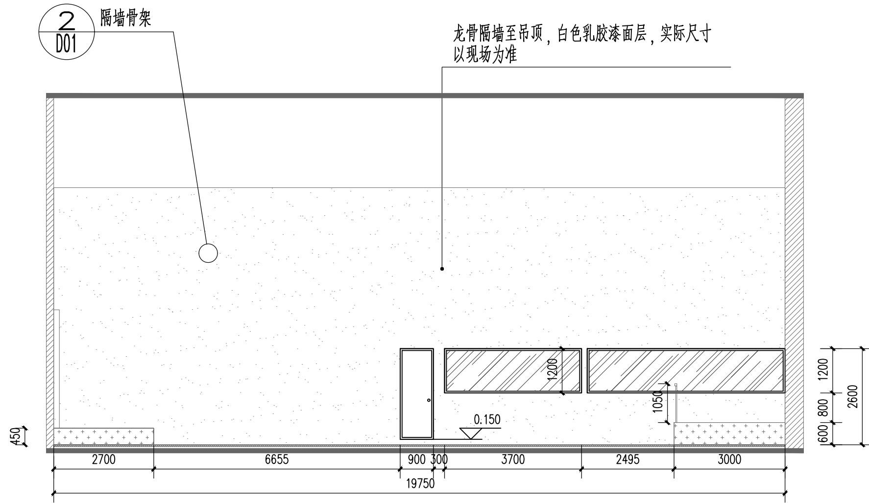
发布厅2 A立面图 1:100
