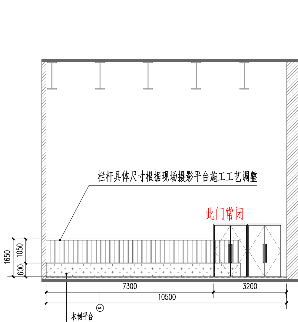
发布厅2 B立面图 1:100
