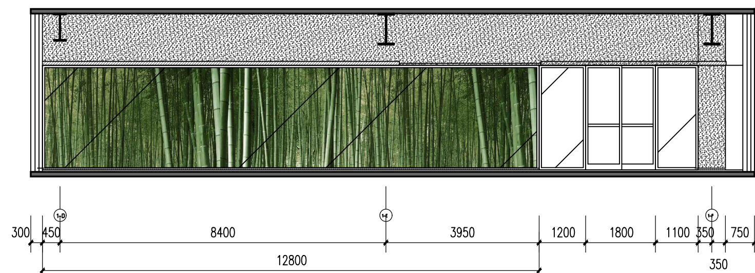
媒体餐厅 G立面图 1:100
