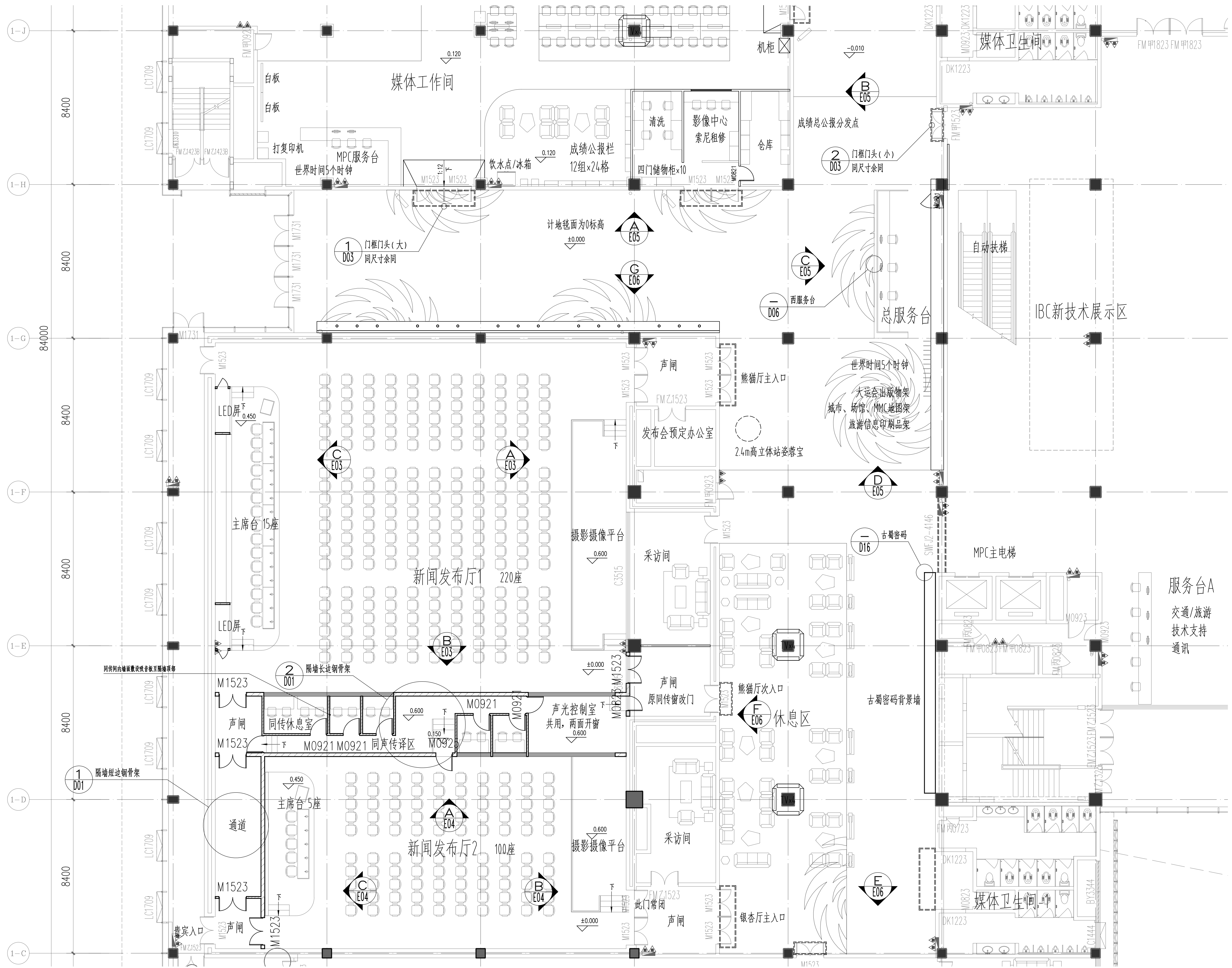
发布厅及其外侧公共通道放大平面图 1:100
