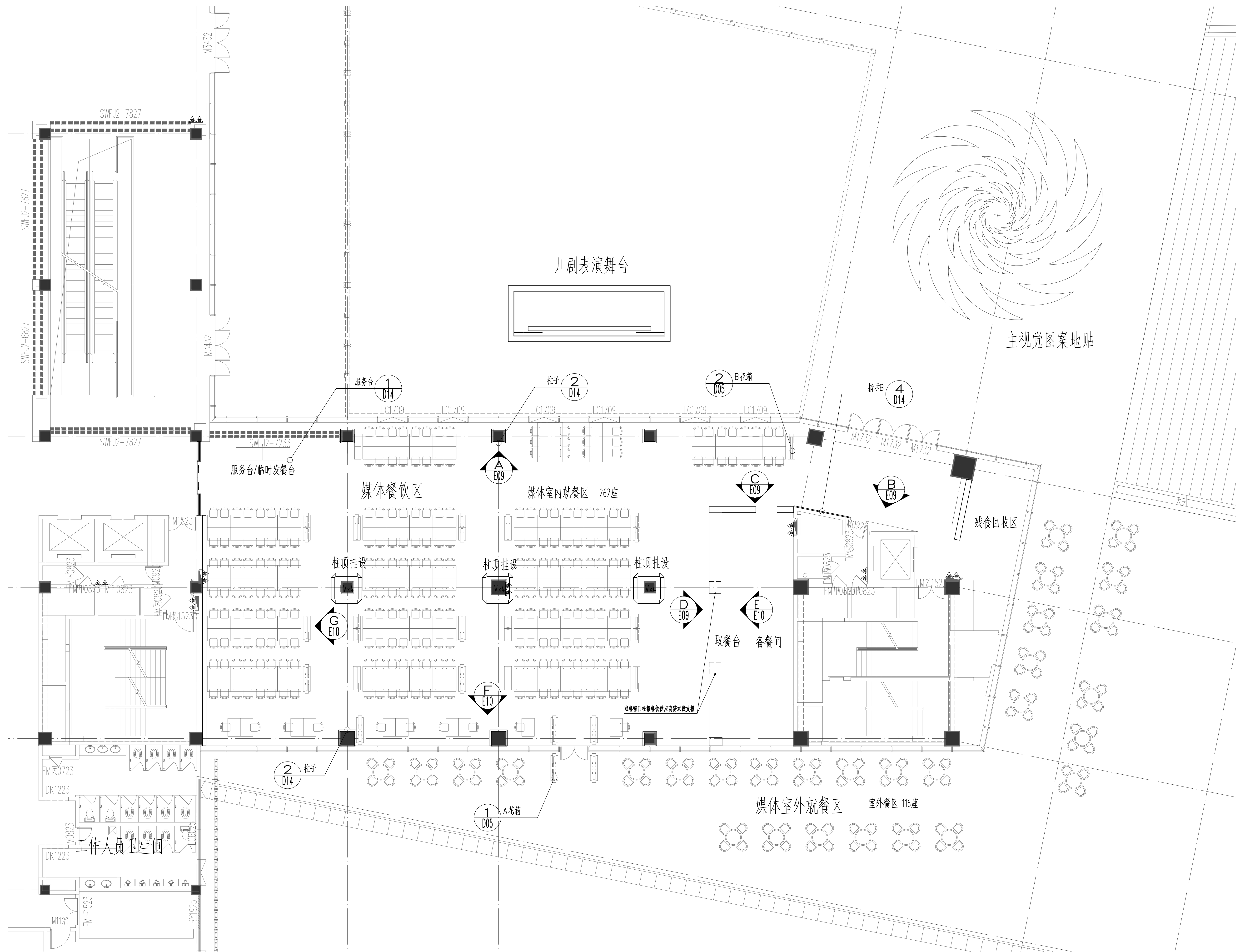
媒体餐厅放大平面图 1:100
