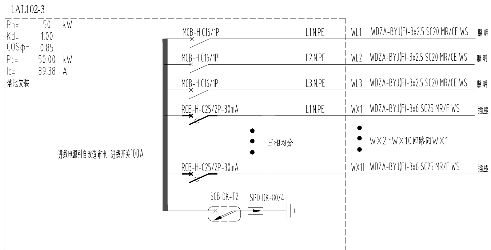
媒体工作普通用电配电箱
