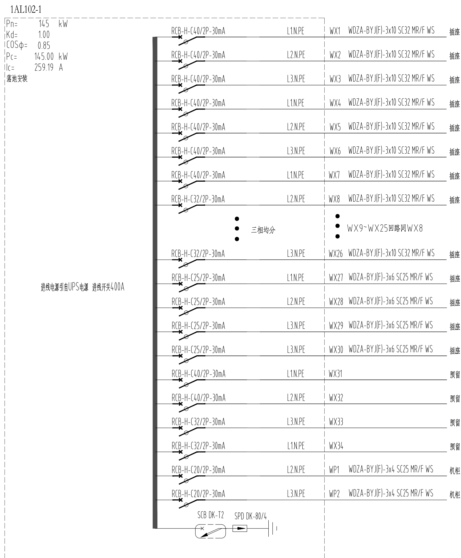
媒体工作间UPS电源动力插座用电配电箱
