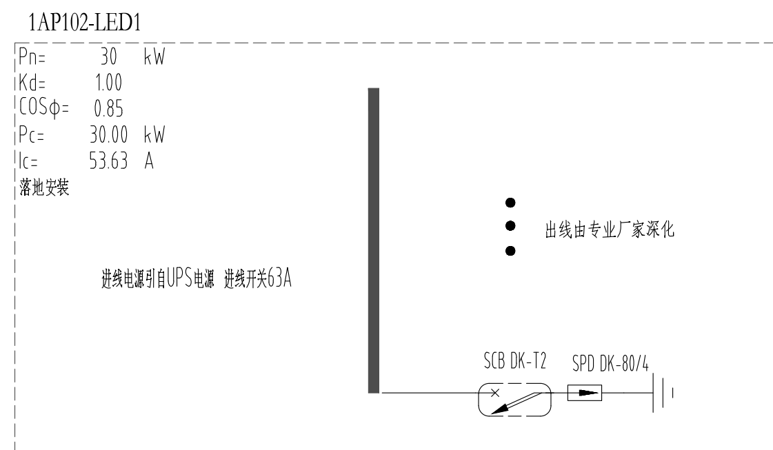
媒体工作间UPS电源LED配电箱1
