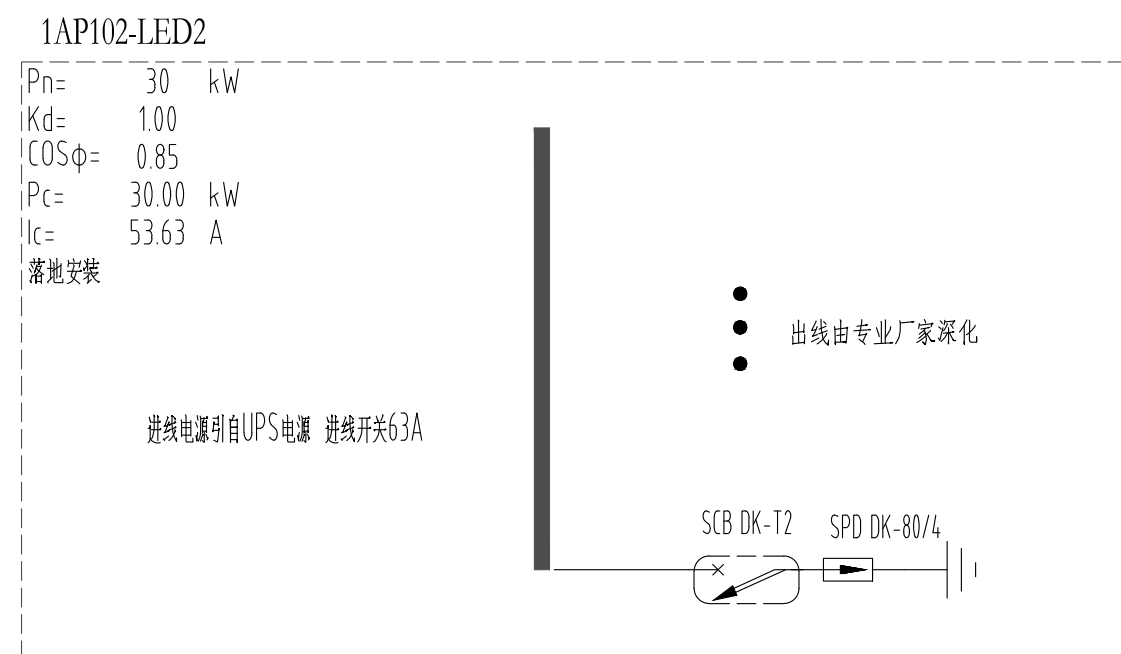
媒体工作间UPS电源LED配电箱2
