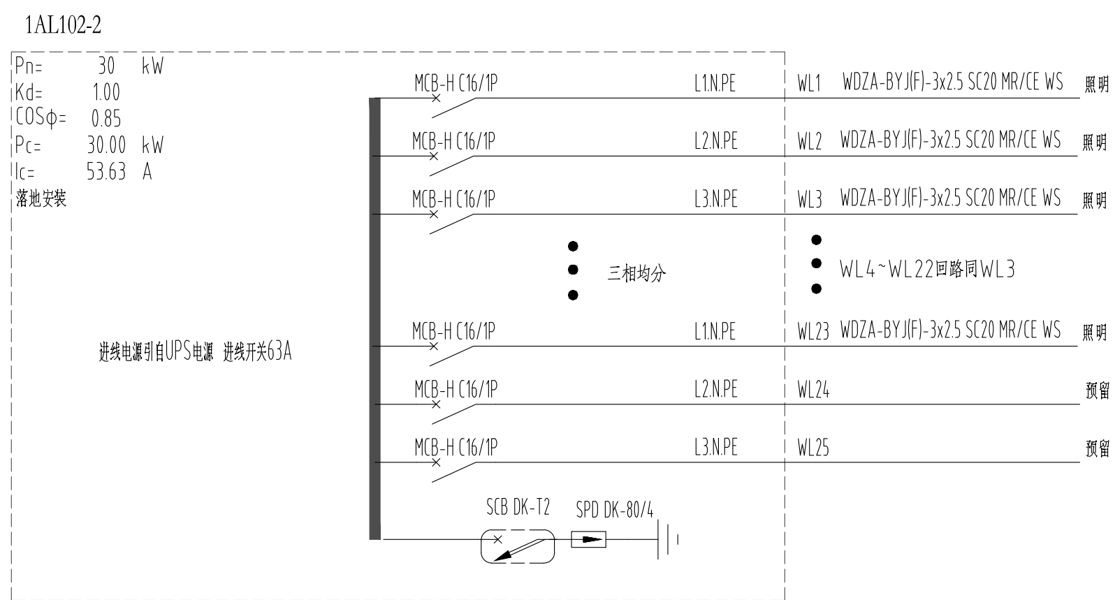
媒体工作间UPS电源照明用电配电箱
