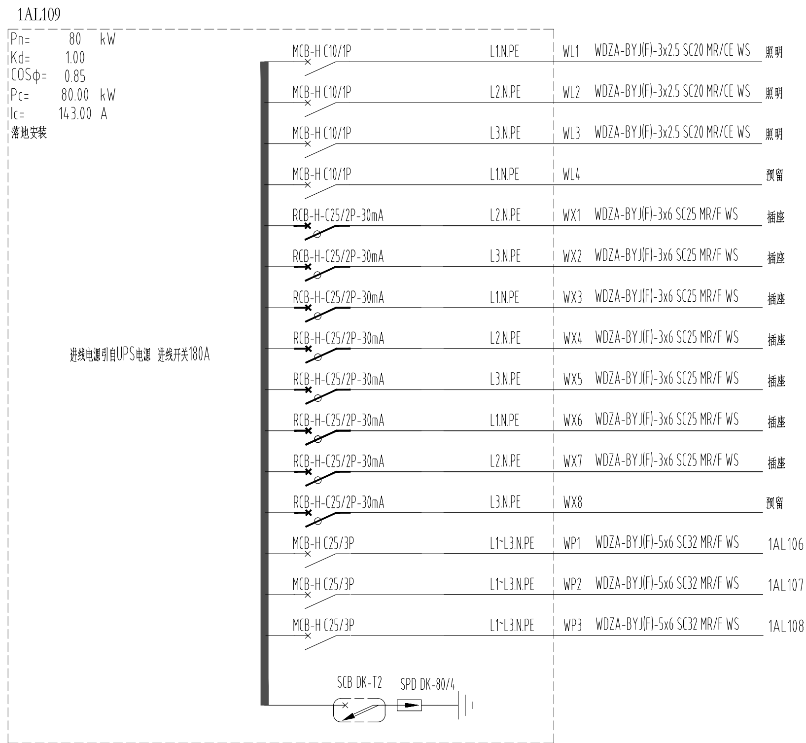
新闻发布厅UPS电源照明用电配电箱
