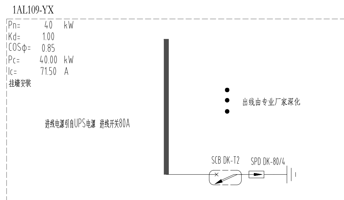
新闻发布厅UPS电源音响配电箱
