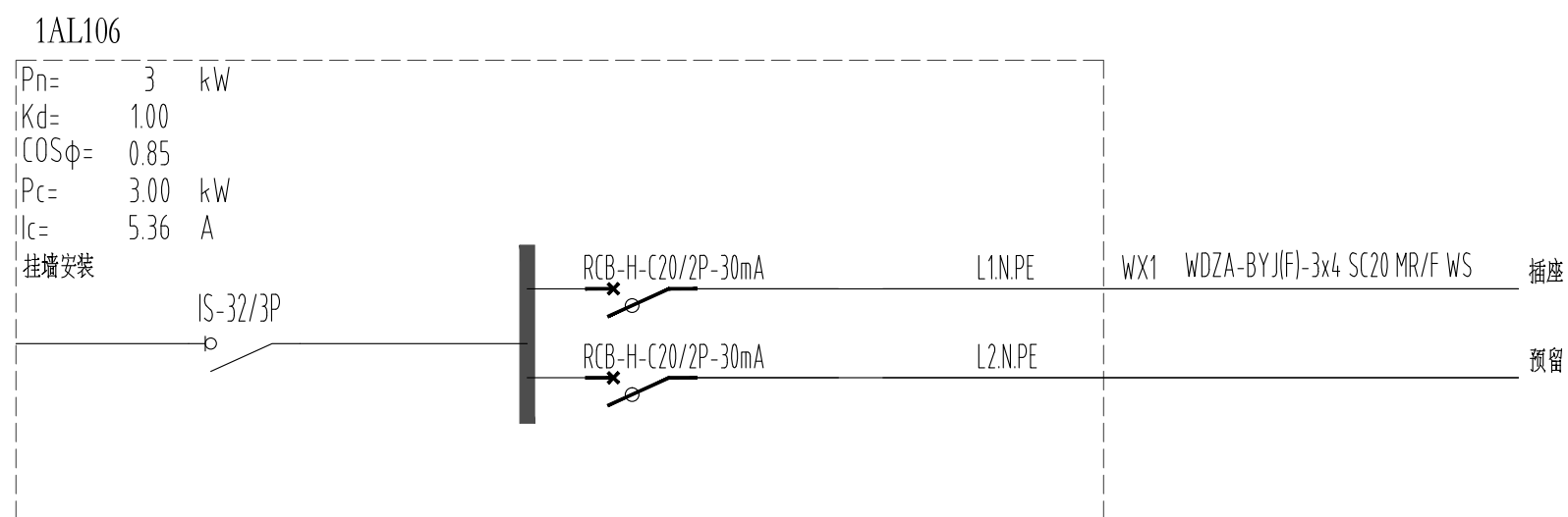
发布会预定办公室UPS电源插座用电配电箱
