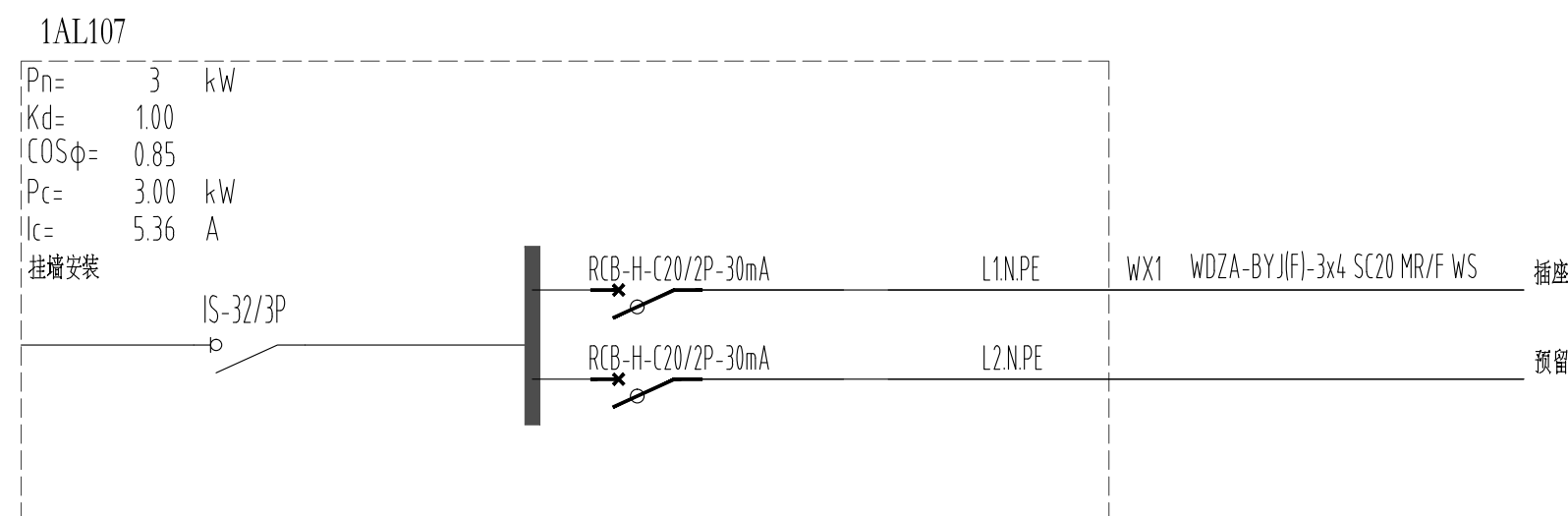
采访间UPS电源插座用电配电箱
