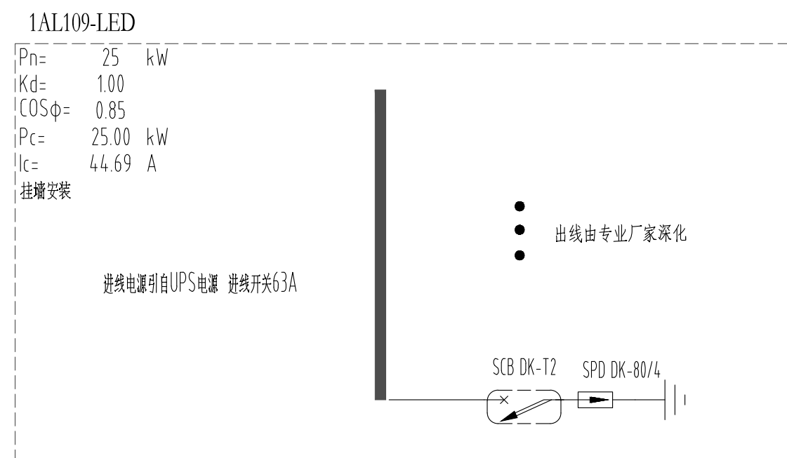
新闻发布厅UPS电源LED配电箱
