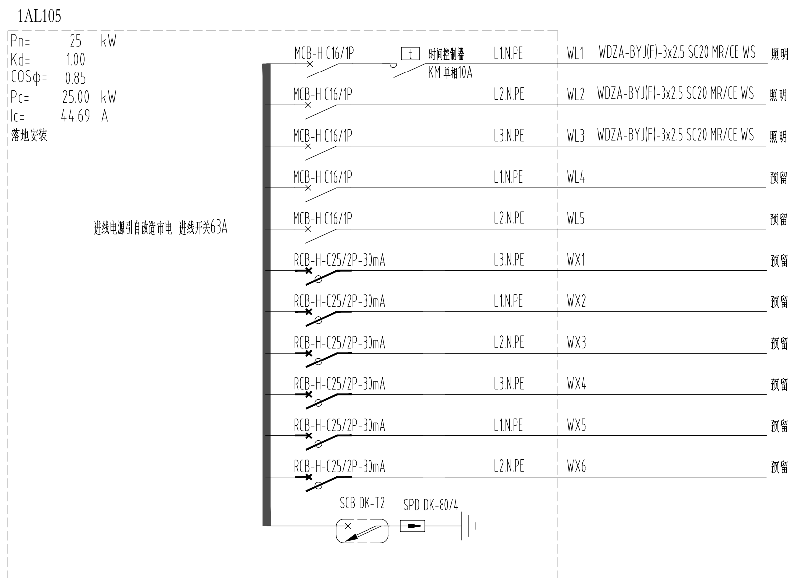
新闻发布厅外休息区用电配电箱
