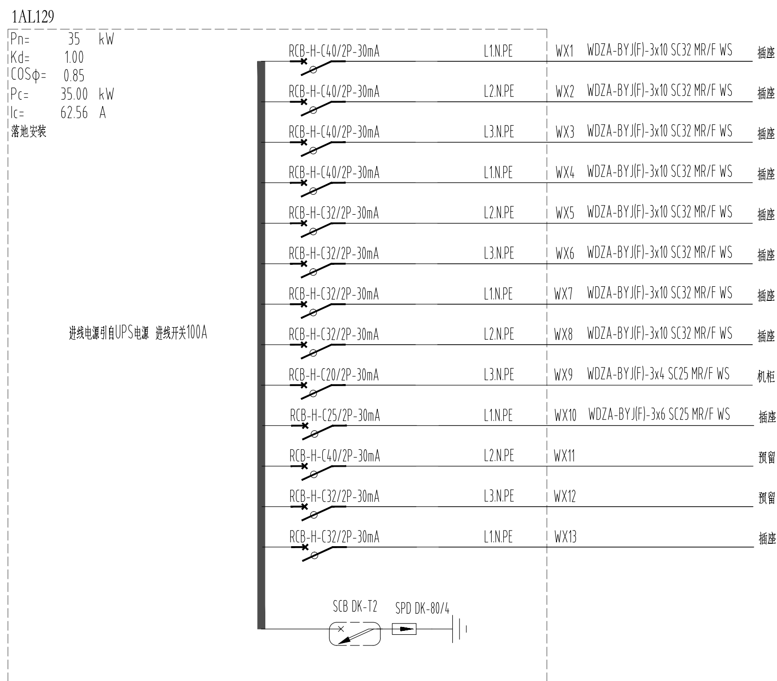
人民日报工作间UPS电源动力插座用电配电箱
