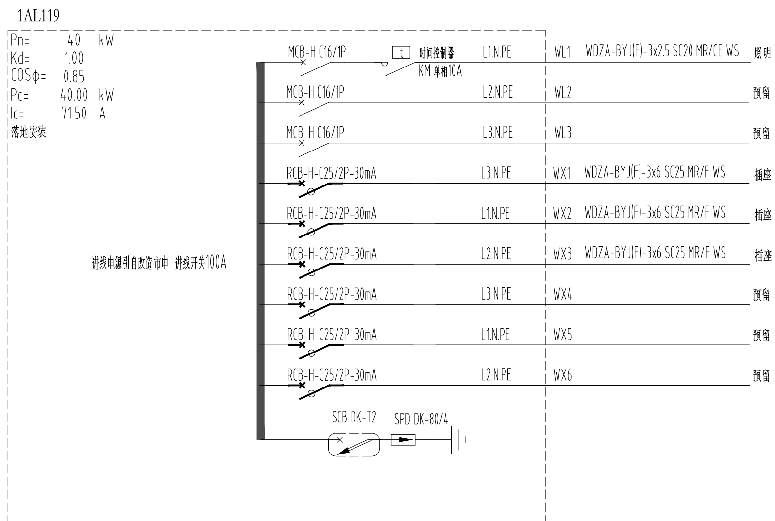
117-119南侧服务欢迎区用电配电箱
