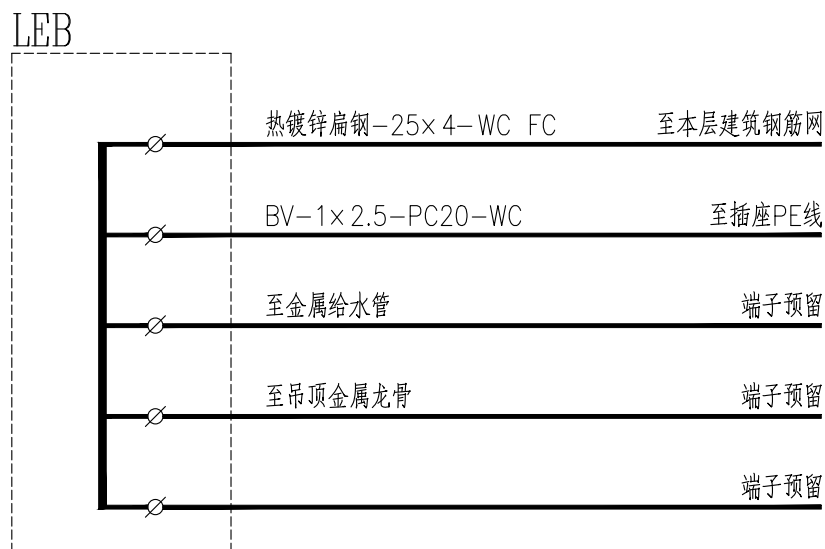
LEB箱大样图
