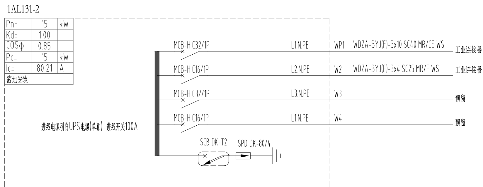
新华社UPS电源机房用电配电箱
