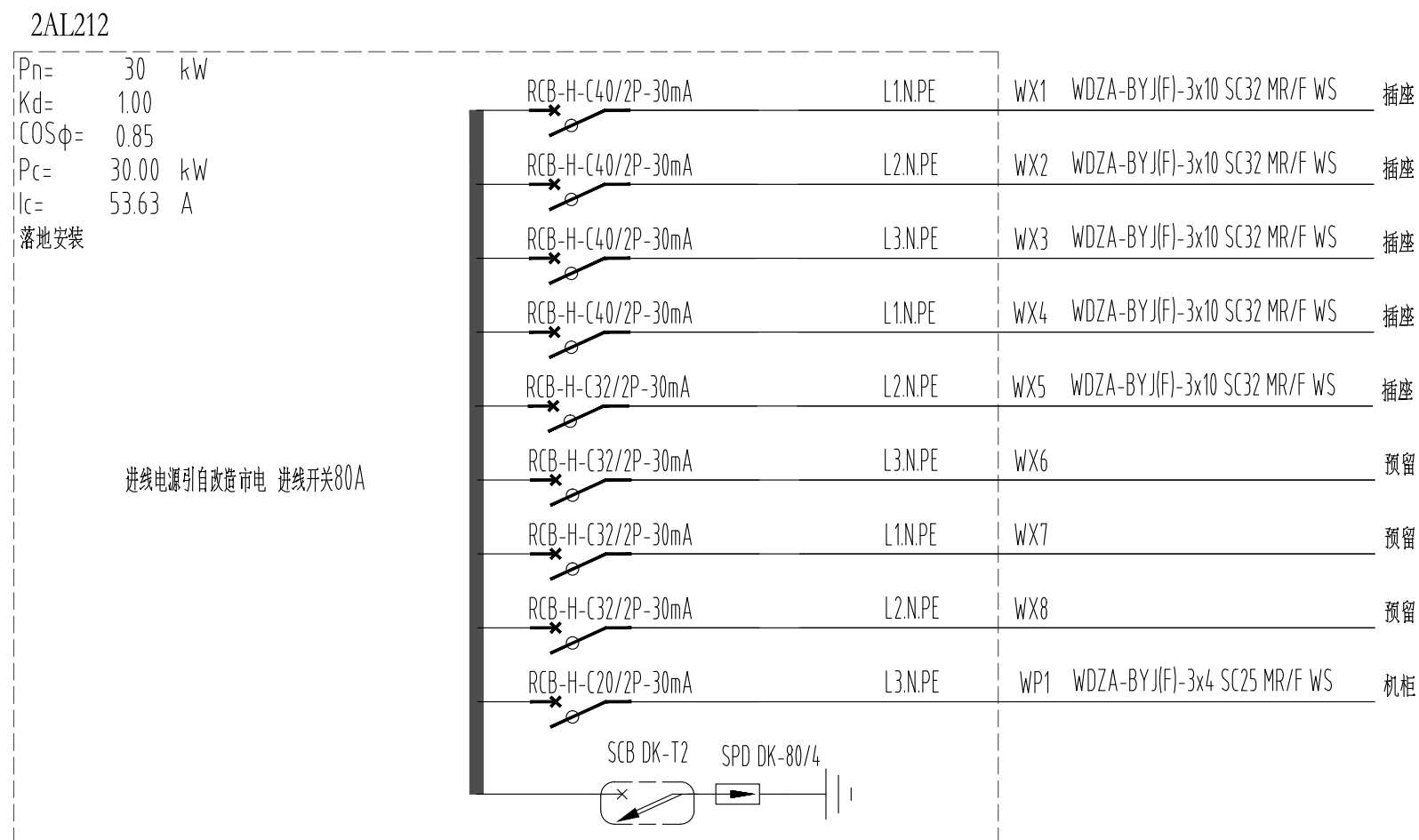
212-215区插座用电配电箱
