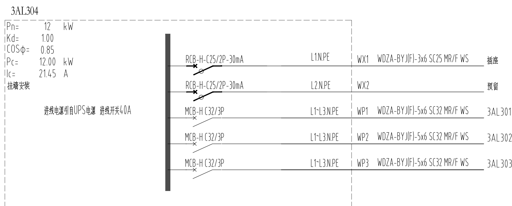
3层采访间UPS电源照明用电配电箱
