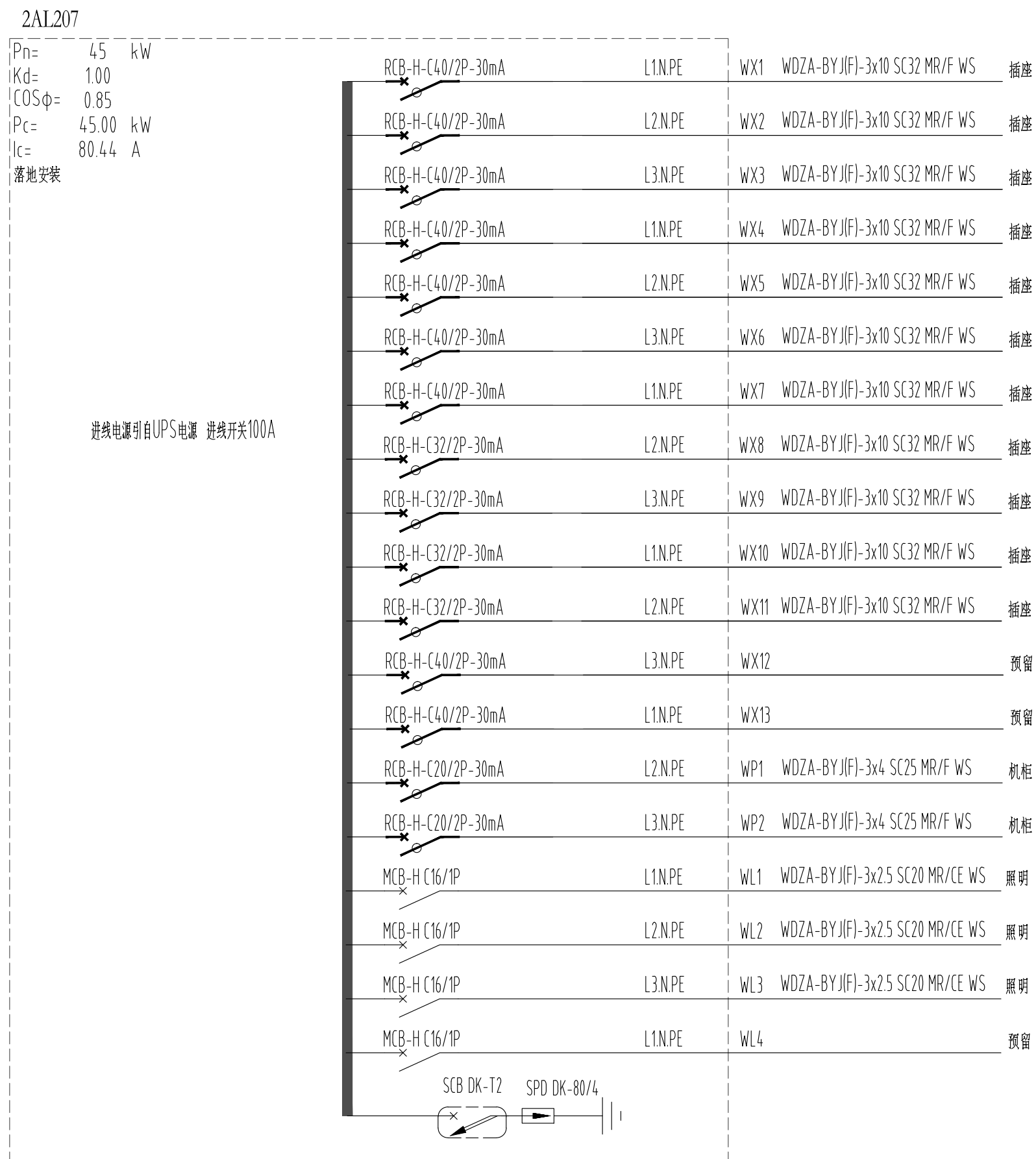
205-210办公区UPS电源动力插座用电配电箱
