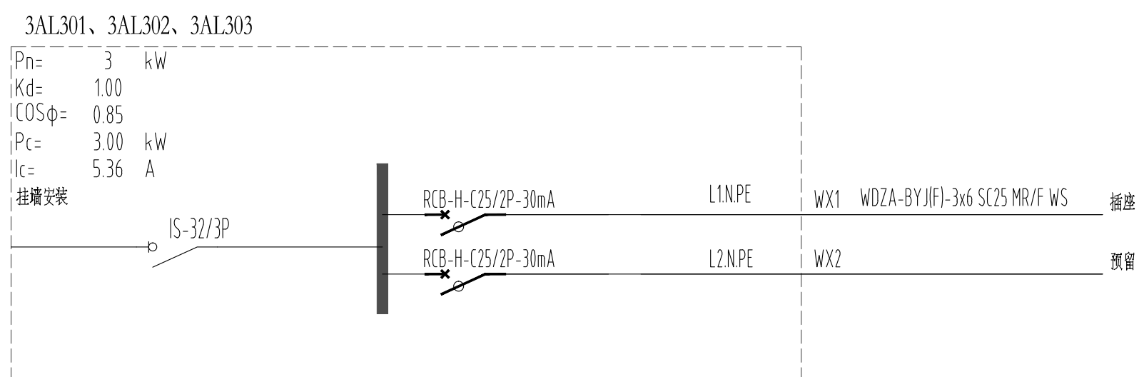
3层采访间UPS电源照明用电配电箱
