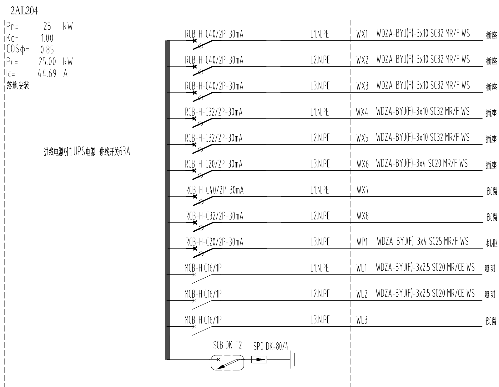
204 办公区UPS电源动力插座用电配电箱
