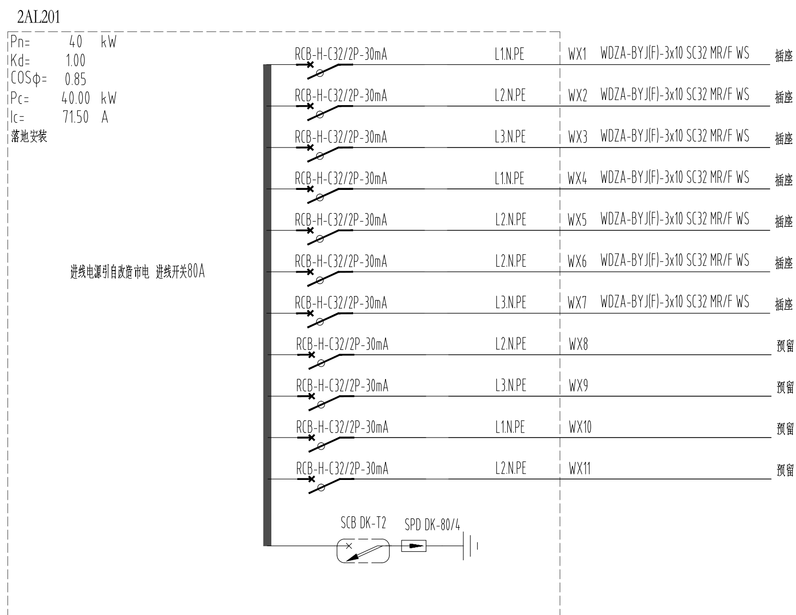
食堂区插座用电配电箱
