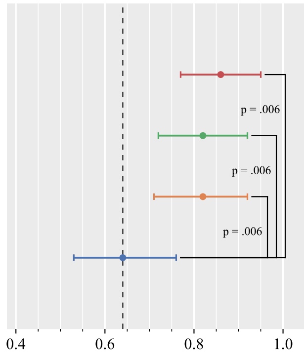
Llama-3.1-70B
