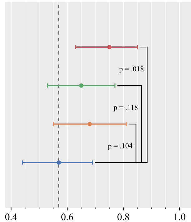
Llama-3.1-8B
