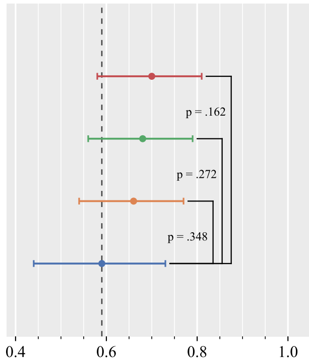
Qwen3-32B
