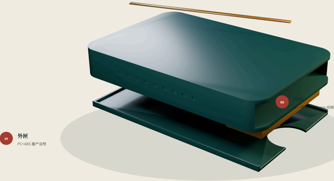
03 抬升片 POM 低摩擦楔形结构
