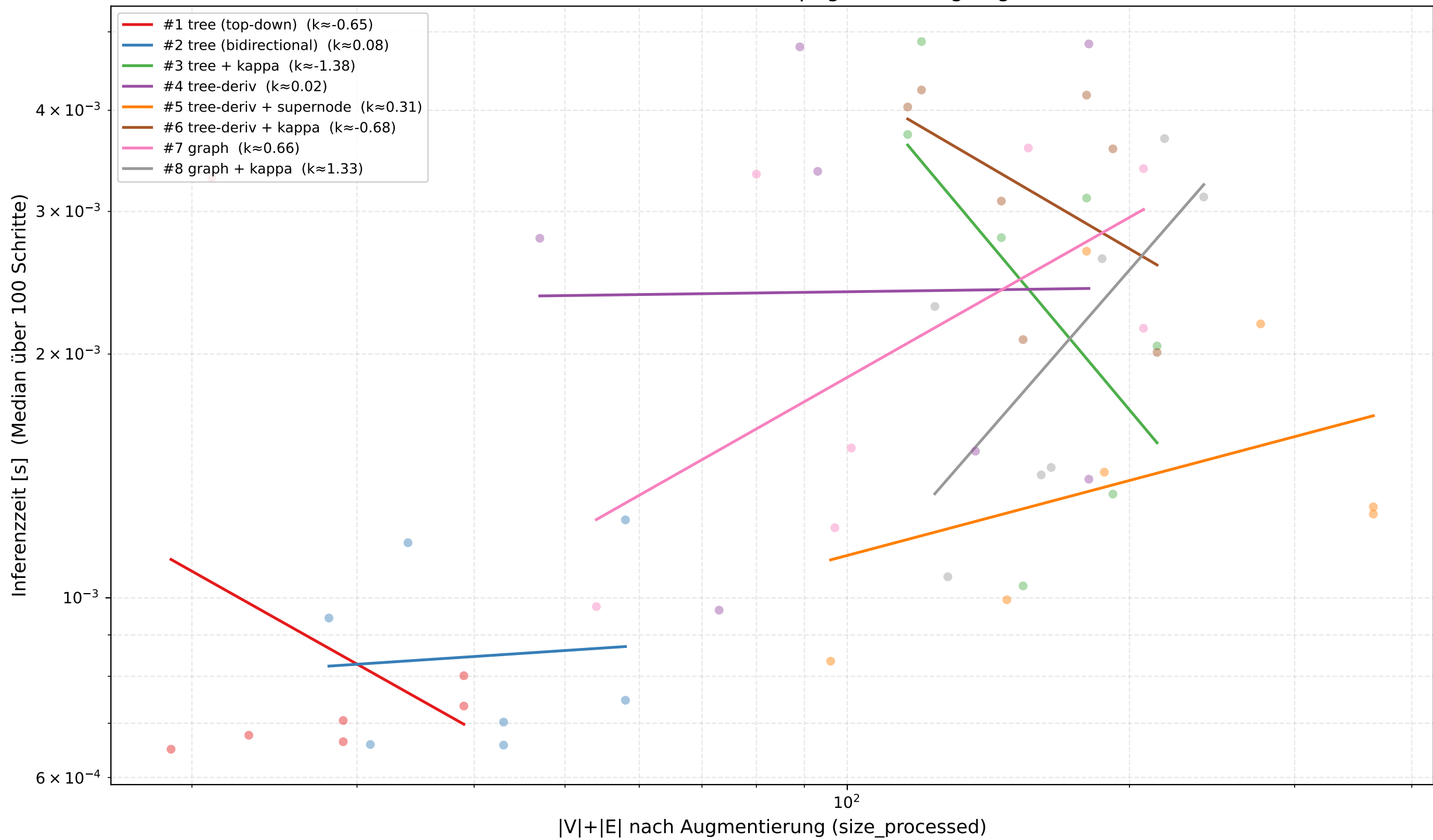
GINConv Inferenzzeit vs. Graphgröße — Log-Log-Plot
